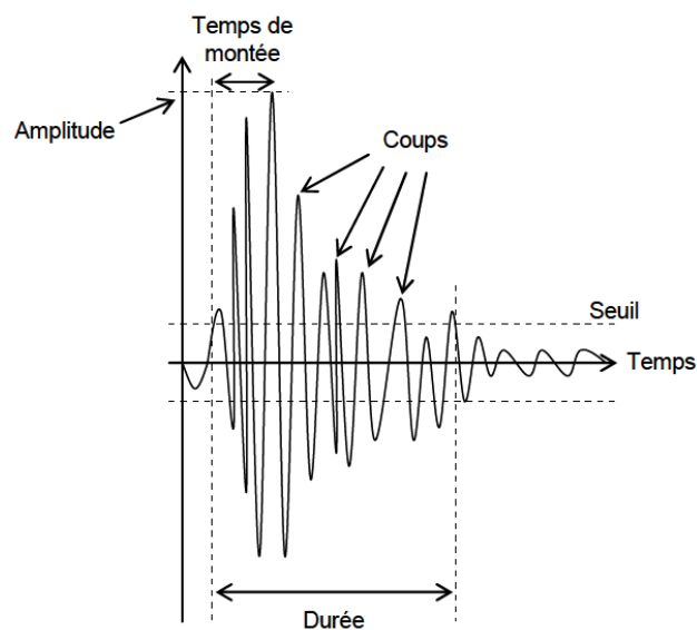
Figure 3-2 : Principaux paramètres d'une salve d'émission acoustique
