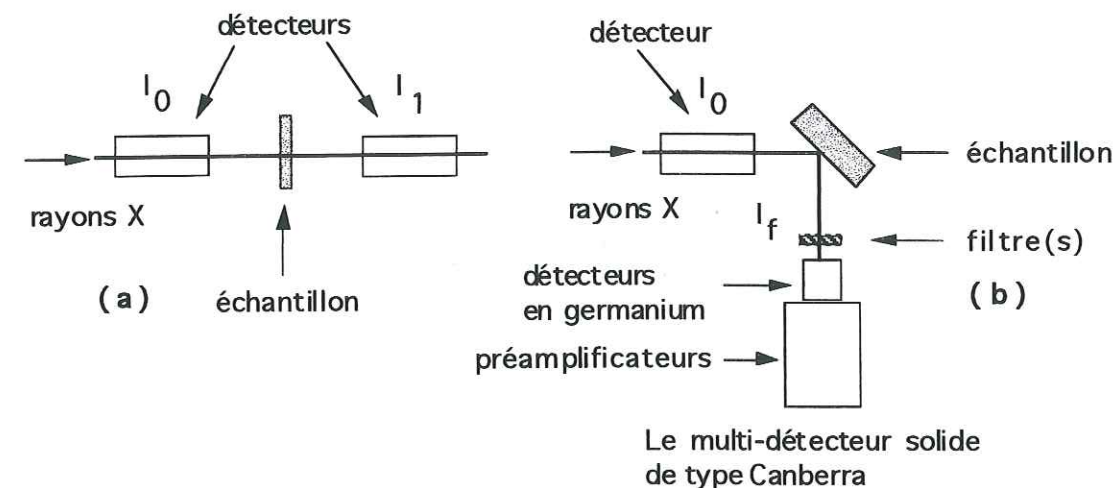
Figure A-4 : Les deux modes de mesure des spectres EXAFS en transmission (a) et en fluorescence (b) .
