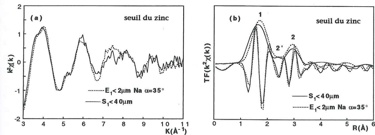
Figure 5-11 : Spectres EXAFS et FDR au seuil du zinc de la fraction inférieure à 40\mu m de Séclin et de la fraction argileuse d'Évin.
