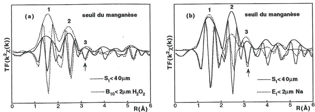
Figure 5-10 : Comparaison au seuil du manganèse des FDR des fractions fines de Maatheidée, d'Évin et de Séclin.
