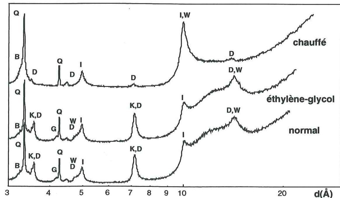
Figure 4-11 : Diffractogrammes d'argiles orientées de TN4<2 \mu m traité H 2 O 2 est échangé Ca. I=illite, K=kaolinite, D=chlorite, W=vermiculite, Q=quartz, B=albite, G=goethite (radiation Cu K \alpha ).
