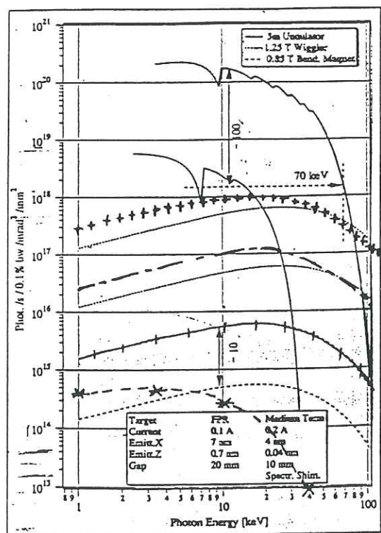
Figure A-2: Flux de photons en fonction de l'énergie sur la ligne CRG/IF. Mode focalisé (--) et non focalisé (-+-) ainsi que le flux de photons reçus sur l'échantillon, par seconde et par mm^2 (++++).
