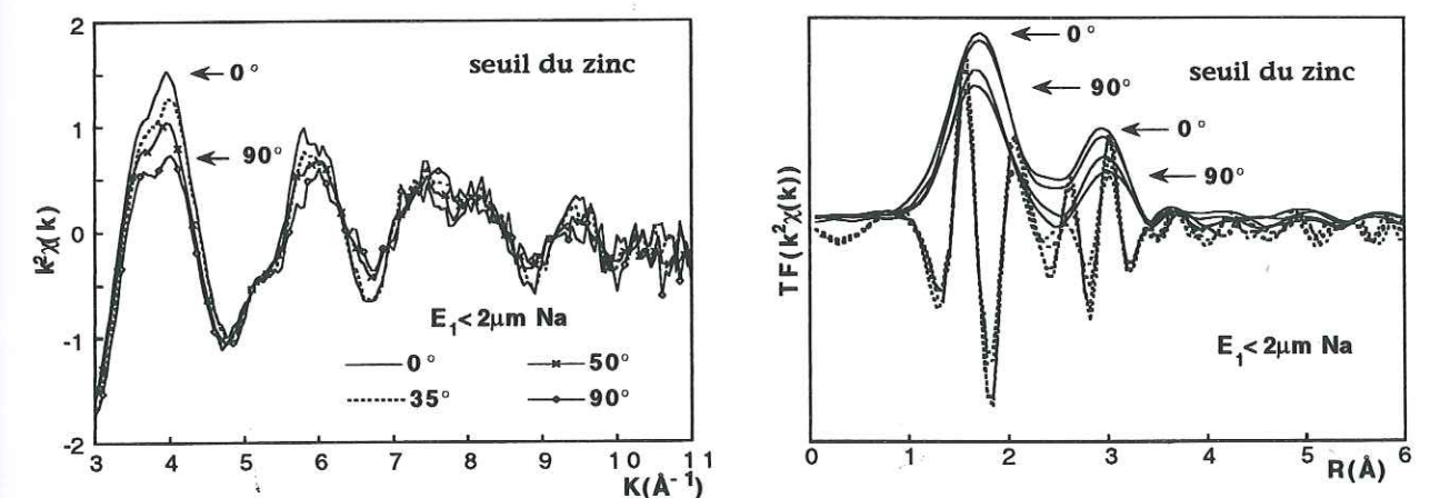
Figure 5-15 : Spectres EXAFS et FDR enregistrés en polarisation au seuil du zinc de la fraction argileuse d'Évin ( E_1 ).
