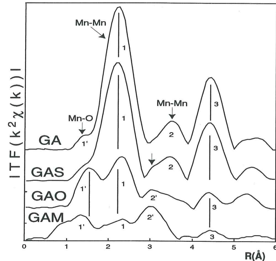
Figure 3-15 : FDR au seuil du manganèse des quatre grenailles d'acier
