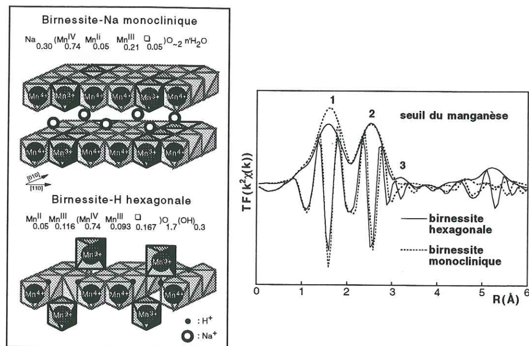
Figure 2-19 : Représentation structurale et FDR au seuil du manganèse de la birnessite hexagonale (pH=4) et de la birnessite monoclinique (pH=9) (d'après Silvester et al., 1997).
