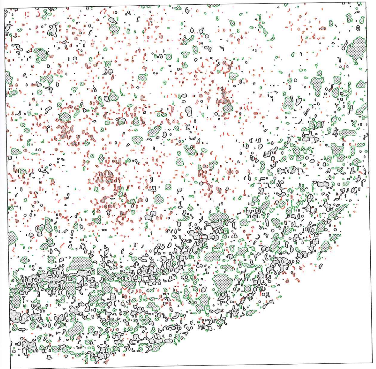
Figure 4-4 : Carte de répartition du plomb, de l'aluminium et du silicium dans le grain n°1 de TN4. Pb>120 : traits rouges + hachures grises Al>80 : traits noirs + hachures gris-clair Si>100 : traits verts + hachures gris-clair échelle 1 cm = 38 microns
