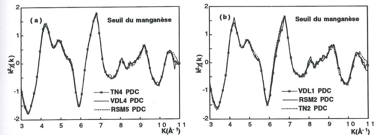
Figure 4-12 : Comparaison au seuil du manganèse entre les spectres EXAFS des six échantillons de plombs de chasse.
