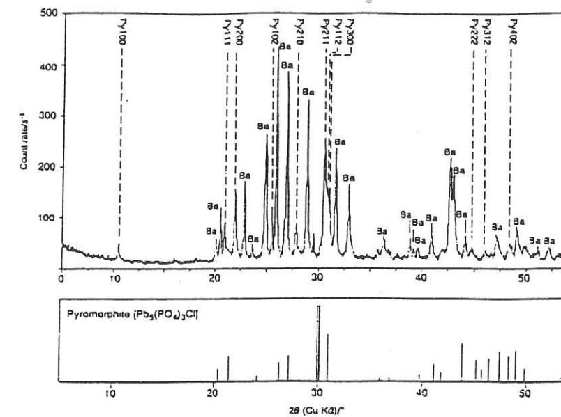
Figure 2-26 : Diffractogramme X de la fraction dense d'un sol pollué par des déchets miniers. La baryte (BaSO 4 ) et la pyromorphite non "pure" (notée Py) sont identifiées. Les raies de diffraction d'une pyromorphite de référence sont indiquées (fiche JCPDS n°19-701) (d'après Cotter-Howells et al., 1994).
