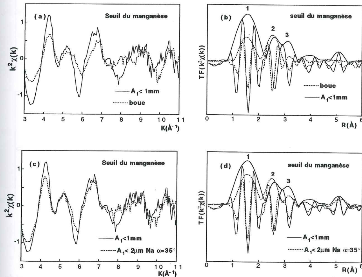
Figure 3-12 : Spectres EXAFS et FDR au seuil du manganèse de la boue, du sol A_1 et de la fraction argileuse échangée Na.
