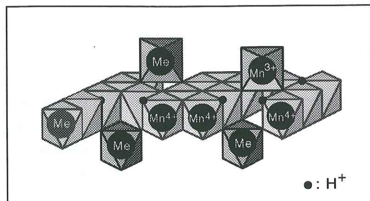
Figure 2-21 : Représentation structurale des métaux (Me) adsorbés sur la birnessite.
