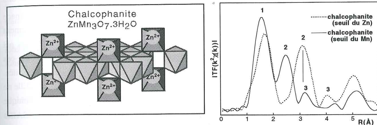
Figure 2-18 : Représentation structurale de la chalcophanite (d'après Wadsley, 1955 ; Post et Appleman, 1988) et FDR au seuil du manganèse et du zinc de la chalcophanite.
