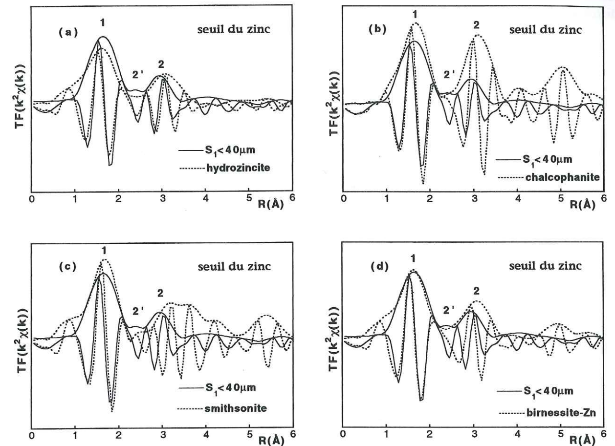
Figure 5-14 : FDR au seuil du zinc de la fraction inférieure à 40 \mu\text{m} de Séclin et de l'hydrozincite (a) , de la chalcophanite (b) , de la smithsonite (c) , et de la birnessite-Zn (d) .
