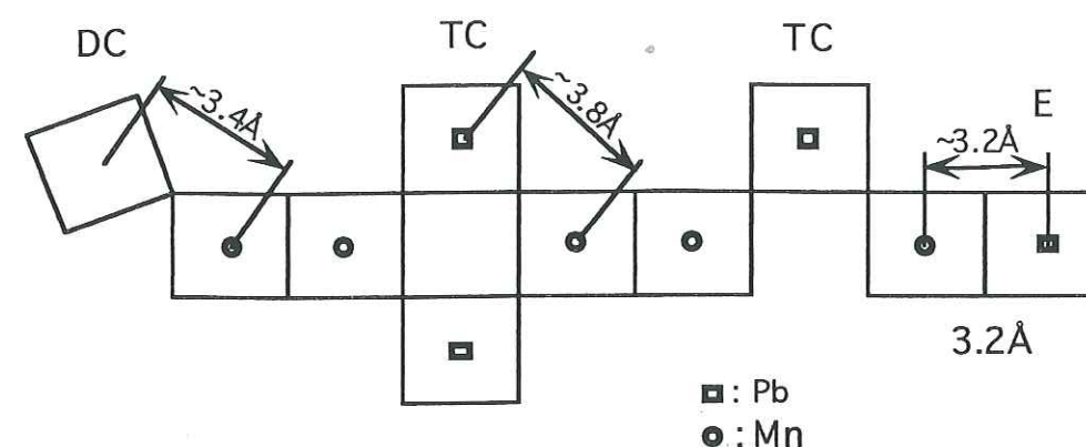
Figure 4-25 : Représentation structurale du plomb adsorbé sur la birnessite hexagonale. Liaisons par arêtes (E), par sommets doubles (DC) ou triples (TC).
