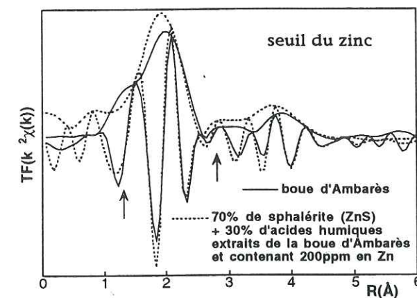
Figure 3-19 : FDR de la boue d'Ambarès et d'une combinaison linéaire de 30% d'acide humique provenant de la boue d'Ambarès à 200 mg/kg de zinc et de 70% de sphalérite.
