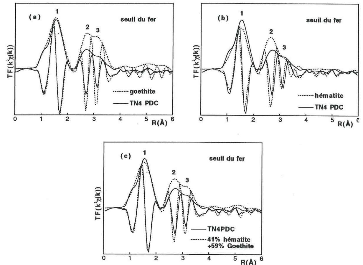
Figure 4-17 : FDR au seuil du fer des nodules de TN4, de la goéthite (a) , de l'hématite (b) et d'une combinaison linéaire de 41% d'hématite et de 59% de goéthite (c) .
