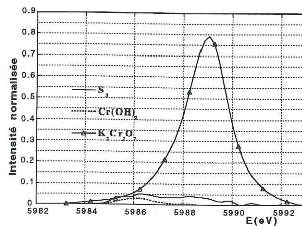
Figure 6-1 : Prépics au seuil du chrome du sol S 3 brut et de K 2 Cr 2 O 7 et de Cr(OH) 3 (d'après Manceau et Hargé, 1996).
