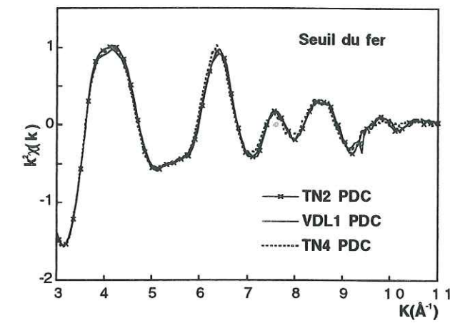
Figure 4-16 : Spectres EXAFS au seuil du fer des échantillons de nodules TN2, VDL1 et TN4.
