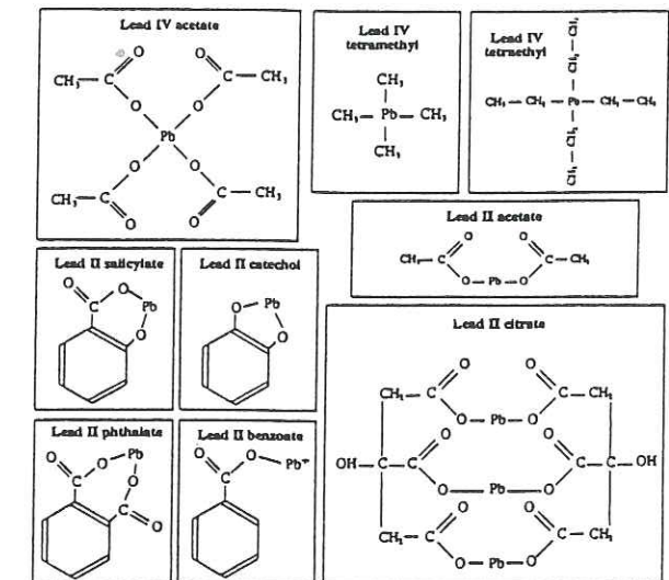
Figure 2-32 : Formules chimiques développées de composés de coordination du plomb et de composés organo-plombiques (d'après Manceau et al., 1996).
