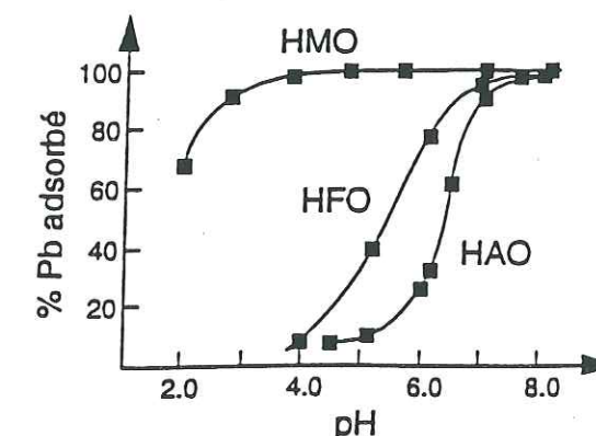
Figure 3-3 : Isothermes d'adsorption du plomb sur HMO, sur HFO et sur HAO (d'après Gadde, 1974).
