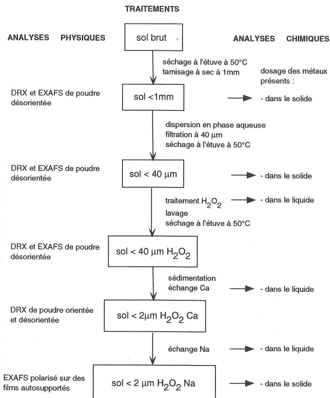
Figure 1-6 : Traitements et analyses chimiques et physiques des sols contaminés par des métaux lourds.
