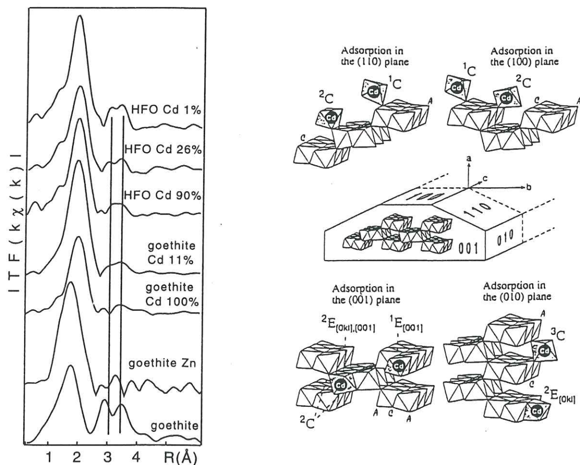
Figure 2-12 : FDR au seuil de l'élément fixé, de Cd (1) ou de Zn (2) adsorbé sur la goéthite et de Cd (1) adsorbé sur HFO à différents taux de recouvrement. La FDR de la goéthite au seuil du fer ainsi qu'une représentation structurale des sites d'adsorption du cadmium sur la goéthite (1) sont également données (d'après: (1) Spadini et al., 1994 ; (2) Schlegel et al., 1997).
