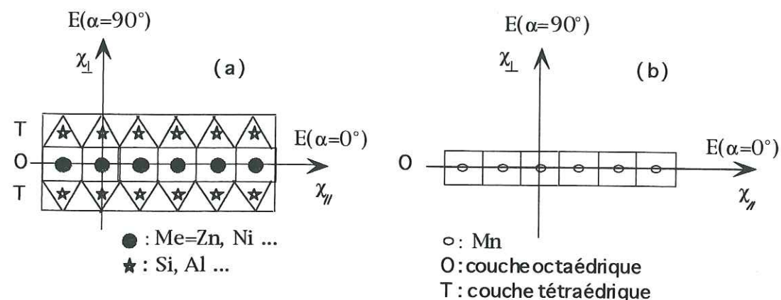
Figure B-1: Représentation structurale schématique d'une argile TOT (a) et d'un phyllo-manganate.
