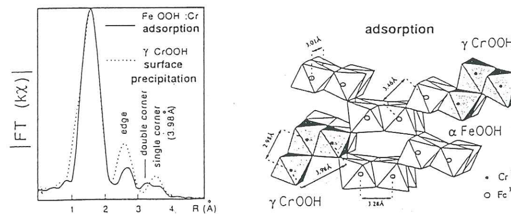
Figure 2-14: Module de la FDR au seuil de Cr, du chrome adsorbé sur la goéthite (trait plein) et du précipité de surface \gamma\text{CrOOH} (pointillés) et représentation structurale de Cr adsorbé sur la goéthite (d'après Charlet et Manceau, 1992).
