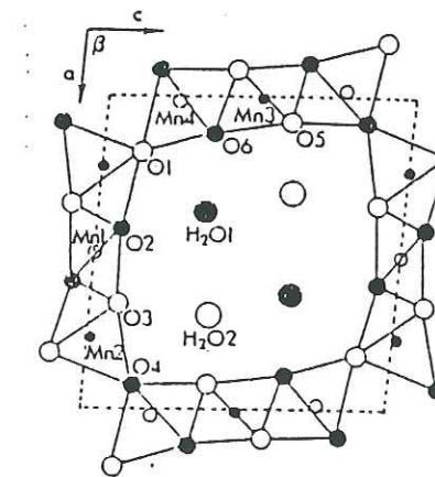
Figure 2-25 : Représentation structurale de la todorokite dans le plan (a,c). Indexation des quatre sites cationiques (M 1 , M 2 , M 3 et M 4 ) occupés par des Mn 4+ et par d'autres cations (d'après Post et Bish, 1988).
