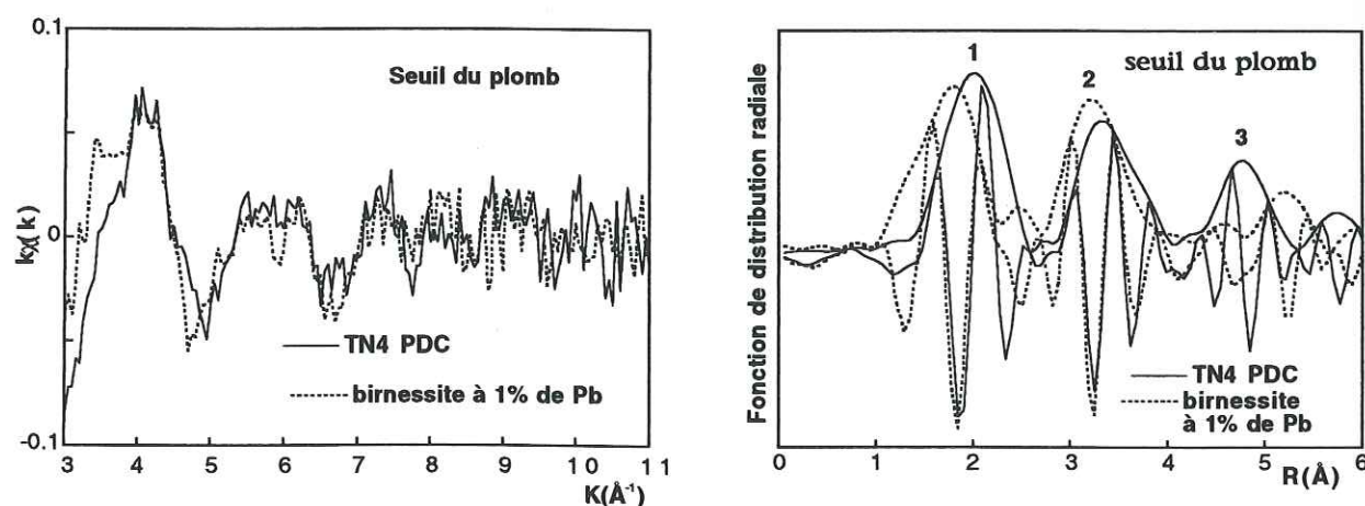
Figure 4-24 : Spectre EXAFS et FDR au seuil du plomb d'un échantillon de nodules TN4 et de la birnessite contenant 1% massique de plomb.
