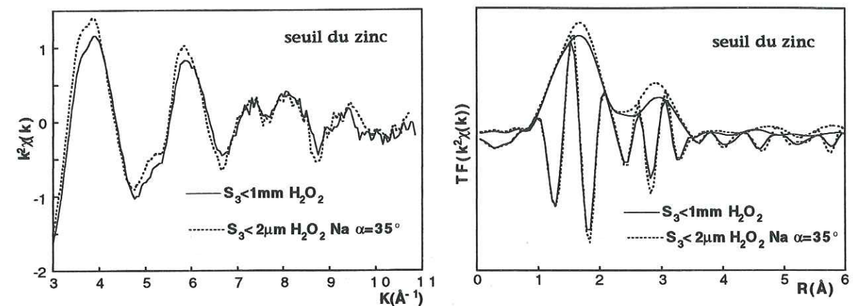
Figure 6-7 : Spectres EXAFS et FDR au seuil du zinc de la fraction inférieure à 1mm traitée \text{H}_2\text{O}_2 et inférieure à 2 \mu\text{m} traitée \text{H}_2\text{O}_2 et échangée Na.
