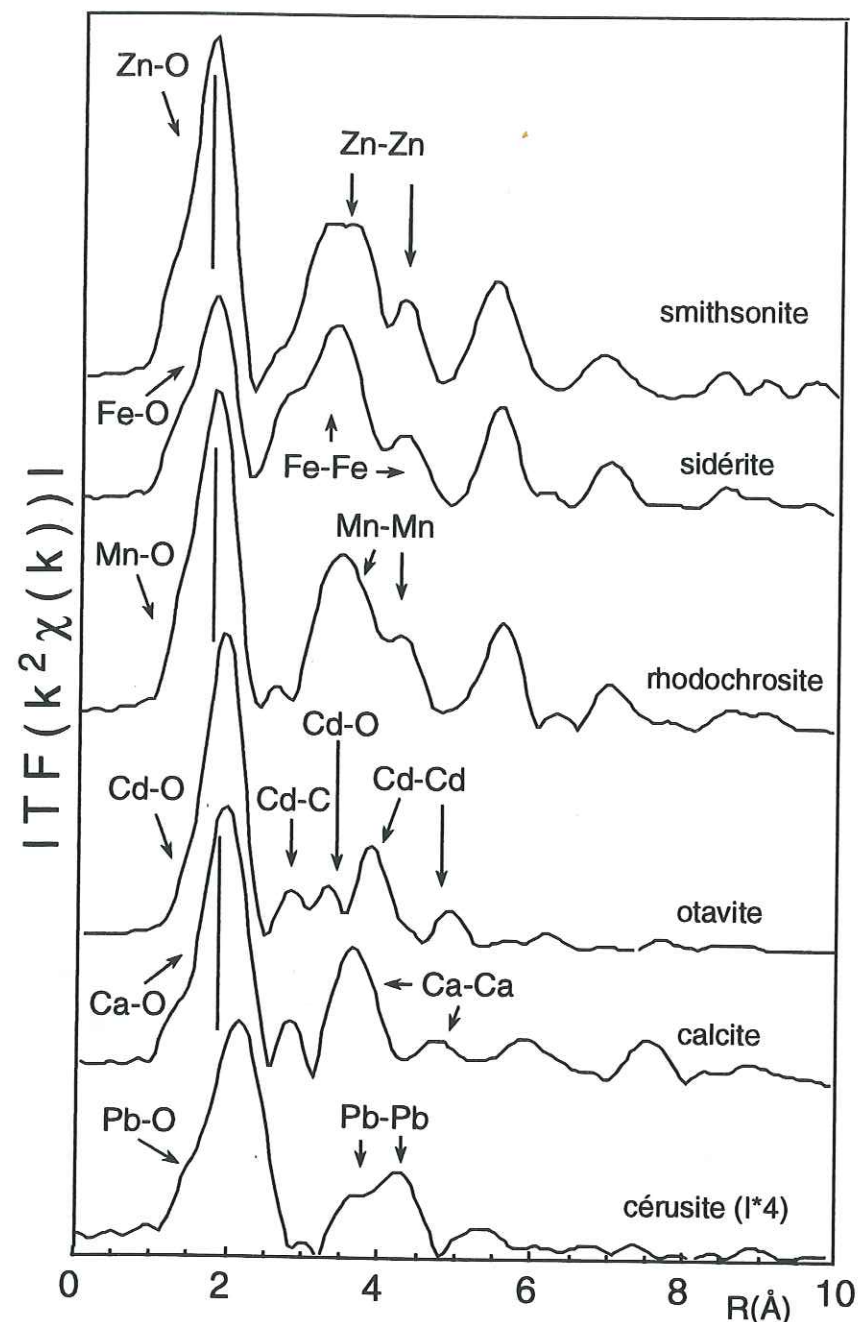
Figure 1-5 : Fonctions de distribution radiale aux seuils : du zinc (smithsonite : ZnCO_3 ), du manganèse (rhodochrosite : MnCO_3 ), du fer (sidérite : FeCO_3 ), du calcium ( CaCO_3 ) et du plomb (cérusite : PbCO_3 : l'intensité I est multipliée par 4). Les spectres EXAFS ont été enregistrés à température ambiante.
