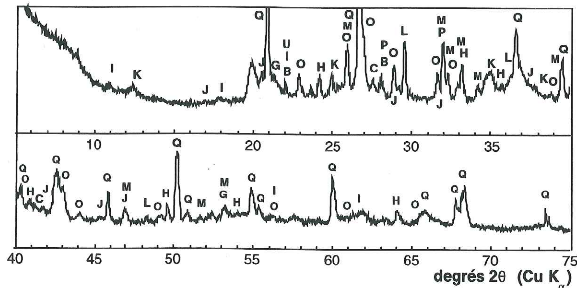
Figure 4-9 : Diffractogramme X des plombs de chasse de TN4. I=illite, K=kaolinite, J=calcite monohydrate, U=cristobalite, G=goethite, B=albite, O=barytine, H=hématite, Q=quartz, P=phosphate de baryum, L=calcite, C=microcline, M=fluoroapatite.
