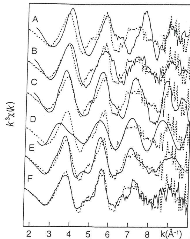
Figure 2-27 : Spectres EXAFS au seuil de Cd d'un échantillon naturel d'apatite (en pointillés) et comparaison avec la goethite-Cd (a) (d'après Spadini et al., 1994), Cd adsorbé sur la goethite (b) (11% de couverture) (d'après Spadini et al., 1994), l'otavite ( \text{CdCO}_3 ) (c) , la crandallite-Cd (d) (spectre théorique) et deux apatites synthétiques (e,f) (d'après Séry et al., 1996).
