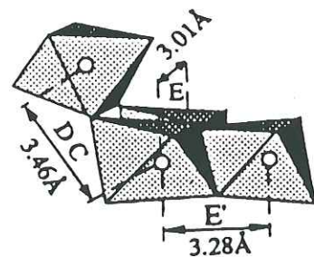
Figure 1-4 : Approche polyédrale de la structure de la goethite ( \alpha FeOOH) et de la ferrihydrate (d'après Manceau et Drits, 1993).
