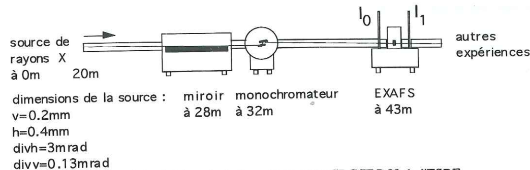
Figure A-3: Schéma de la ligne de lumière CRG/IF D32 de l'ESRF.
