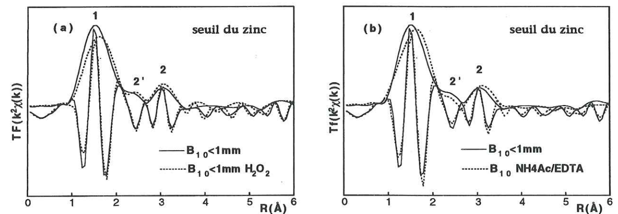
Figure 5-22 : FDR au seuil du zinc de B 10 brut, traité par H 2 O 2 ou par le mélange NH 4 Ac/EDTA.
