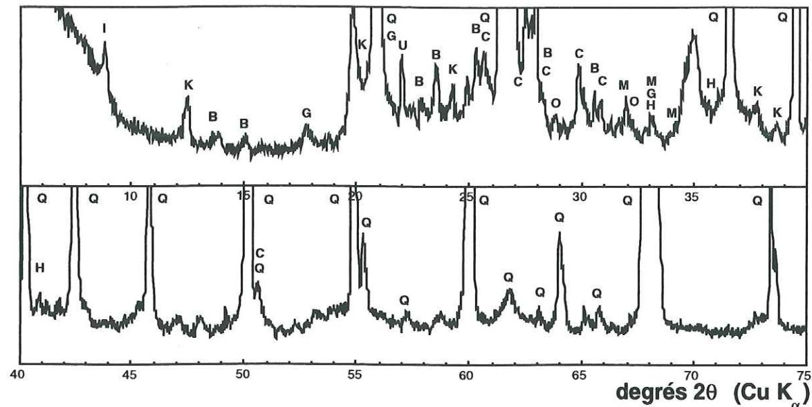
Figure 4-10 : Diffractogramme X de la fraction inférieure à 40 \mu m de TN4. I=illite, K=kaolinite, G=goethite, B=albite, O=barytine, C=microcline, H=hématite, Q=quartz, U=cristobalite, M=fluoroapatite.
