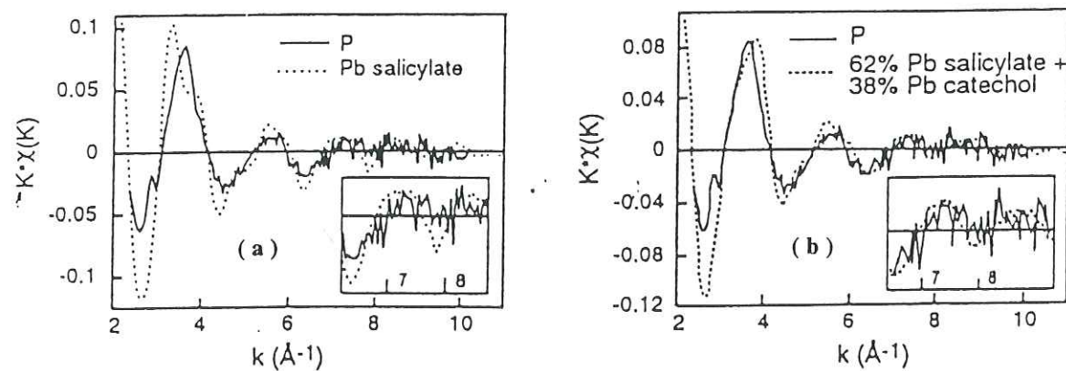
Figure 2-34 : Comparaisons entre les spectres EXAFS de l'échantillon de sol (P), du salicylate de plomb (a) et d'une combinaison salicylate et catéchol Pb (b) (d'après Manceau et al., 1996).
