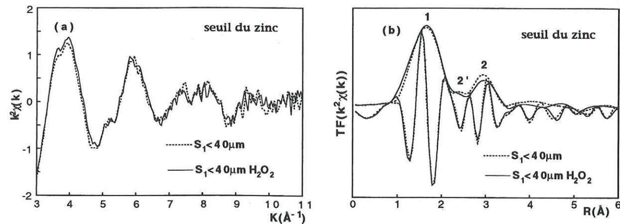
Figure 5-13 : Spectres EXAFS et FDR au seuil du zinc des fractions argileuse et inférieure à 50 \mu\text{m} de Séclin.
