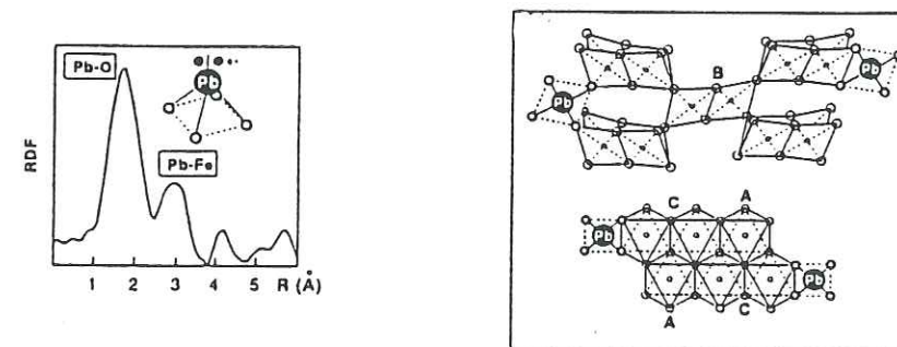
Figure 2-13 : FDR et représentation structurale de Pb 2+ adsorbé sur la ferrihydrite (d'après Manceau et al., 1992a).
