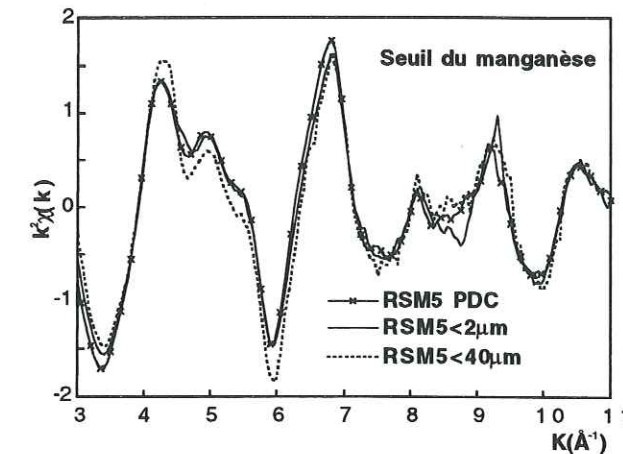
Figure 4-14 : Comparaison au seuil du manganèse des spectres EXAFS des échantillons de plombs de chasse, de la fraction inférieure à 40µm et de fraction argileuse provenant de RSM5.
