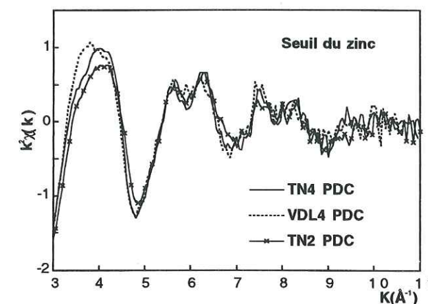
Figure 4-19 : Spectre EXAFS au seuil du zinc de trois échantillons de plombs de chasse (TN4, TN2 et VDL4).
