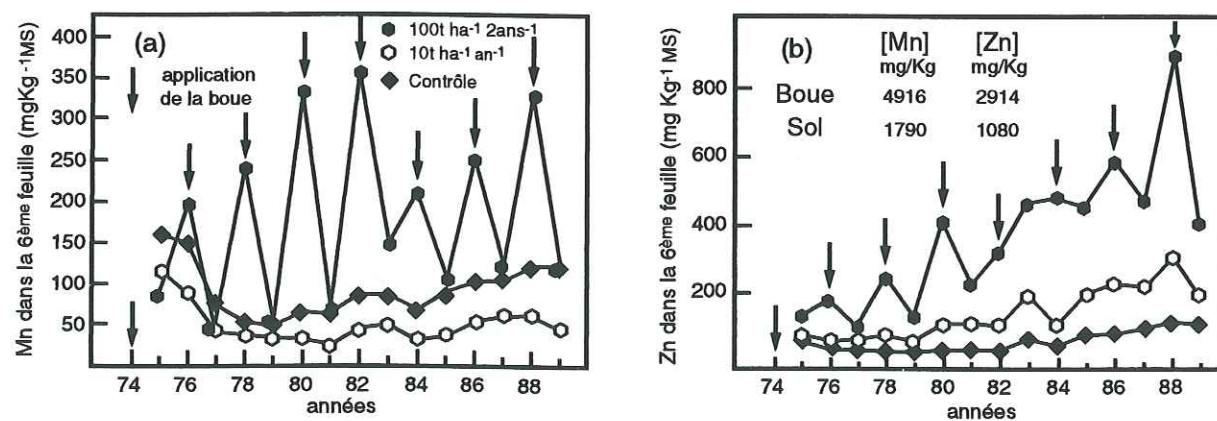
Figure 3-2 : Concentration en manganèse (a) et en zinc (b) présents dans la 6 ème feuille de maïs cultivé sur le sol amendé par la boue d'Ambarès (d'après Mench et al, 1992 ; Juste et Mench, 1992).
