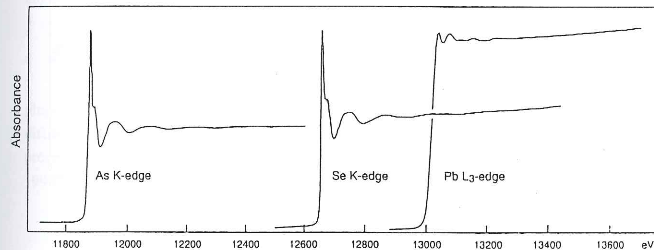
Figure 1-2 : Emplacement des seuils d'absorption X de l'arsenic, du sélénium et du plomb (d'après Manceau et al, 1997).
