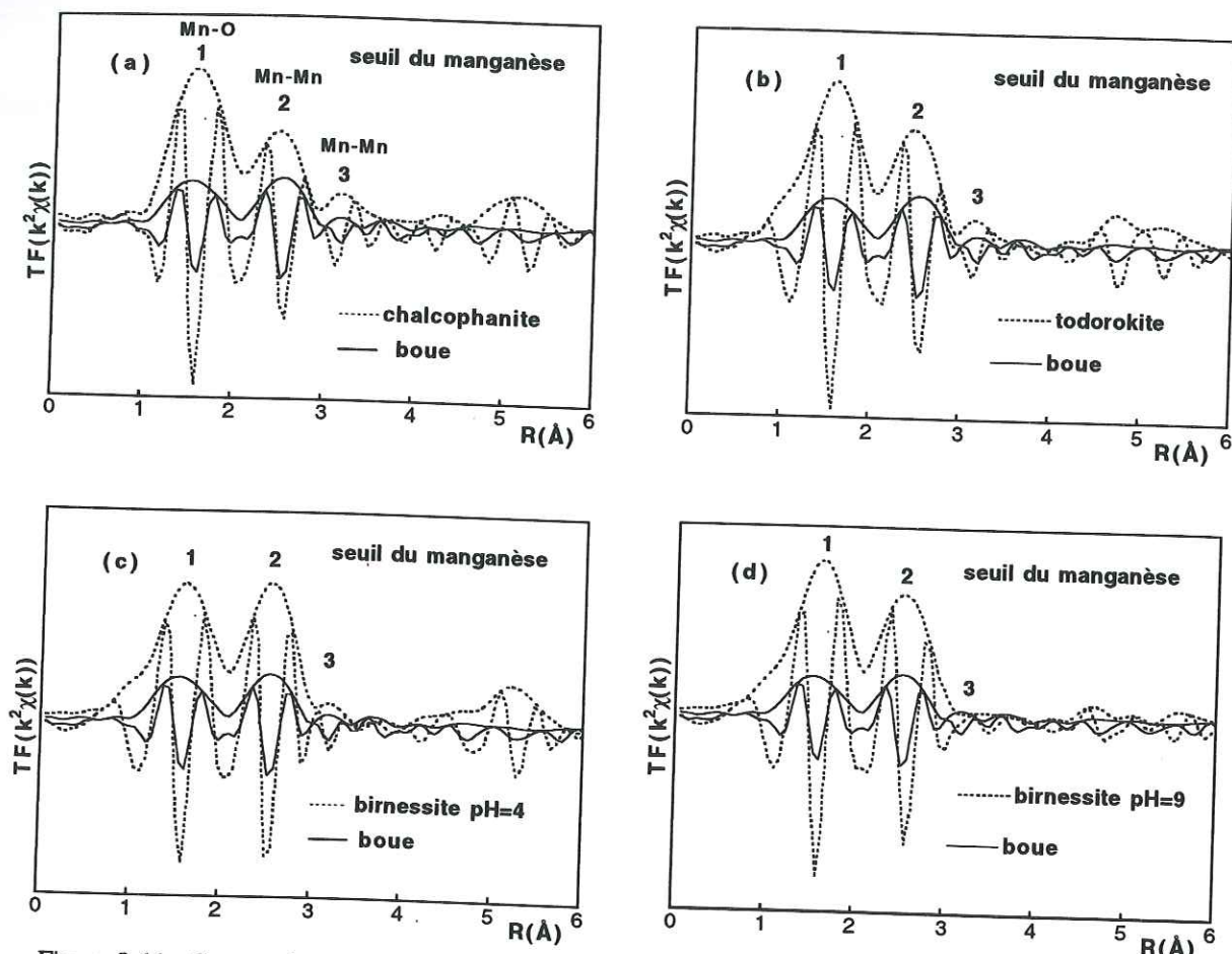
Figure 3-11 : Comparaison des FDR au seuil du manganèse de la boue d'Ambarès, de la chalcophanite (a) , de la todorokite (b) , de la birnessite hexagonale (c) et monoclinique (d) .
