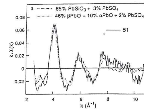
Figure 2-30 : Spectre EXAFS au seuil L_{III} du plomb d'un échantillon de sol situé dans les environs d'un ancien site de traitement de batteries au plomb (d'après Manceau et al., 1996)
