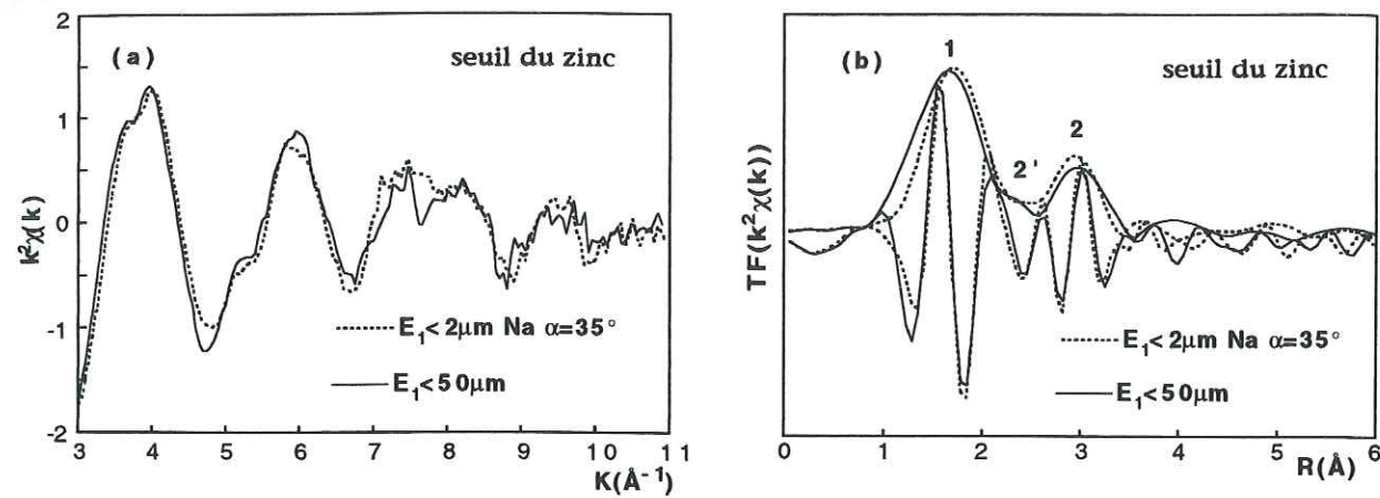
Figure 5-12 : Spectres EXAFS et FDR au seuil du zinc des fractions inférieure à 50 \mu\text{m} et argileuse d'Évin.
