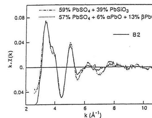
Figure 2-29 : Spectre EXAFS au seuil L_{III} du plomb d'un échantillon de sol provenant d'un ancien site de traitement de batteries au plomb (d'après Manceau et al., 1996).
