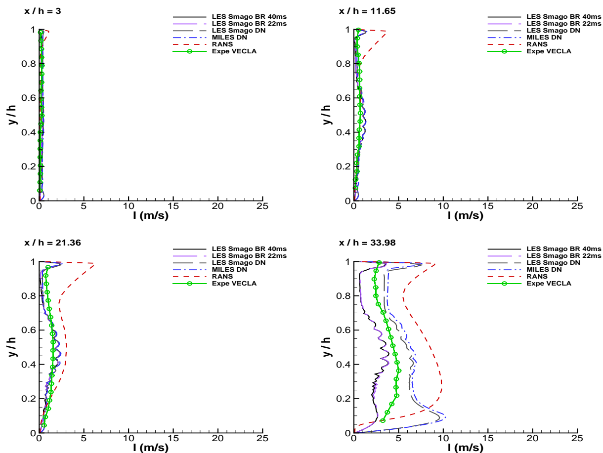
FIGURE V.9 – Intensité turbulente I = \sqrt{(v'_x)^2 + (v'_y)^2} pour 8 sections x/h de la veine. Comparaison des simulations LES/Smagorinsky avec Bruit Rouge pour une moyenne temporelle sur 40 ms, LES/Smagorinsky avec Bruit Rouge pour une moyenne temporelle sur 22 ms, LES/Smagorinsky avec Déstabilisation Numérique, MILES avec Déstabilisation Numérique et RANS avec l'expérience VECLA. (1ère PARTIE)
