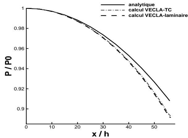
FIGURE III.4 – Comparaison Taylor-Culick/Calculs laminaires VECLA : variation de la pression moyenne adimensionnée le long de la veine.
