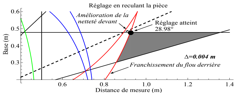
FIGURE 5.7: Optimisation par recul additionnel de la pièce
