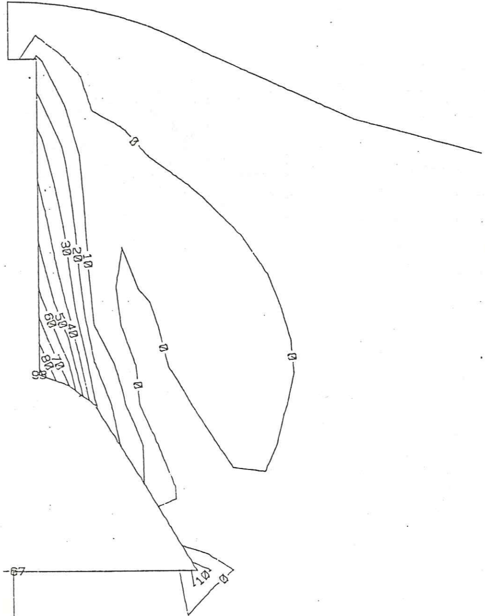
Fig. 76 Contours de la contrainte principale tangentielle 3 (MPa). Les chiffres positifs indiquent une extension.
