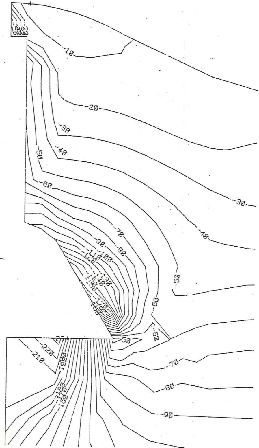
Fig. 51 Contours d'intensité de contrainte principale 1 (MPa). Les chiffres négatifs indiquent une compression.
