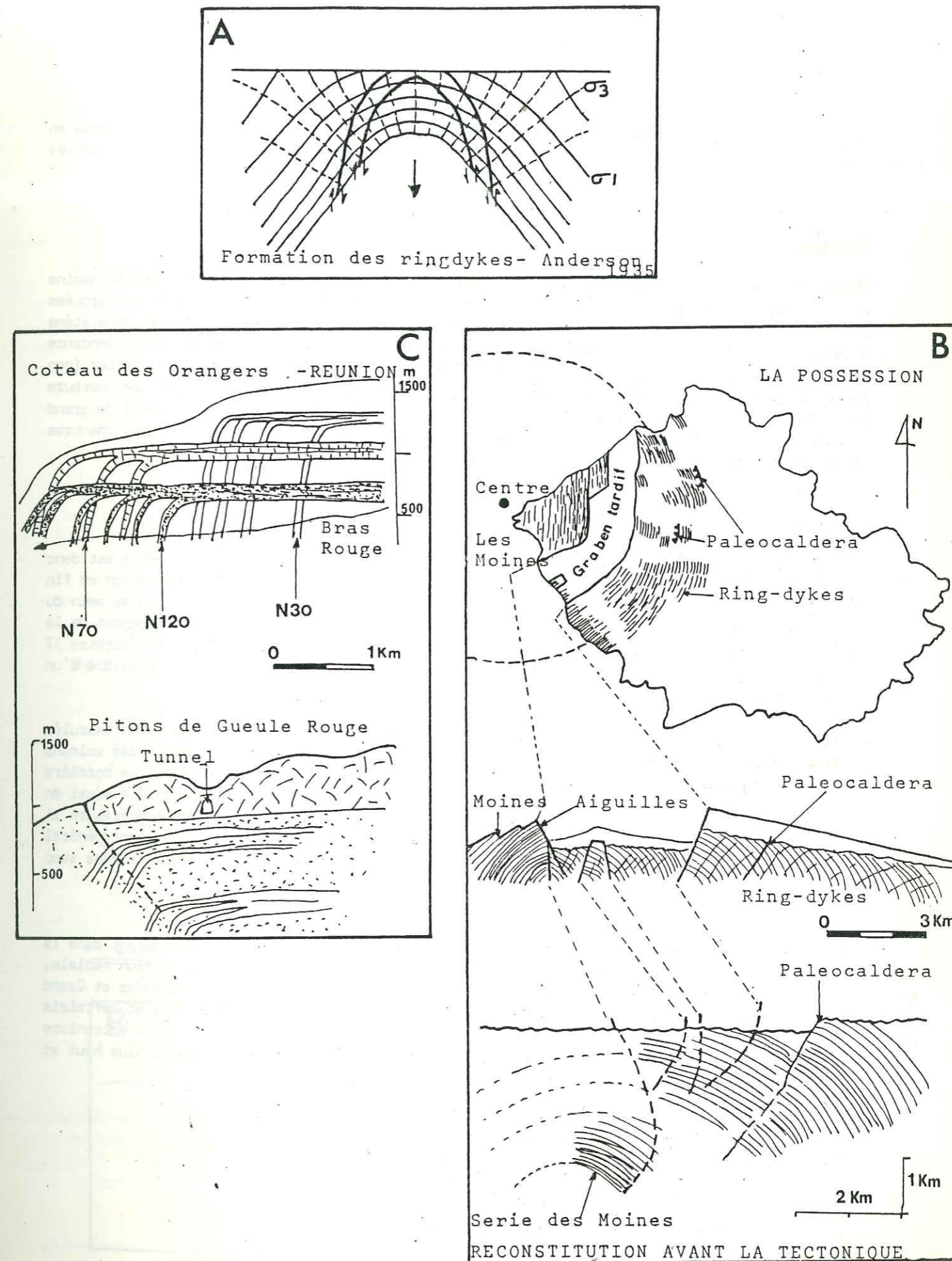
Fig. 20 A-Origine des ring dykes le long de fractures cisailantes par baisse de pression magmatique. B-Les ring dykes de la Possession. Une reconstitution du système est obtenue par soustraction de l'effet de la tectonique Holocène en horst et graben. C-Les dykes en cloche du Piton des Neiges et leur association avec le rebord de la caldera.
