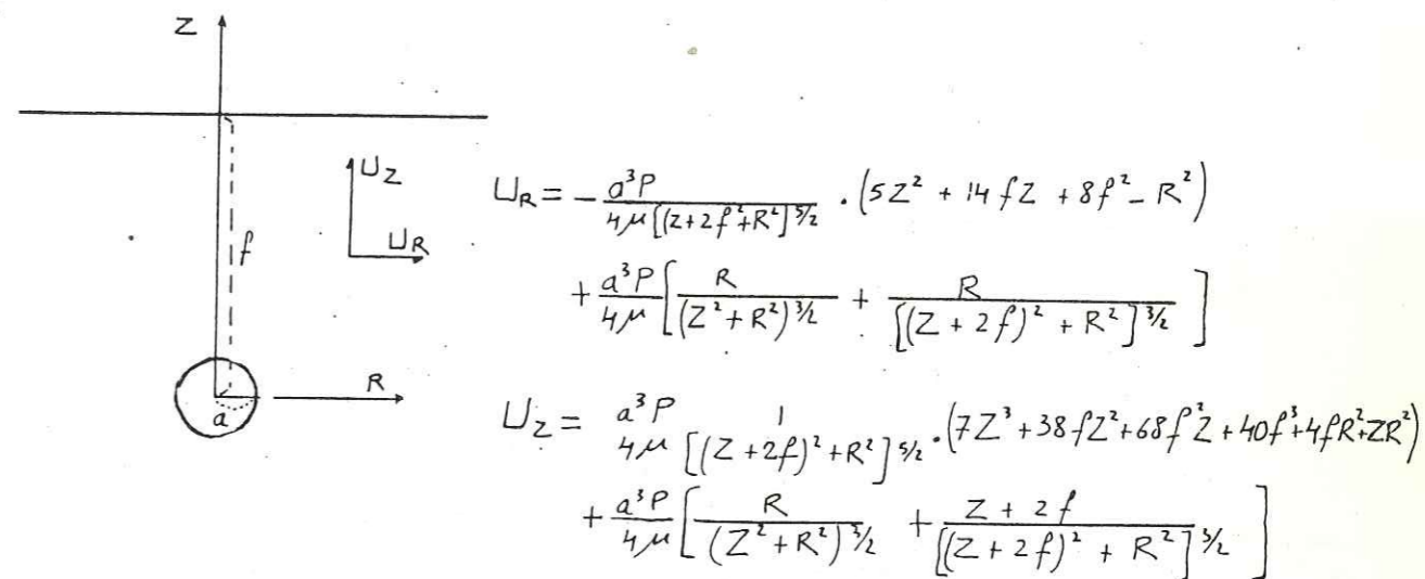
Fig. 36 Le modèle analytique de Mogi (1958) donne les déplacements horizontaux et vericaux dans un milieu semi-infini pour une chambre très petite.
