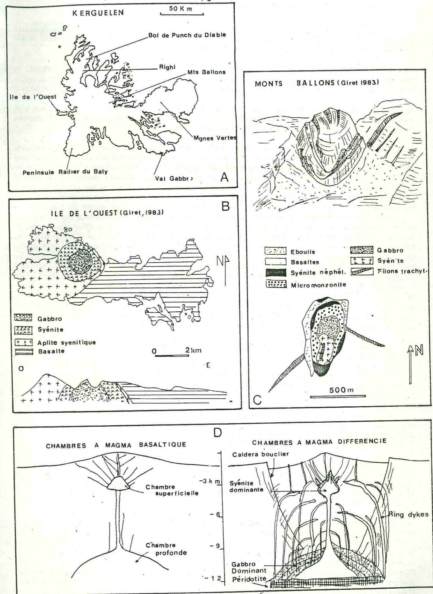
Fig. 17 A-Les complexes annulaires de Kerguelen(Giret, 1983). B-Un complexe intermédiaire. C-Un complexe hypovolcanique. D-Les modèles de chambres magmatiques
