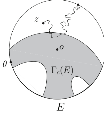
FIGURE 2.3.1 – L'hypothèse (\mathcal{H})
