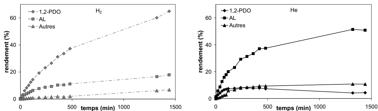
Figure 47 : Evolution des rendements des produits de la réaction en fonction du temps en présence du catalyseur 0,6% Ir/C. 100 mL 5% glycérol/NaOH 1 M, 500 mg catalyseur, autoclave en inox équipé avec un pot en Téflon ® , 50 bar H 2 (à gauche) ou 30 bar He (à droite), 180 °C. 1,2-PDO : 1,2-propanediol ; AL : acide lactique ; Autres : 1,3-propanediol, éthylène glycol, 1-propanol, 2-propanol, acide formique, acide acétique, éthanol, méthanol.
