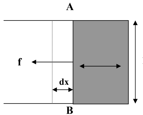
Figure II.5. Lamme mince de liquide déposée dans un cadre dont un des bords est mobile.
