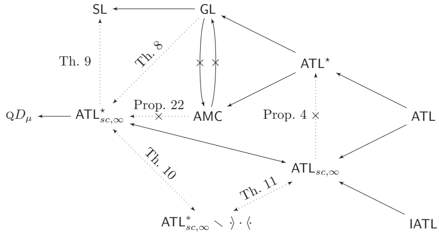
FIG. 4.6 – Expressivités comparées de ATL_{sc,\infty} et ATL^*_{sc,\infty} avec les logiques classiques
