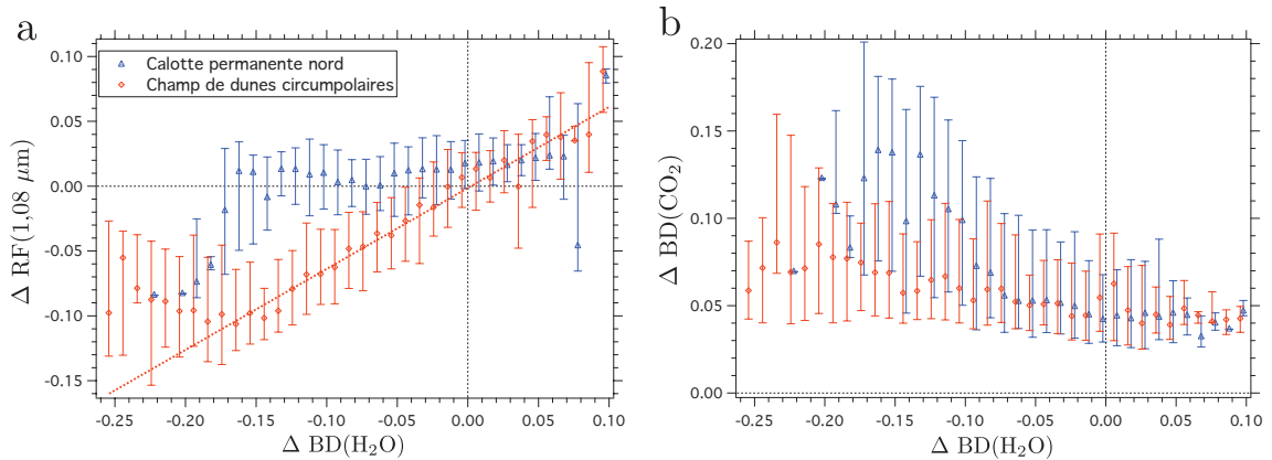
FIGURE 4.32 – (a) Variation du facteur de réflectance à 1,08 \mu\text{m} au moment du LICS en fonction de la variation de la profondeur de la bande à 1,5 \mu\text{m} de la glace de H 2 O. (b) Variation de la profondeur de la bande à 1,43 \mu\text{m} de la glace de CO 2 au moment du LICS en fonction de la variation de la profondeur de la bande à 1,5 \mu\text{m} de la glace de H 2 O. En raison de leur grand nombre, les valeurs ont été regroupées en intervalle de 0,01 unité de profondeur de bande de la glace de H 2 O. La valeur médiane des 2 paramètres dans chaque intervalle est représentée par un triangle bleu pour les points extraits de la calotte et par un diamant rouge pour les points issus du champ de dunes circumpolaires. Les barres d'erreur indiquent la plage nécessaire pour inclure 70% des valeurs.
