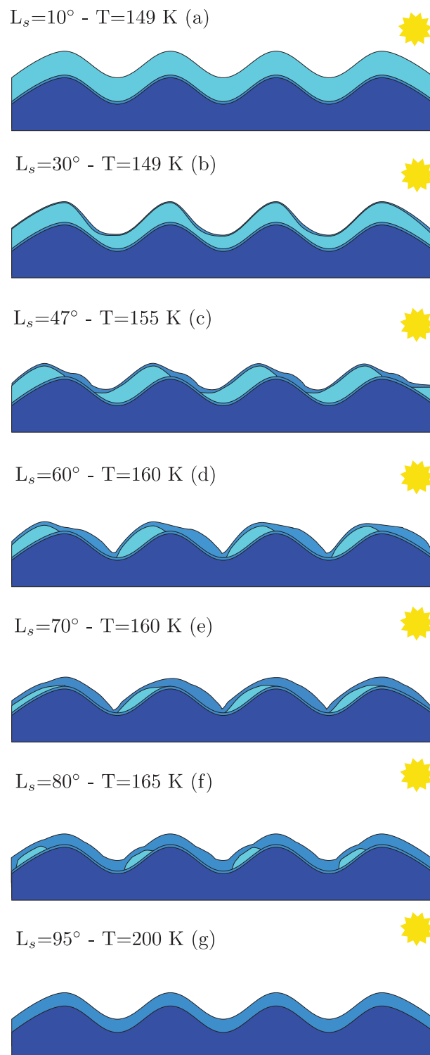
FIGURE 3.56 – Possible scénario d'évolution des dépôts saisonniers sur le plateau de Geminina Lingula présenté sous la forme de coupes à différentes longitudes solaires. L'échelle horizontale est de l'ordre de 50 m. L'échelle verticale n'est pas respectée pour plus de clarté. En bleu foncé est représentée la glace d'eau pérenne de la calotte permanente nord, en bleu la glace d'eau saisonnière et en bleu ciel la glace de CO 2 contaminée en glace d'eau et en poussière. La température indiquée est celle mesurée par l'instrument TES à une résolution spatiale de 3 kilomètres par pixel, qui ne résout pas le mélange des températures de la glace de CO 2 et H 2 O.
