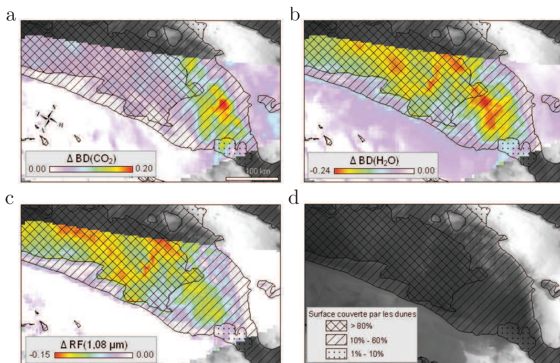
FIGURE 4.17 – Variation des 3 paramètres spectraux entre les observations 2924_0 (L s =42,1°) et 2972_1 (L s =48,1°) : (a) profondeur de la bande d'absorption à 1,43 \mu\text{m} de la glace de CO 2 , (b) profondeur de la bande d'absorption à 1,5 \mu\text{m} de la glace de H 2 O et (c) facteur de réflectance à 1,08 \mu\text{m} . Les surfaces hachurées et pointillées indiquent la densité du champ de dunes. Le fond de la carte est une mosaïque d'images MOC acquises en été (Caplinger & Malin, 2001).
