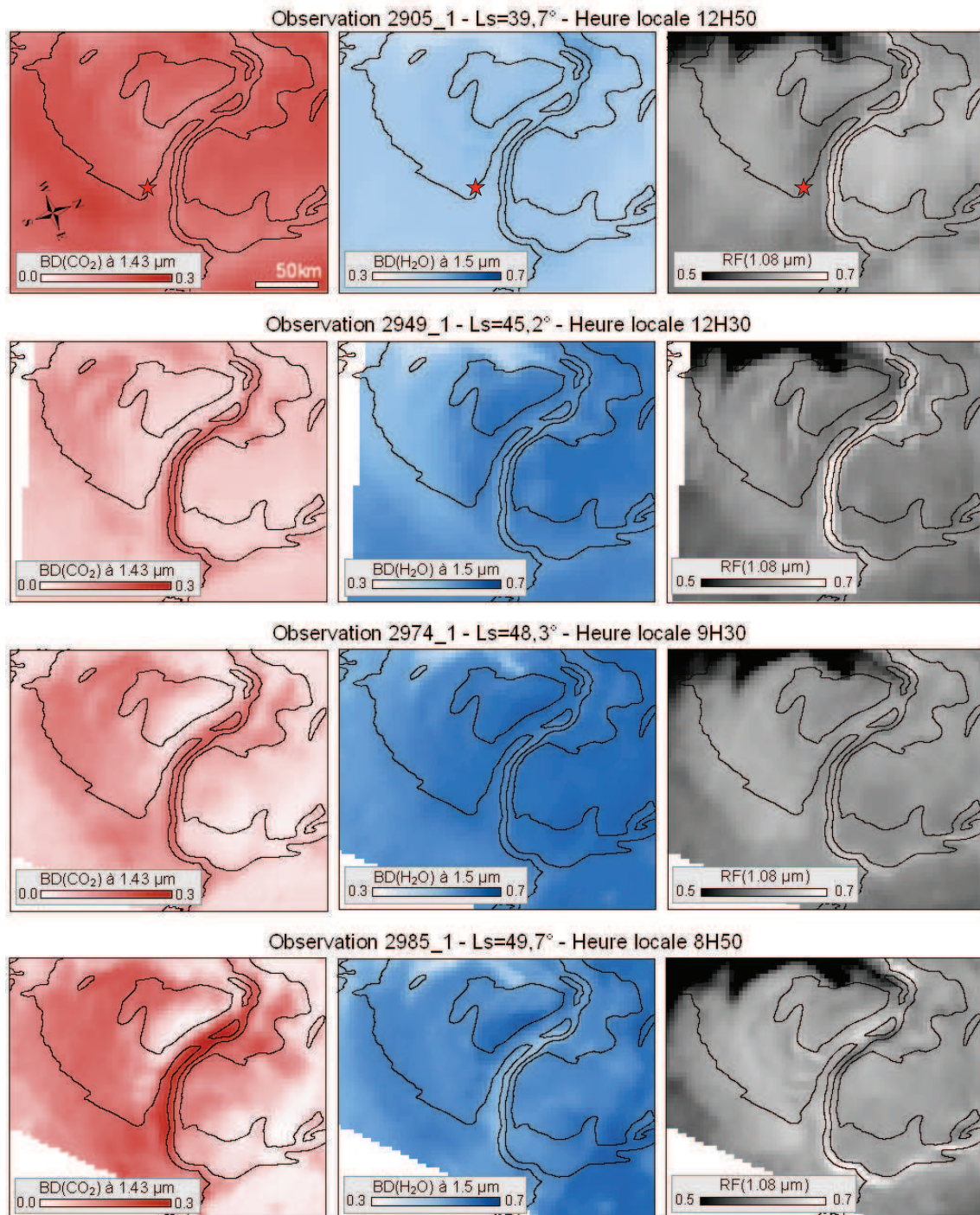
FIGURE 4.4 – Evolution des dépôts saisonniers nord au niveau du site de Rupes Tenuis en terme de profondeur de la bande à 1,43 \mu\text{m} de la glace de \text{CO}_2 (colonne de gauche), profondeur de la bande à 1,5 \mu\text{m} de la glace de \text{H}_2\text{O} (colonne du milieu) et facteur de réflectance à 1,08 \mu\text{m} (colonne de droite) pour 4 observations OMEGA acquises entre L_s 39,7^\circ et 49,7^\circ . L'étoile rouge indique la position de la région d'intérêt pour laquelle les paramètres spectraux et la température de surface sont tracés sur la figure 4.3. La topographie est indiquée par des lignes de niveau espacées de 500 m.
