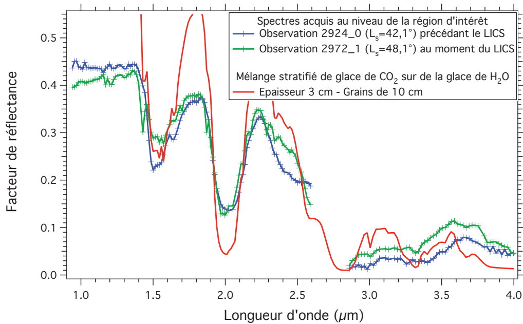
FIGURE 4.19 – Comparaison de deux spectres extraits au niveau de la région d'intérêt, là où le LICS est le plus intense, avant le LICS (spectre bleu, observation 2924_0) et au moment du LICS (spectre vert, observation 2972_1). Les deux spectres ont été corrigés uniquement de l'effet des gaz car la forte contamination en poussière de la surface empêche l'utilisation de la méthode de correction de l'effet des aérosols. Le spectre rouge est issu de la modélisation du transfert radiatif dans un mélange stratifié où une couche de glace de CO 2 de 3 cm d'épaisseur constituée de grains de 10 cm surmonte une couche de glace de H 2 O composée de grains de 150 \mu\text{m} .
