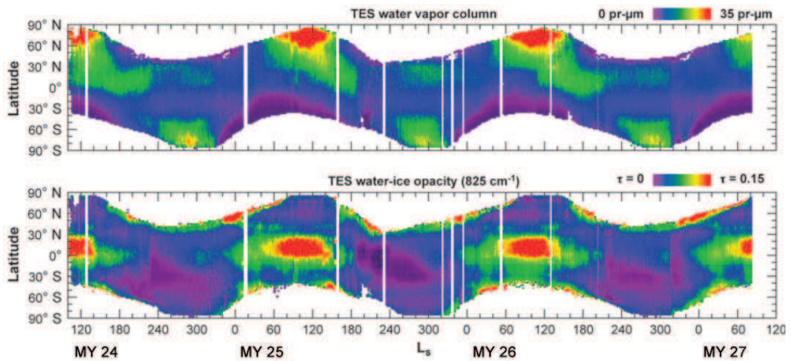
FIGURE 1.23 – Densité de colonne de vapeur d'eau (haut) et opacité des nuages de glace d'eau (bas) sur trois années martiennes en fonction de la latitude. Ces figures ont été obtenues en moyennant les mesures selon la longitude. Notez la répétabilité du cycle de la vapeur d'eau et des nuages, ce dernier étant caractérisé par deux maxima locaux : la ceinture de nuages tropicaux en été et le polar hood proche du bord des condensats saisonniers. Figure extraite de Smith (2008).
