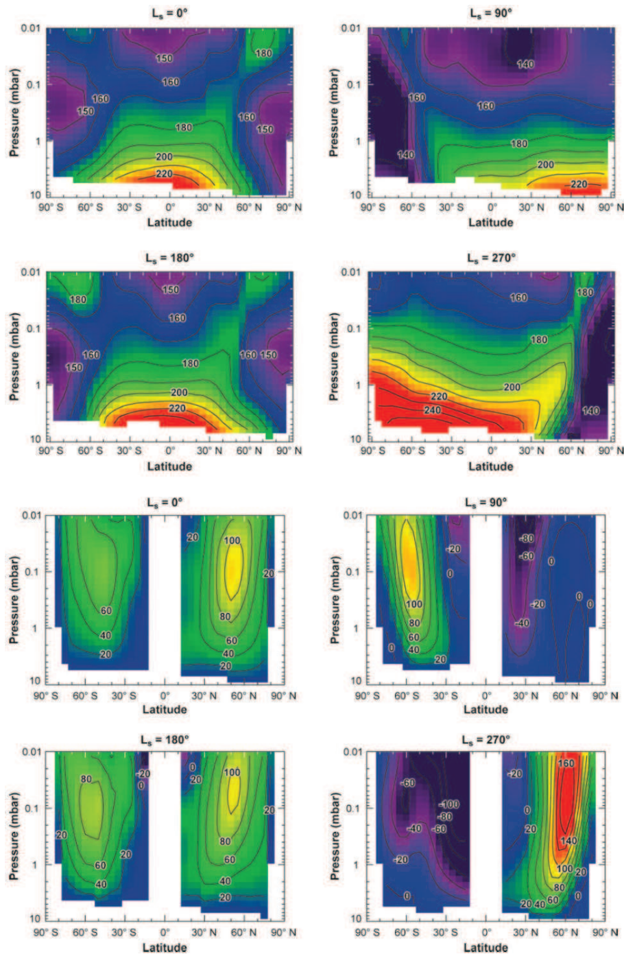
FIGURE 1.11 – Température atmosphérique (en haut) et vents zonaux (en bas) à 14 h en fonction de la latitude et de la pression, pour quatre longitudes solaires. Le sommet des figures, à 1 Pa, correspond à une altitude d'environ 65 km au-dessus de la surface. Les données de température ont été obtenues par l'instrument TES à bord de Mars Global Surveyor. Les vents zonaux sont déduits de l'équation du vent thermique. L'unique cellule de Hadley aux solstices se dédouble aux équinoxes. Notez aux quatre saisons le réchauffement adiabatique induit par les branches descendantes des cellules de Hadley. Les latitudes polaires sont le siège de températures extrêmement basses en hiver, favorables à la condensation du \text{CO}_2 atmosphérique. Image extraite de (Smith, 2008).
