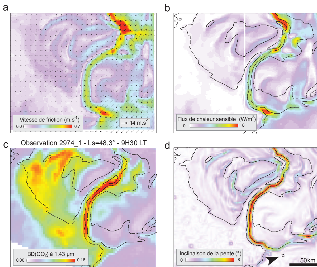
FIGURE 4.10 – Résultats de la simulation méso-échelle des caractéristiques de l’atmosphère à L_s=50^\circ au niveau de la région de Rupes Tenuis, effectuée à une résolution horizontale de 2 km. (a) Vitesse de friction ; (b) Flux de chaleur sensible entre l’atmosphère et la surface. Les flèches sur la figure a donnent l’intensité et la direction du vent à 10 m au-dessus du sol. Ces flèches sont tracées tous les 4 points de grille. Toutes ces quantités ont été moyennées sur une journée. (c) Profondeur de la bande à 1,43 \mu\text{m} de la glace de \text{CO}_2 pour l’observation 2974_1 acquise à L_s 48,3^\circ et 9H30 heure locale. d : Inclinaison de la pente d’après les données MOLA rééchantillonnées à l’échelle spatiale de la simulation. La topographie est indiquée par des lignes de niveau espacées de 500 m.
