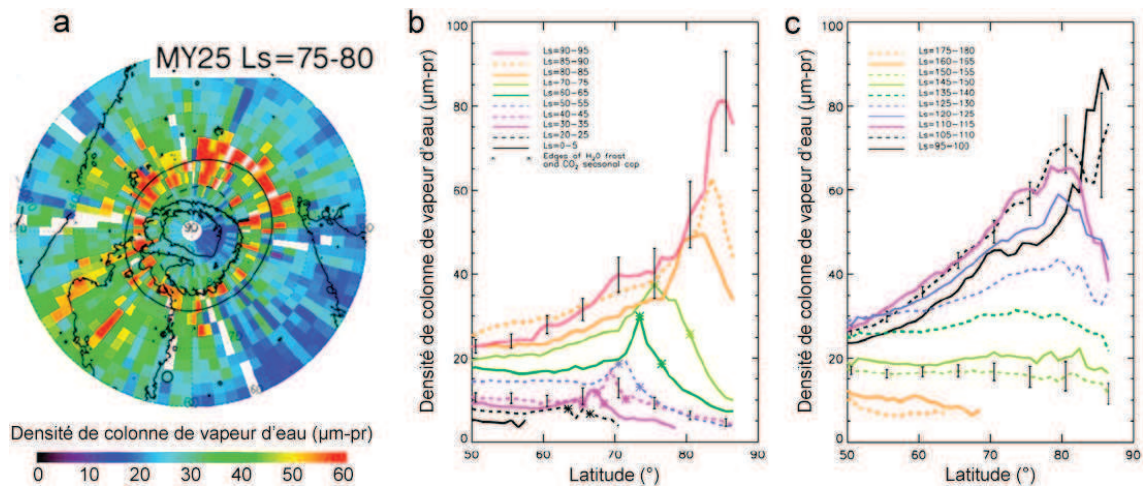
FIGURE 1.32 – Mise en évidence par l'instrument TES d'un anneau de vapeur d'eau entourant les dépôts saisonniers nord lors de leur retrait. a : Carte en projection polaire de la densité de colonne de vapeur d'eau obtenue pour L_s = 75-80 . La topographie MOLA est indiquée par des lignes de niveau espacées d'un 1 km. La limite des condensats de CO 2 et de H 2 O est représentée respectivement en trait pointillé et en trait plein. Ces limites sont extraites de Titus (2009). b et c : Moyennes longitudinales de la densité de colonne de vapeur d'eau pendant le printemps (b) et l'été (c) de l'année martienne 25. Sur la figure b, les étoiles indiquent la limite des condensats de CO 2 et de H 2 O, la limite de la glace de H 2 O étant celle située à la latitude la plus basse. Figures d'après Pankine et al. (2010).
