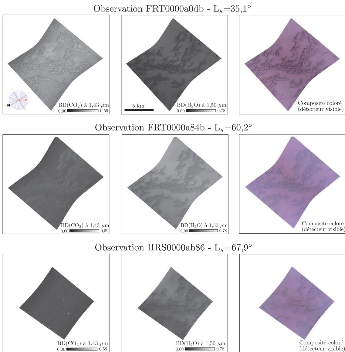
FIGURE 4.21 – Evolution des dépôts saisonniers nord observés par CRISM au niveau du site de Olympia Undae pendant l'année martienne 29, entre L_s 35,1° et 67,9°. Colonne de gauche : profondeur de la bande à 1,43 \mu\text{m} de la glace de CO 2 . Colonne du milieu : profondeur de la bande à 1,5 \mu\text{m} de la glace de H 2 O. Colonne de droite : composite coloré réalisé à partir des données du détecteur visible.
