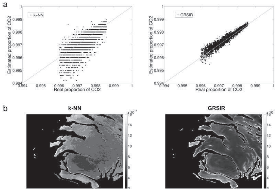
FIGURE 2.18 – Comparaison entre les méthodes k-NN et GRSIR. a : Estimation de la proportion de glace de \text{CO}_2 en fonction de sa proportion réelle par la méthode k-NN (gauche) et GRSIR (droite). b : Estimation de la proportion de poussière contenue dans la calotte permanente sud de Mars par la méthode k-NN (gauche) et GRSIR (droite). Figures extraite de Bernard-Michel et al. (2009).
