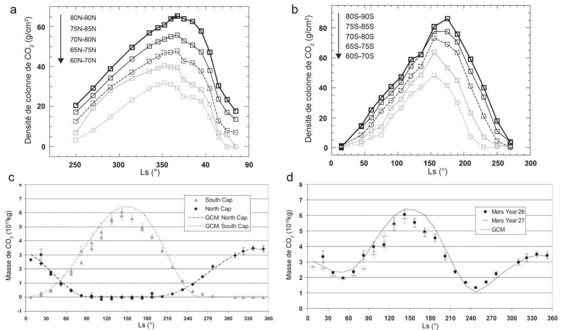
FIGURE 1.19 – Evolution hivernale et printanière de la densité de colonne de glace carbonique pour plusieurs bandes de latitude de l'hémisphère nord (a) et sud (b) de Mars, obtenue grâce aux mesures de l'instrument HEND (d'après Litvak et al. (2005)); c : Evolution saisonnière de la masse des dépôts saisonniers nord et sud obtenue grâce aux mesures de l'instrument GRS et comparaison aux prédictions du GCM de la NASA Ames (Haberle et al. , 1999); d : Evolution saisonnière de la masse totale des dépôts saisonniers pendant les années martiennes 26 (points) et 27 (traits) et comparaison aux prédictions du GCM (d'après Kelly et al. (2006)).
