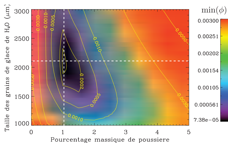
FIGURE 3.48 – Plan de la distance minimale entre le spectre OMEGA RAC 1157_2 et les spectres synthétiques lorsqu’on fait varier les combinaisons de proportion massique de poussière et de taille de grains de glace d’eau. Le contour central sans label correspond à la valeur 1.10^{-4} .
