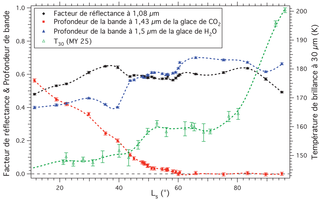
FIGURE 3.29 – Plateau de Gemina Lingula. Evolution temporelle du facteur de réflectance à 1,08 µm (diamants noirs), de la profondeur de la bande d'absorption à 1,43 µm de la glace de CO 2 (carrés rouges), de la profondeur de la bande d'absorption à 1,5 µm de la glace de H 2 O (triangles bleus) et de la température de brillance à 30 µm (triangles verts) dans une région de 182 km 2 située au sommet du plateau de Gemina Lingula. A une date donnée, la dispersion des valeurs des 3 paramètres spectraux dans la région d'intérêt est généralement inférieure à l'incertitude sur la détermination de ces paramètres, indiquée par les barres d'erreur. Par contre, la dispersion des valeurs de température de brillance au sein de la région est plus importante que l'erreur sur l'estimation de cette température. L'évolution temporelle de chaque grandeur est ajustée par une fonction spline qui a pour but de guider visuellement le lecteur.
