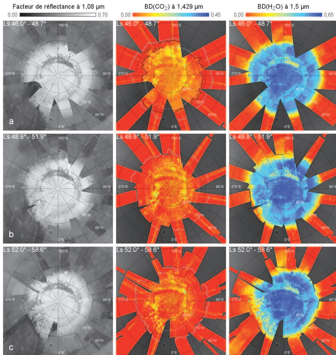
FIGURE 3.12 – Même légende que pour la figure 3.7 mais pour (a) L s 46,0°-48,7°, (b) L s 48,8°-51,9° et (c) 52,0°-58,6°.
