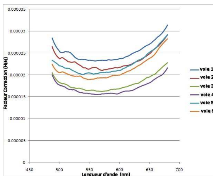
FIGURE 2.22 – Facteurs de correction de la réponse spectrale du système configuré pour l’acquisition à l’excitation de 360nm (appliqués à chaque voie d’acquisition)
