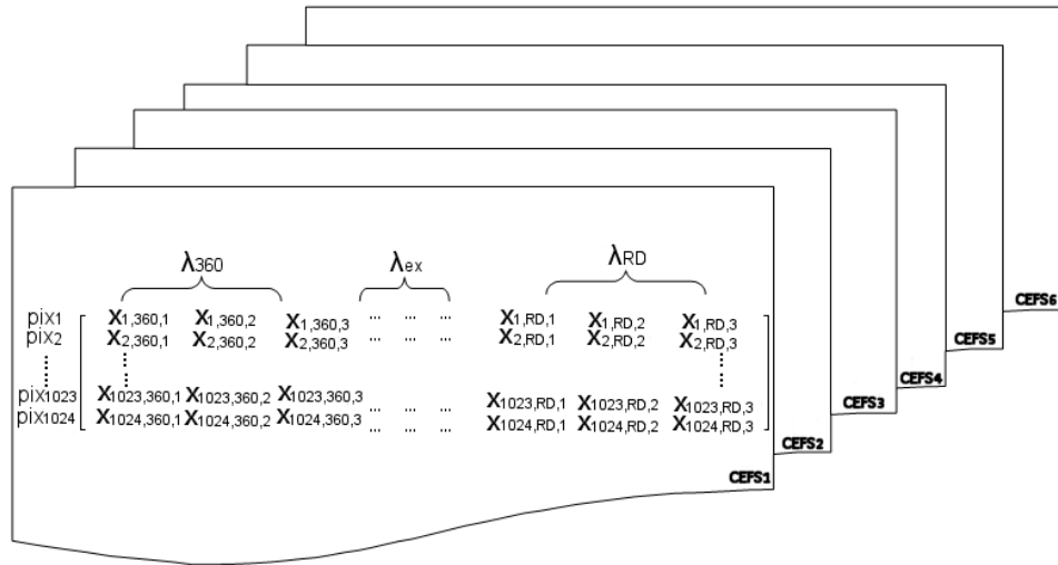
FIGURE 4.11 – Organisation de nos données spectrales (pour un site de mesure/individu) dans une matrice 3D M_i . La matrice contient 6 tableaux correspondant à 6 distances interfibrilles ( CEFS ). Pour chaque tableau, les lignes correspondent à l'arrangement des colonnes de pixels sur le capteur CCD. Chaque colonne de données représente une acquisition du spectre mesuré pour une excitation et à une distance interfibrilles
