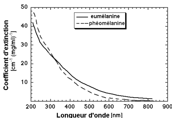
FIGURE 1.7 – Spectres de coefficient d'extinction molaire pour les deux types de mélanine dans la peau humaine : eumélanine (ligne foncée) et phéomélanine (ligne claire) [OMLC, 2004]
