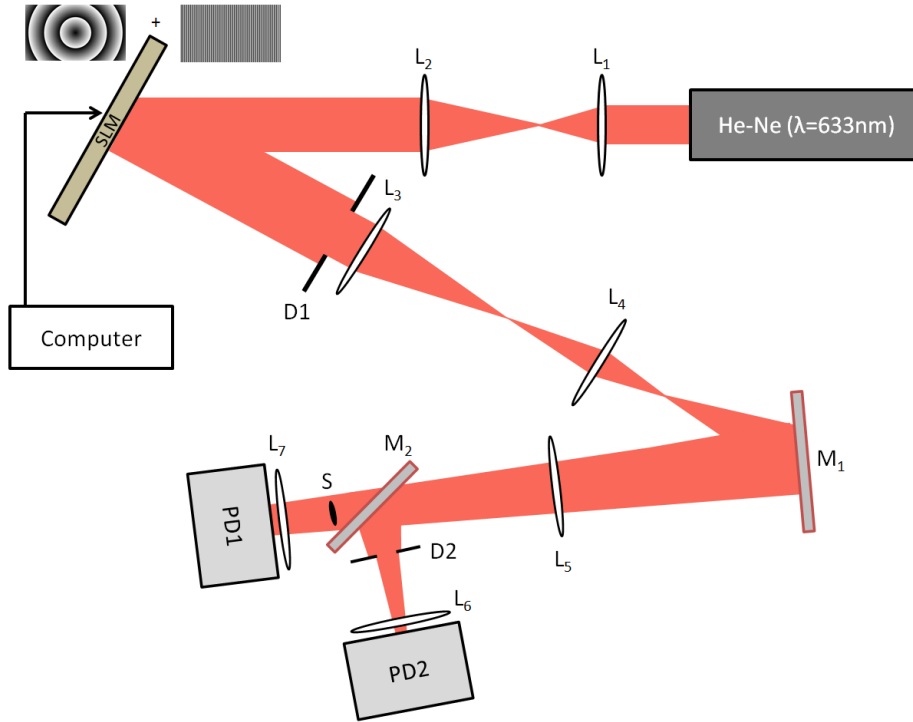
FIGURE 2.21 – Dispositif expérimental comportant un SLM de phase et un diagnostic de divergence basé sur un stop et un diaphragme. Les focales utilisées sont les suivantes : f_1 = 50\text{mm} , f_2 = 150\text{mm} , f_3 = 250\text{mm} , f_4 = 40\text{mm} , f_5 = 500\text{mm} et f_6 = f_7 = 50\text{mm} .
