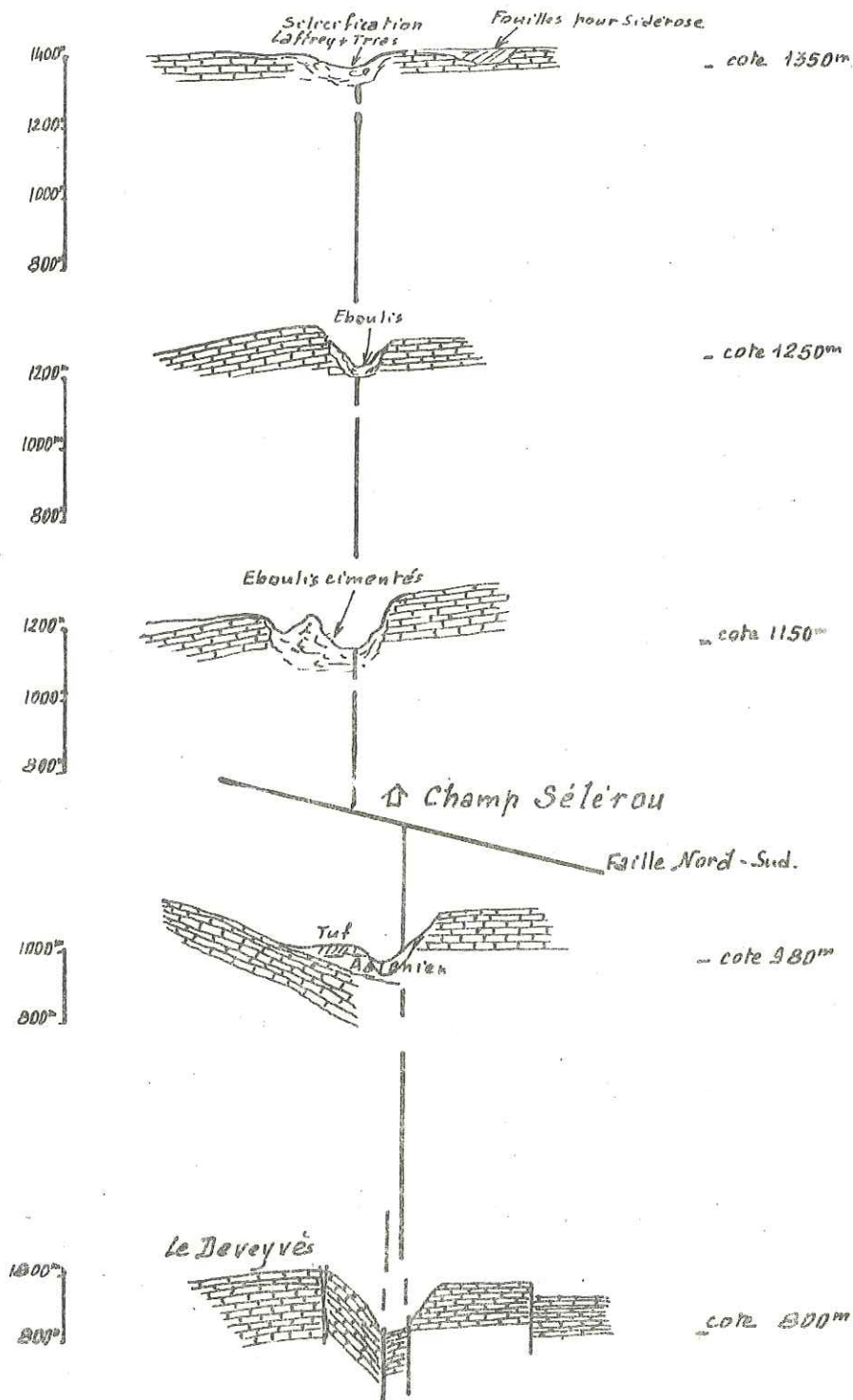
Faille Nord 50°E de Champ Sélérou
