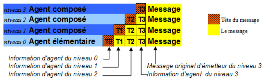
FIGURE 5.7 – Modification du contenu des messages dans le modèle SMA-Récuratif
