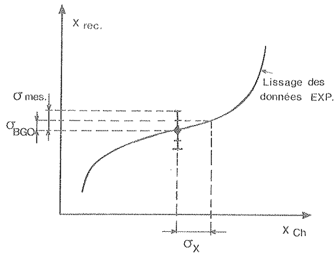
Figure II.30 : Schématisation de la méthode d'extraction de la résolution spatiale.
