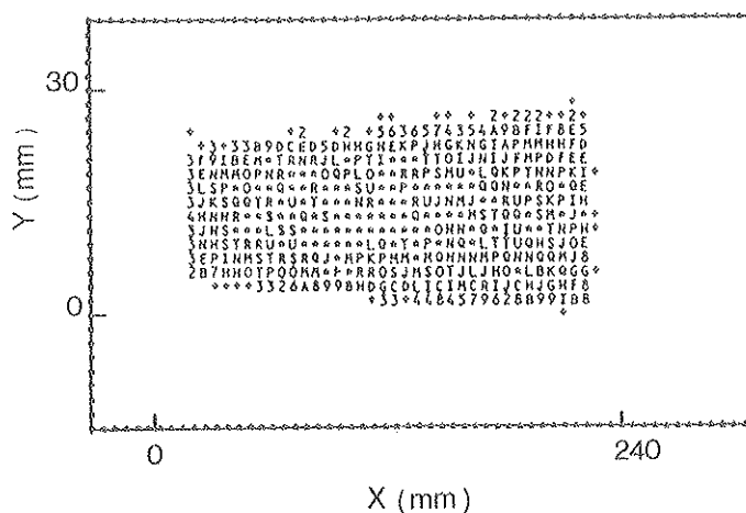
Figure B.2 : Image reconstruite à l'aide des chambres à fils d'un cristal de BGO tronç-pyramidal.
