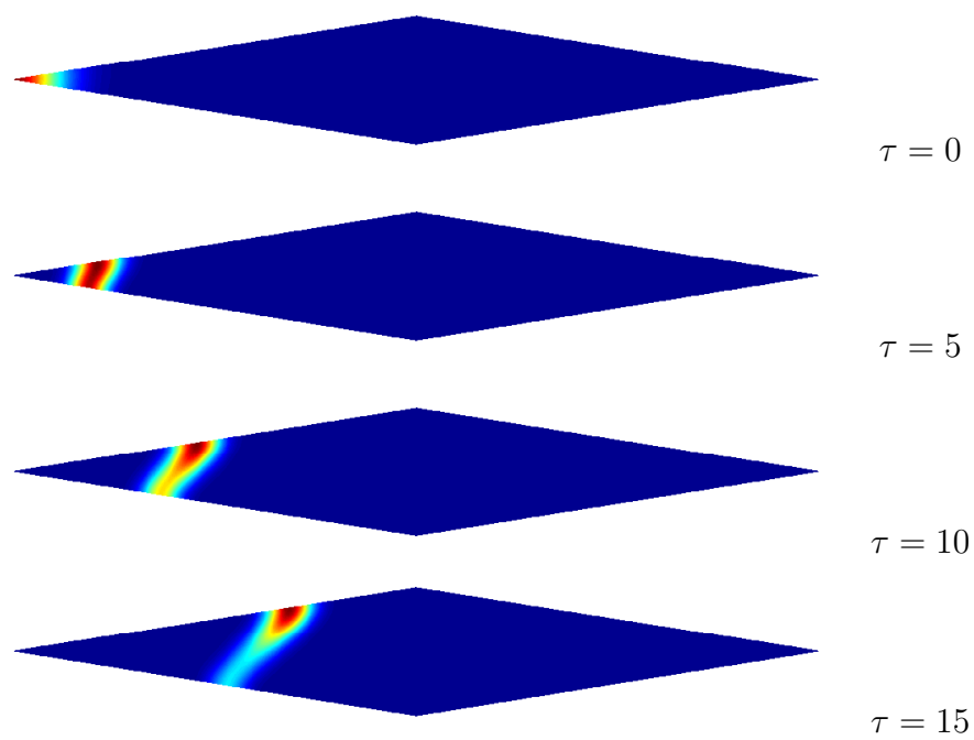
FIGURE 5.6 – Valeur des paramètres : \gamma = \frac{\pi}{2} , \theta = \frac{\pi}{4} et \alpha = \frac{\pi}{10} . Les vecteurs propres associés \check{\xi}(\gamma, \theta, \alpha, \tau) pour \tau = 5k , 0 \leq k \leq 3 . Domaine de calcul : \text{Los}(20, 35, \frac{\pi}{10}) . Degré : \mathbb{Q}_8 .
