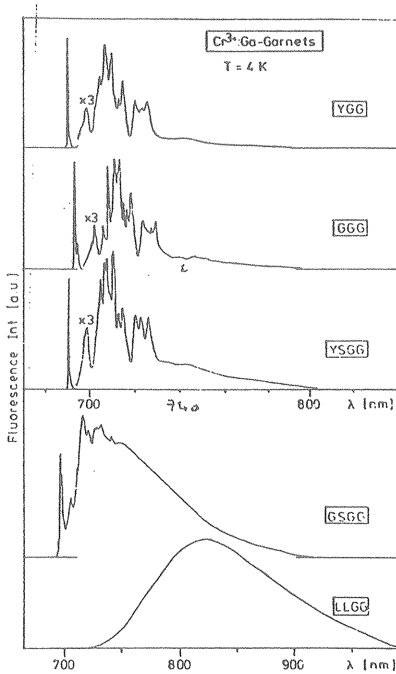
Figure 3 Spectre de fluorescence de Cr 3+ dans YGG, GGG, YSGG, GSGG et LLGG [4].
