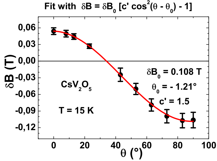
FIGURE 4.23 – Variation angulaire du splitting \delta B pour CsV_2O_5 à T = 15 K.
