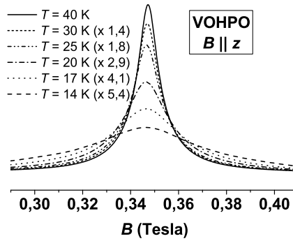
FIGURE 4.6 – Les profils des courbes d'absorption des trois composés entre 12 K et 40 K suivant la direction magnétique z . Dans la légende, les valeurs en face des températures sont les facteurs d'agrandissement des courbes. Ces facteurs d'agrandissement sont tels que les courbes d'absorption ont toutes la même aire en dessous.
