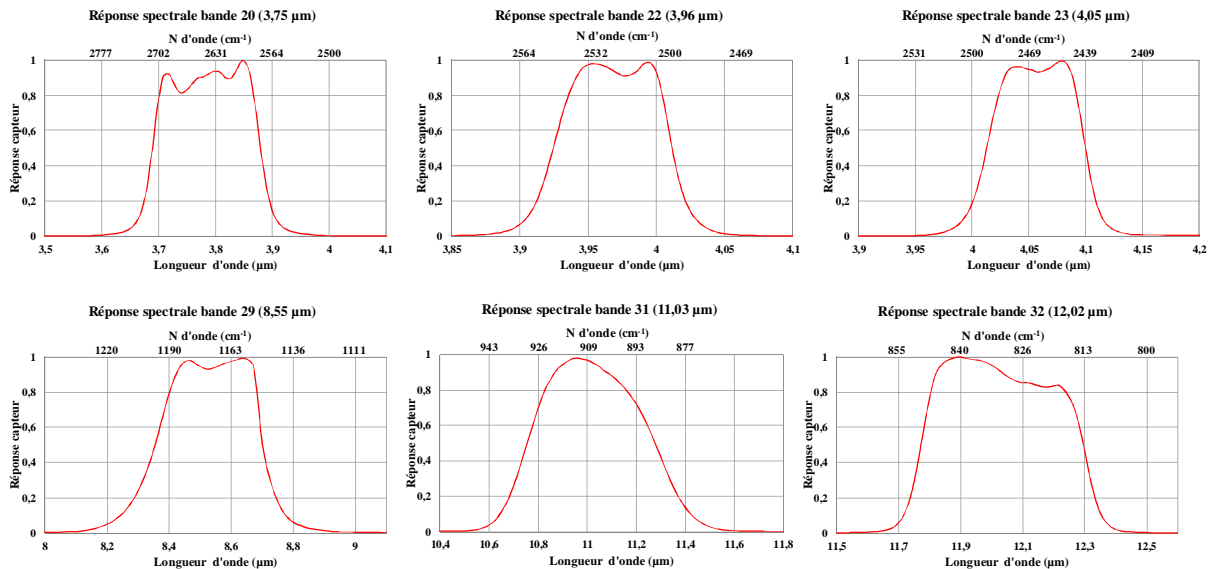
Figure 4.7 Réponse spectrale des canaux d'émissivité MODIS.
