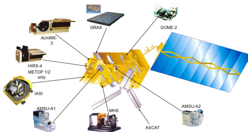
Figure 3.3 Instruments à bord du satellite METOP-A.
