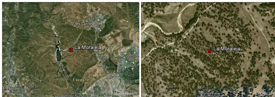
Figure 3.16 Idem figure 3.13 mais pour “La Moraleja”.
