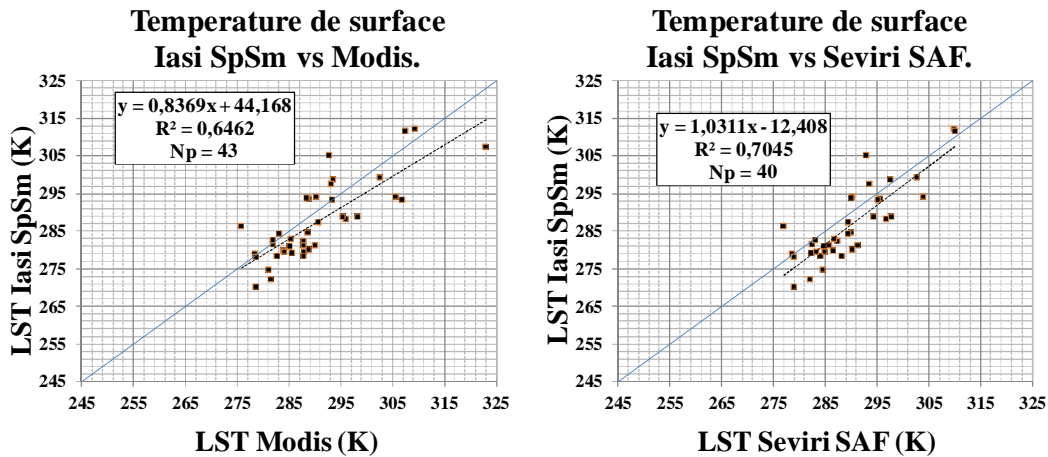
Figure 4.24 Validation LST pour les points de contrôle avec végétation moyenne (La Moraleja, Casinos, São Matias et Maroc Toubkal).
