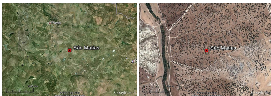
Figure 3.18 Idem figure 3.13 mais pour “São Matias”.
