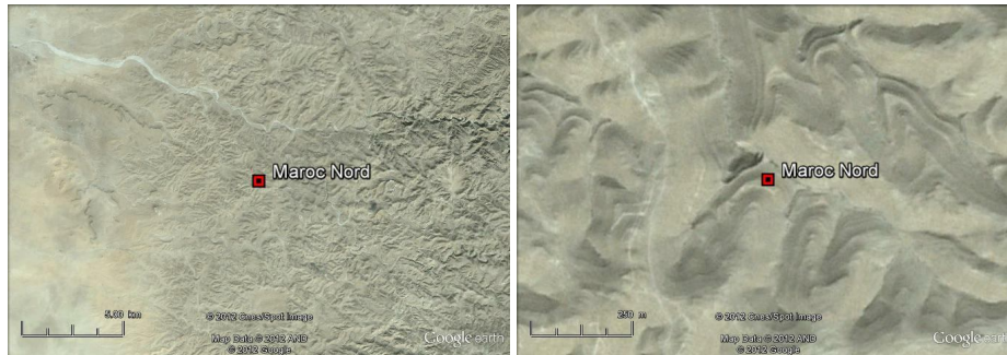
Figure 3.19 Idem figure 3.13 mais pour “Maroc Nord”.
