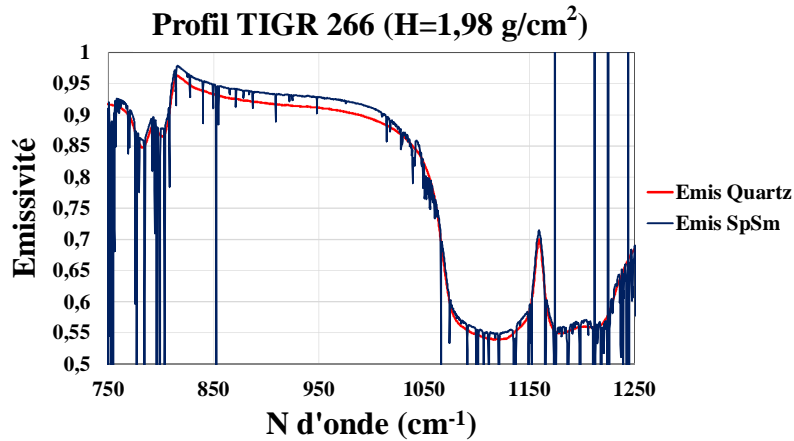
Figure 2.12 Emissivité de quartz restituée avec la méthode SpSm pour un profil humide (TIGR 266; H=1,98 \text{ g/cm}^2 ) avec un bruit de 1 K en température.
