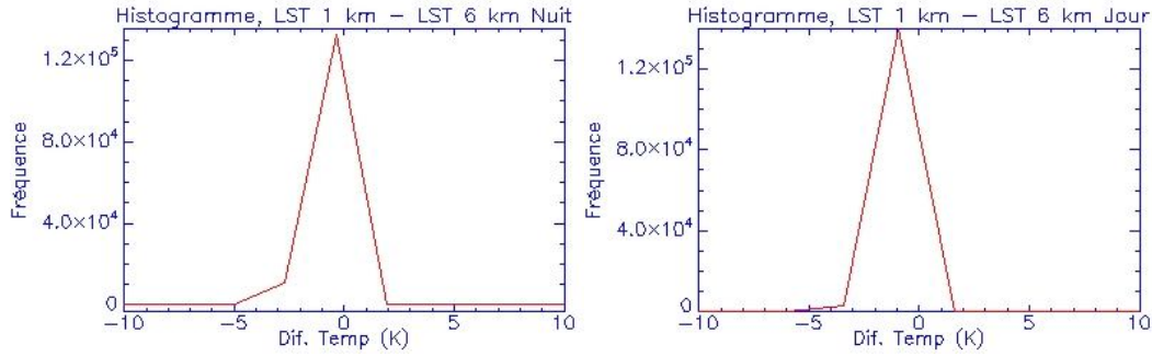
Figure 4.6 Distribution de températures LST MODIS.
