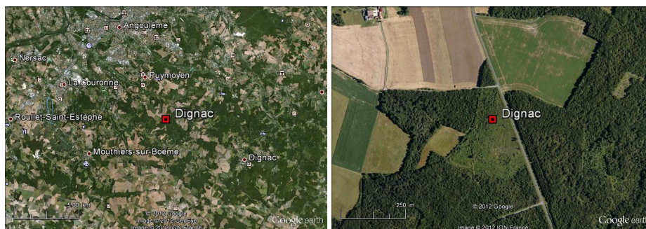
Figure 3.14 Idem figure 3.13 mais pour “Dignac”.
