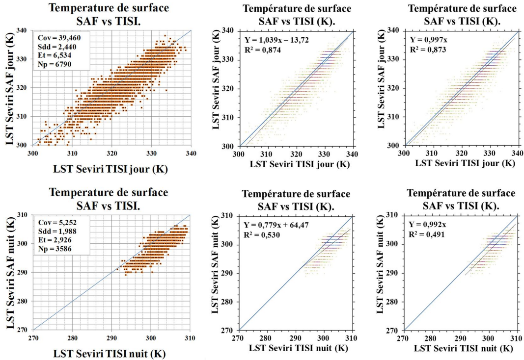
Figure 4.16 Dispersion LST SEVIRI TISI et SAF pour le 3 juillet 2008. En haut image de jour et en bas image de nuit.
