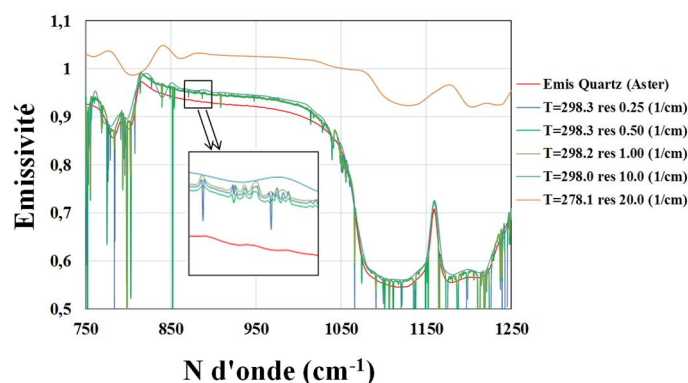
Figure 2.21 Application SpSm avec différentes résolutions des données sur le profil TIGR 266 (H=1.98 g/cm 2 ), LST=300K, introduction d'une erreur d'un degré en température.
