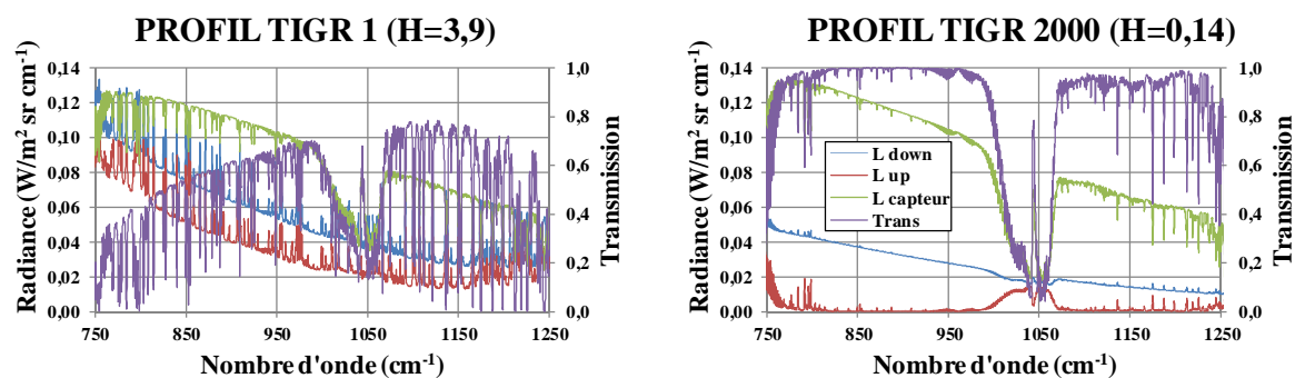
Figure 2.17 Radiances atmosphériques pour des profils atmosphériques humide (gauche) et sec (droite).
