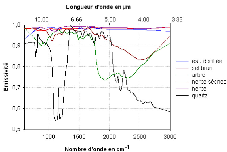
Figure 1.2 Signatures spectrales représentatives de différents sols.
