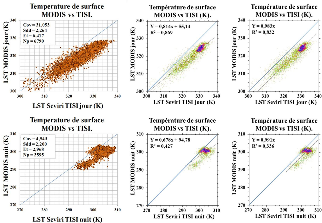
Figure 4.14 Dispersion LST MODIS et LST SEVIRI TISI pour le 3 juillet 2008. En haut, image de jour et en bas, image de nuit.
