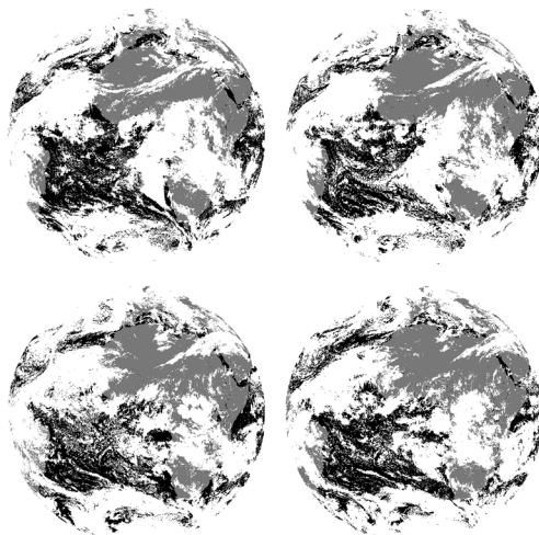
Figure 3.9 Exemples de produits SEVIRI « cloudmask » correspondant au 1 janvier 2008 à 00h, 06h, 12h et 18h respectivement.
