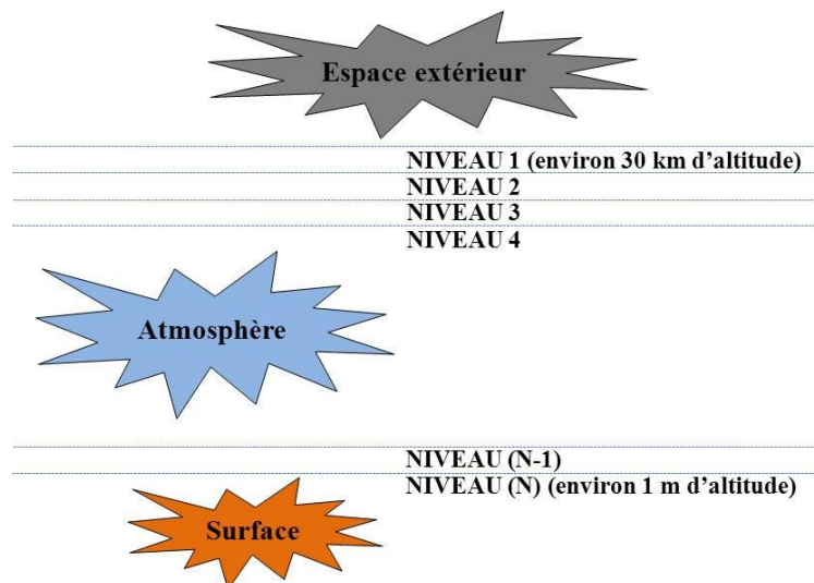
Figure 1.4 Schéma d'un profil atmosphérique.
