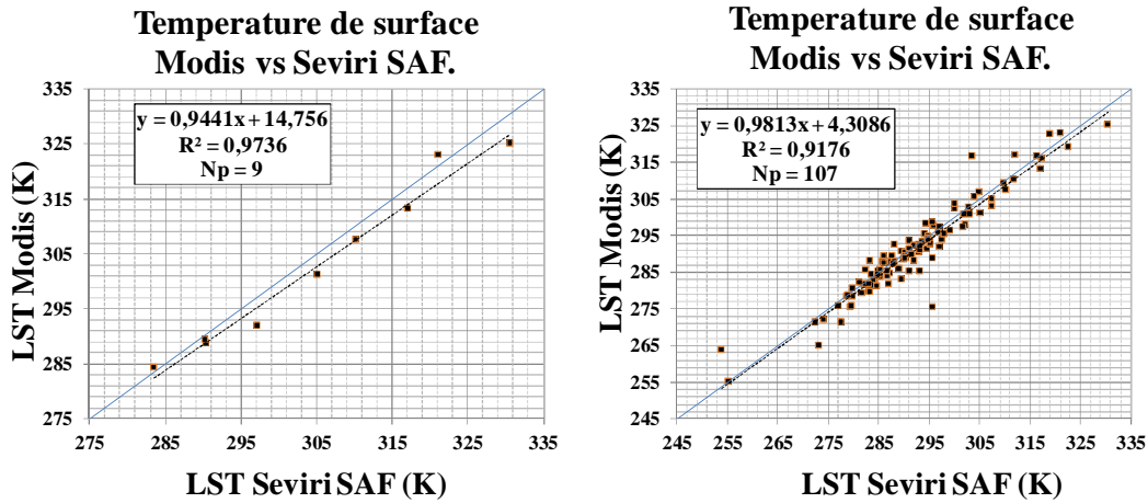
Figure 4.13 Comparaison LST MODIS vs SEVIRI SAF pour les points de contrôle, à gauche pour le 3 juillet 2008 et à droite pour toutes les dates retenues (table 4.2).
