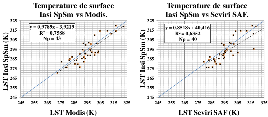
Figure 4.23 Validation LST pour les points de contrôle désertiques (Maroc Nord, Maroc Algérie, Algérie Ghardasa et Algérie Est).
