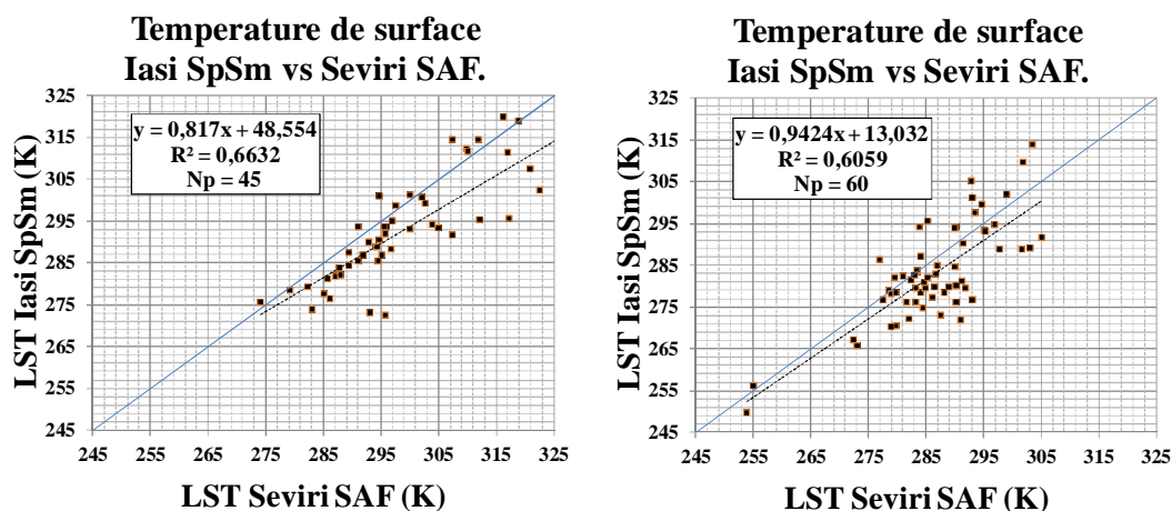
Figure 4.20 Validation des températures SpSm estimées sur les points de contrôle et pour toutes les dates vs SEVIRI. A droite de nuit, à gauche de jour.
