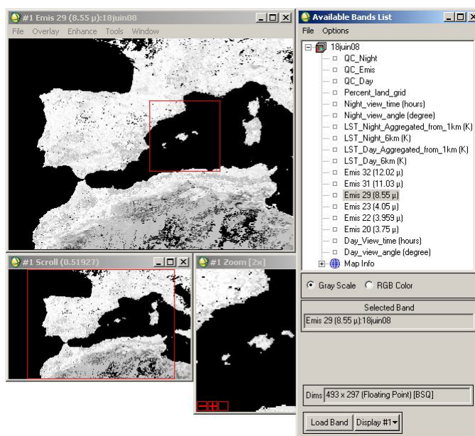
Figure 4.1 Image MOD11B1 avec ses 18 bandes correspondant au 18 juin 2008 couvrant la zone d'étude.
