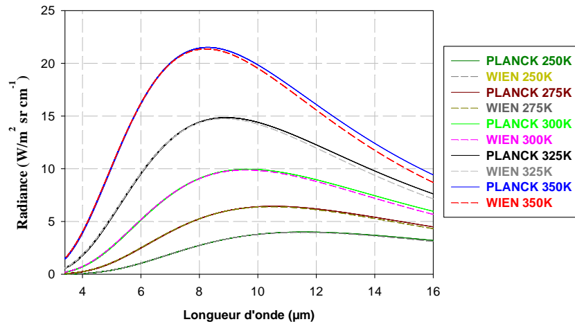
Figure 2.9 Approximation de Wien de l'expression de corps noir de Planck.
