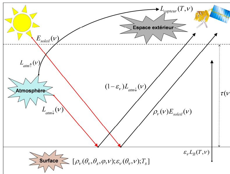
Figure 1.3 Schéma du bilan énergétique.
