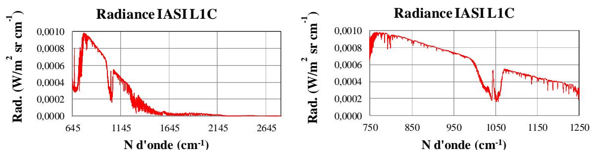
Figure 3.7 Exemple de données radiance IASI. A gauche l'intervalle spectral total de IASI et à droite la représentation comprise entre 750 et 1250 \text{cm}^{-1} .
