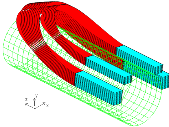
FIGURE 8.10 – Représentation des têtes pour un raccordement au plus court.
