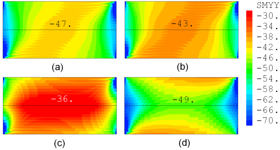
FIGURE 4.9 – Modélisation de la contrainte mécanique appliquée sur les câbles dans la direction y (transverse aux câbles), en MPa. Les pressions moyennes sont indiquées. (a) chargement mécanique. (b) chargement mécanique puis thermique. Le chargement magnétique est ajouté avec : (c) un champ extérieur parallèle de 9 T ou (d) un champ extérieur anti-parallèle de 9 T.
