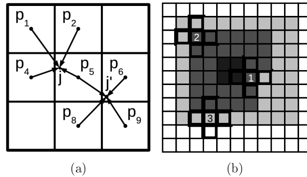
FIGURE 4.5 – (a) Calcul des centroïdes locaux par interpolation des moyennes de région les plus proches. (b) Modèle topologique. Du blanc au gris foncé, les labels sont 0, 1, 2 et 3, 0 étant le fond de l'image. Le voxel 1 ne peut pas changer de label car il y a plus de 3 labels différents dans son voisinage. Le voxel 2 peut changer de label. Le voxel 3 ne peut pas changer car le fond fait partie de son voisinage.
