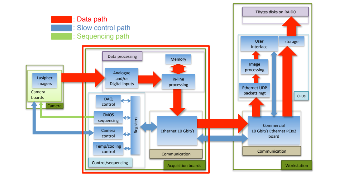
FIGURE II.15 – Schéma de principe du flux de données de l'acquisition 10 Gbits/s.
