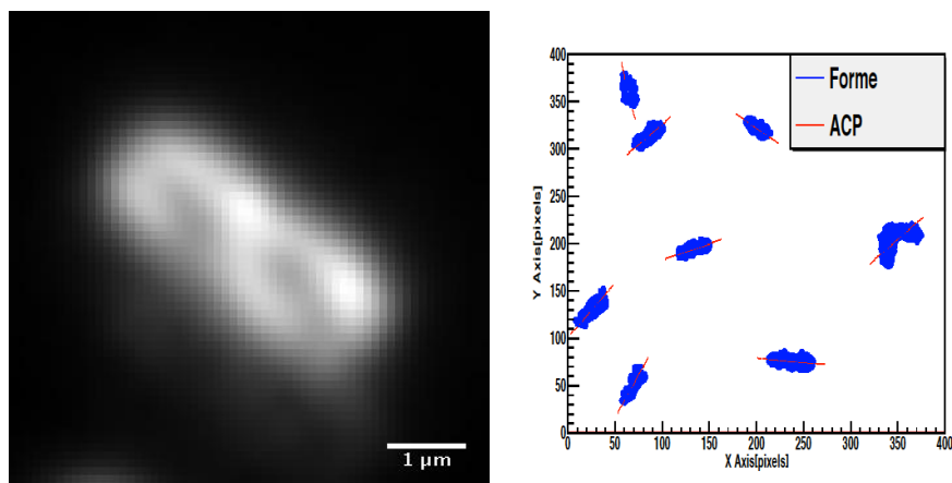
FIGURE II.22 – Image reconstruite d'une bactérie E. Coli à partir de 2500 images prises à 500 Hz au x100 (gauche). La figure de droite montre les axes principaux des bactéries obtenus par la méthode de la composante principale (matrice de covariance de la forme ou de la charge)
