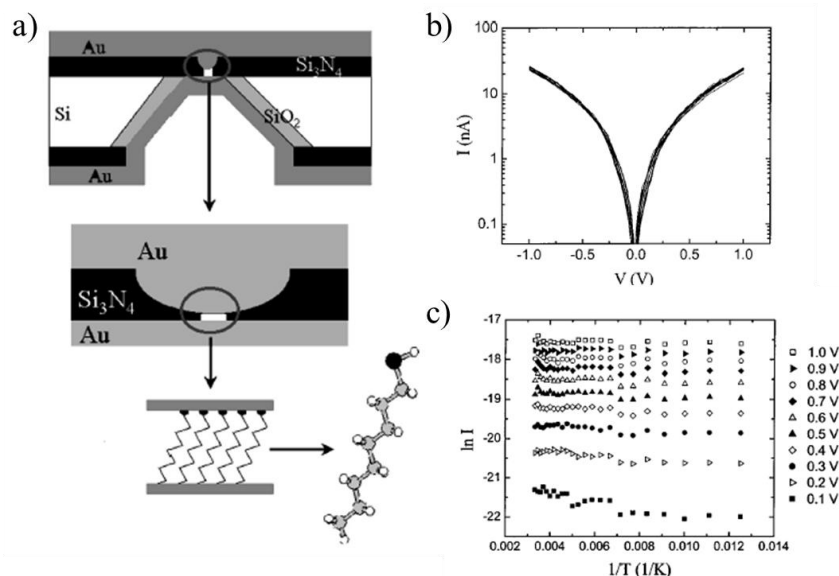
Figure 1.7 : a) Représentation schématique du dispositif étudié. b) Courbes I-V du dodecanethiol à différentes températures (de 300 à 80 K). c) Courbes d'Arrhénius issues des données obtenues en b) à des polarisations variant de 0,1 V à 1V avec des pas de 0,1 V. Figures reproduites d'après [2].
