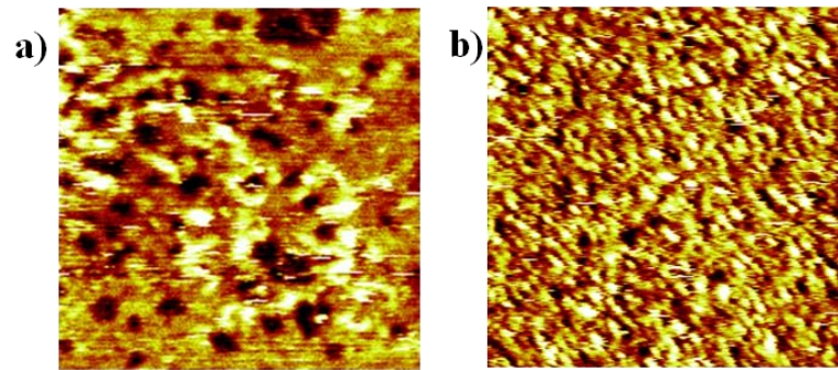
Figure E3 : b) Image STM de P3DTBr à 5.10^{-6} M dans du phényloctane ( I_T = 55 pA / V_T = +925 mV / 67 \times 67 nm 2 ) déposée sur une couche de C 11 COOHs. Quelques brins sont visibles au centre. c) Image typique d'une surface d'Au(111) avec C 11 COOHs, suite au dépôt de deux gouttes de P3DTBr à 5.10^{-6} M dans du phényloctane ( I_T = 95 pA / V_T = -1560 mV / 64 \times 64 nm 2 ).
