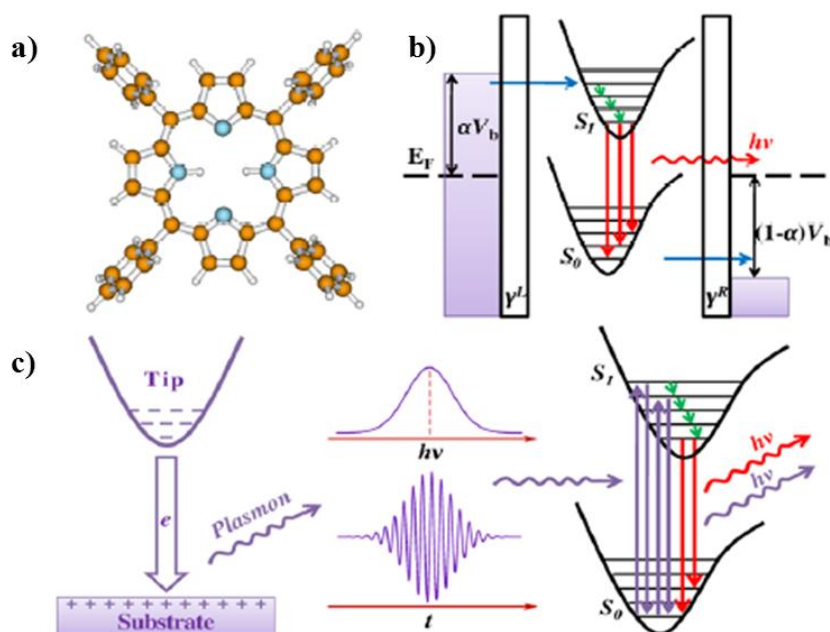
Figure 1.18 : a) Structure de la porphyrine étudiée, identique à celle présentée en Figure 1.15 a). b) Emission de photons provoquée par effet tunnel tenant compte de la relaxation interne. c) Procédé reposant sur les plasmons. Figures reproduites d'après [1].
