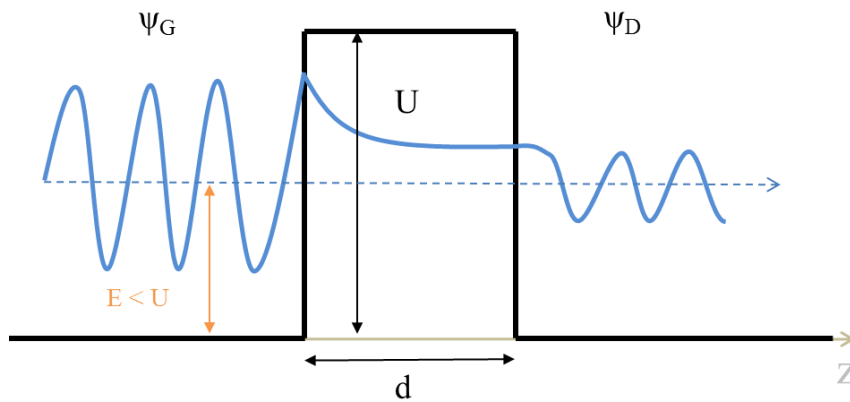
Figure 2.1 : Barrière de potentiel rectangulaire et unidimensionnelle.
