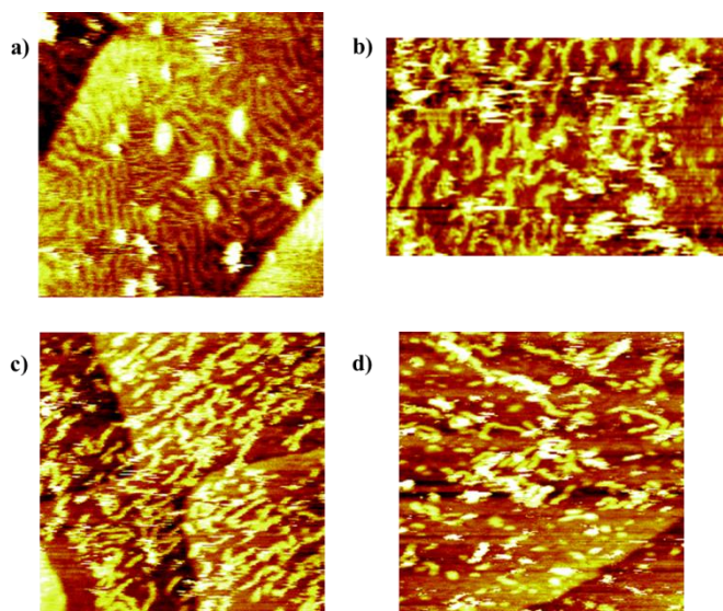
Figure 4.32 : Les P3ATBr sur Au (111). a) Image STM de P3DTBr à 5.10^{-6} M sur Au (111) montrant une première couche organisée ainsi que quelques « amas » plus clairs ( I_T = 70 pA, V_T = -1140 mV, 35 \times 35 nm 2 ). b) Image STM de P3DTBr à 5.10^{-5} M sur Au (111) montrant des brins de polymères qui ne semblent ni fixés ni organisés sur la surface ainsi que d'autres, plus élevés ( I_T = 15 pA, V_T = -990 mV, 120 \times 75 nm 2 ). c) Image STM de P3PDTBr à 5.10^{-6} M sur Au (111) montrant une première couche peu organisée ( I_T = 100 pA, V_T = -915 mV, 140 \times 140 nm 2 ). d) Image STM de P3PDTBr à 5.10^{-6} M sur Au (111) montrant des brins déposés sur la surface mais non organisés ainsi que le passage d'autres situés à une hauteur supérieure ( I_T = 125 pA, V_T = -770 mV, 85 \times 85 nm 2 ).
