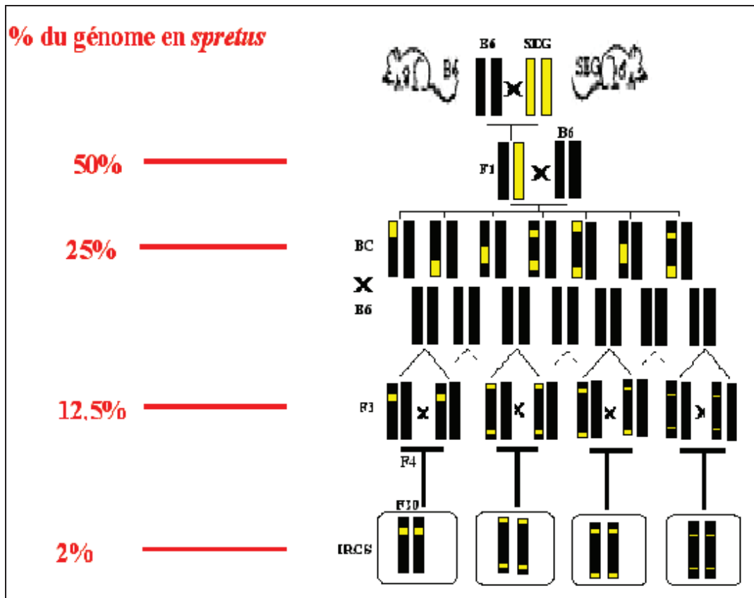
Figure 6 : Etablissement des lignées IRCS créées à l'institut Pasteur. Le premier croisement entre le lignées parentales B6 et SEG est suivi par deux backcross sur B6. Une vingtaine de croisements frère – sœur permettent de fixer le génome spretus à l'état homozygote dans un fond B6. Chacune des 55 lignées IRCS possède en moyenne 1,5% du génome spretus .
