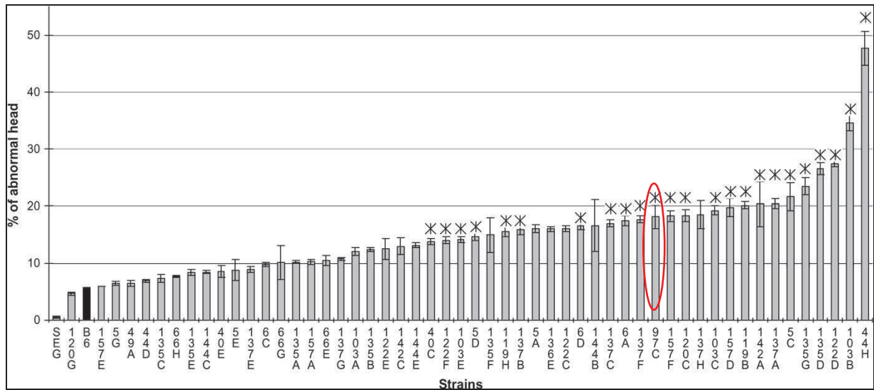
Figure 9: Fréquence d'anomalies de morphologie de la tête des spermatozoïdes. Les valeurs moyennes (+/- SEM) sont présentés et les astérisques (*) distinguent les 24 souches qui ont montré une augmentation significative des valeurs moyennes par rapport à B6.
