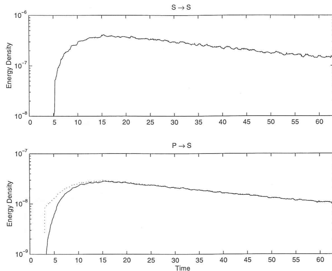
FIG. 4.17 - Densité d'énergie S correspondant à la réflexion d'ondes S incidentes (en haut), ou d'ondes P incidentes (en bas). La valeur prédite en négligeant l'anisotropie du champ incident est indiquée en pointillé; le trait plein correspond à la valeur obtenue en tenant compte de l'anisotropie.
