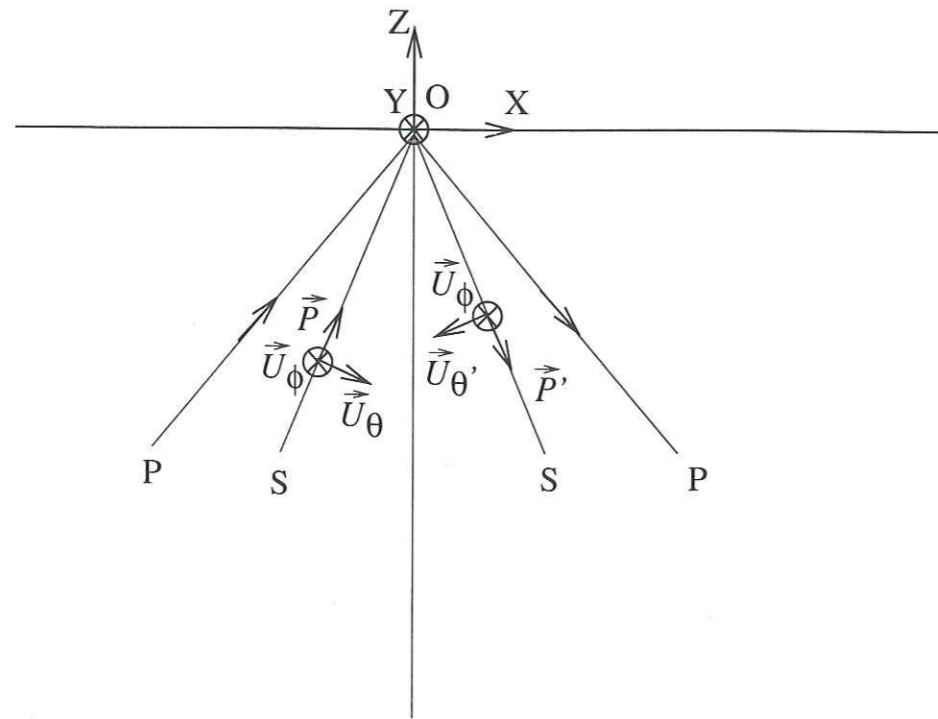
FIG. 4.12 – Conventions pour l'expression des vecteurs de Stokes incidents et réfléchis. Les conversions possibles sont également indiquées.
