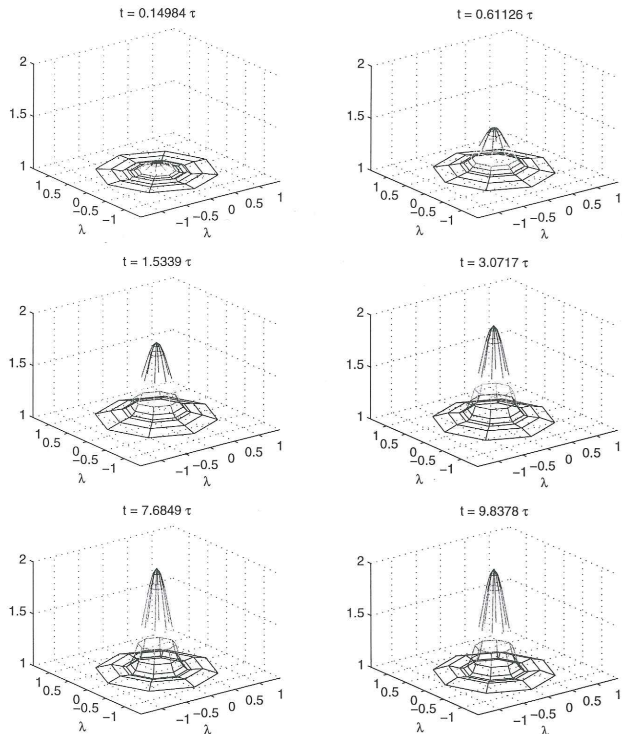
FIG. 6.3 – Evolution spatio-temporelle du cône de rétrodiffusion. Sur l'axe vertical: (I_{coh} + I_{inc})/I_{coh} ; axes horizontaux: distance par rapport à la source exprimée en longueur d'onde. Le temps est exprimé en fonction du temps libre moyen au-dessus de chaque figure.
