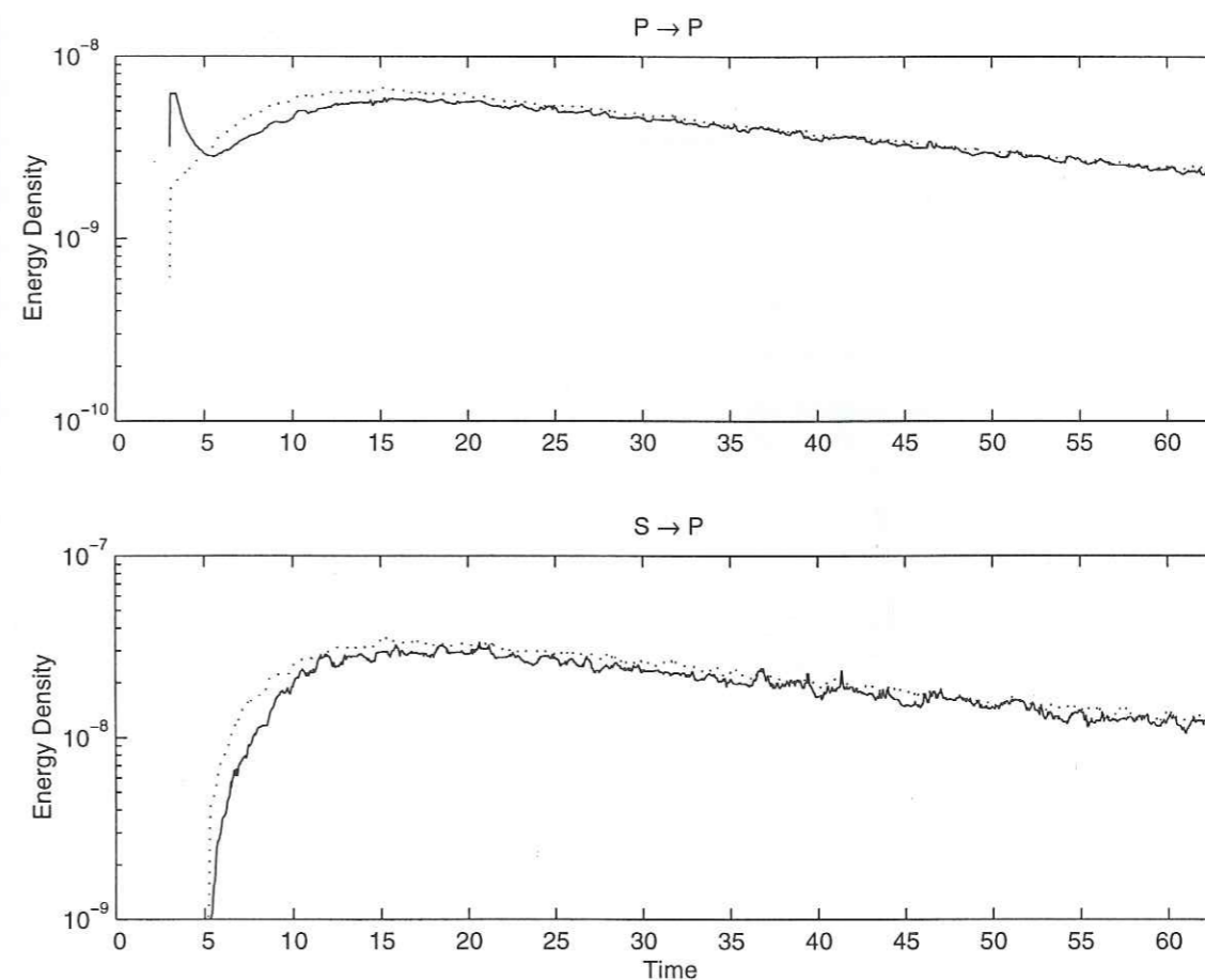
FIG. 4.16 – Densité d'énergie P correspondant à la réflexion d'ondes P incidentes (en haut), ou d'ondes S incidentes (en bas). La valeur prédite en négligeant l'anisotropie du champ incident est indiquée en pointillé; le trait plein correspond à la valeur obtenue en tenant compte de l'anisotropie.
