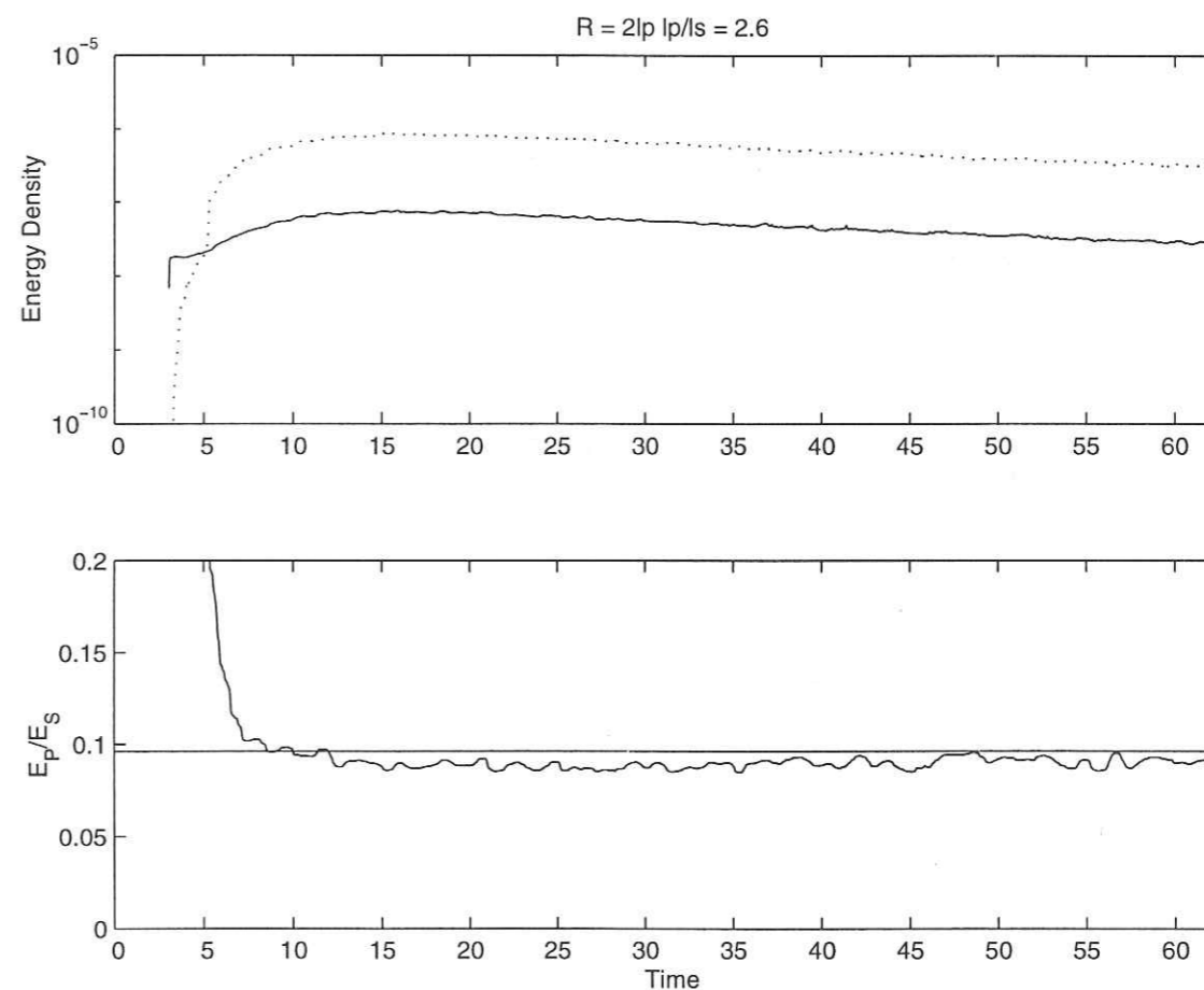
FIG. 4.15 – Résultat de la simulation Monte-Carlo pour une source d'ondes S et un détecteur situés au voisinage de la surface. La distance source-station R ainsi que le rapport l_P/l_S sont indiqués sur la figure. En abscisse, l'unité de temps est le temps libre moyen des ondes S. En haut, évolution temporelle de la densité d'énergie des ondes P (trait plein) et des ondes S (pointillé). En bas, évolution du rapport des densités d'énergie E_P/E_S . La valeur "théorique" du rapport d'énergie est indiquée.
