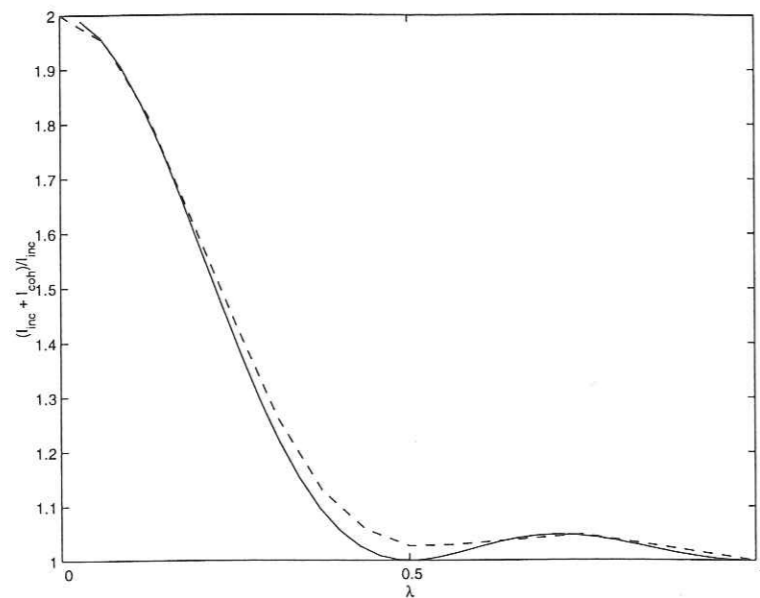
FIG. 6.5 – Comparaison entre la forme du cône obtenue par simulation Monte-Carlo (pointillé) après 15 temps libres moyens et la prédiction asymptotique analytique. La distance par rapport à la source est exprimée en abscisse en fonction de la longueur d'onde
