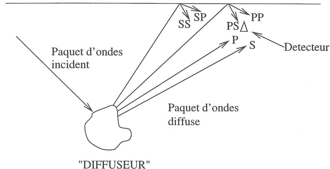
FIG. 4.14 - Représentation schématique des différentes probabilités pour l'énergie d'atteindre le détecteur.
