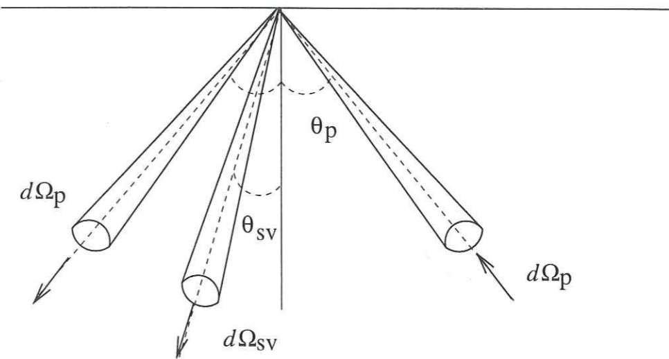
FIG. 4.13 – Modification de l'angle solide d'un faisceau d'énergie P lors de la réflexion à la surface
