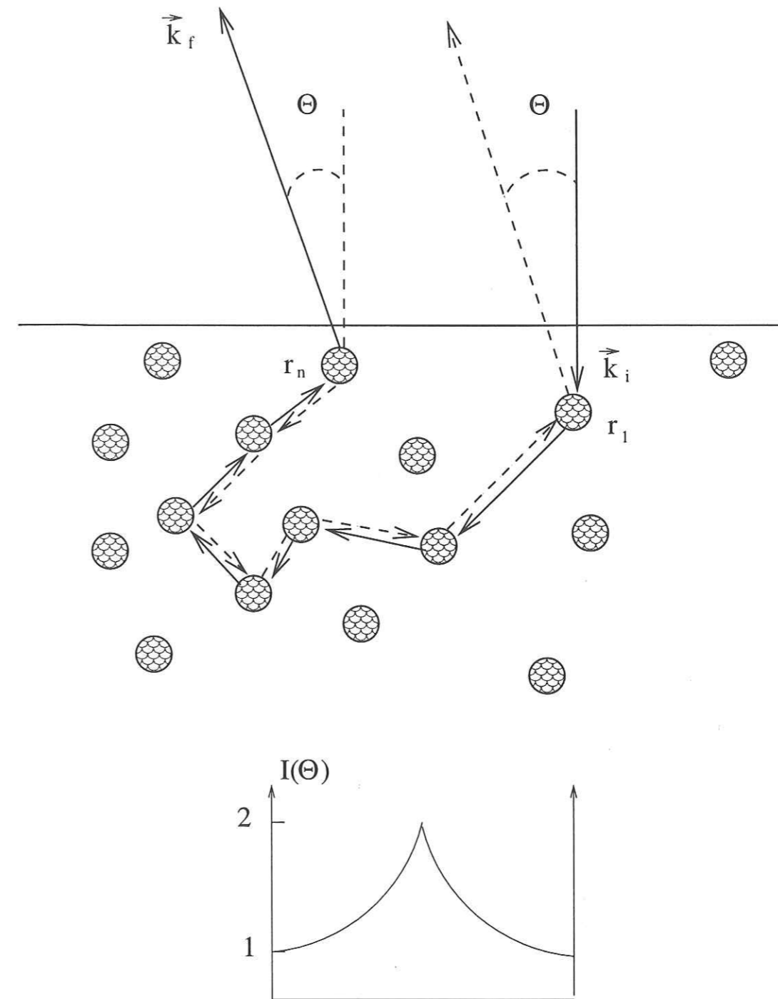
FIG. 6.1 – Situation typique pour l'observation du cône. Une onde collimatée (et approximativement plane) est envoyée sur un échantillon contenant des diffuseurs. On mesure l'intensité rétrodiffusée par l'échantillon en champ lointain en fonction de l'angle \Theta mesuré par rapport à la direction d'incidence. L'intensité mesurée autour de la direction incidente présente un facteur d'amplification par rapport au niveau de base (ici normalisé à 1). Idéalement, le facteur d'amplification vaut 2.
