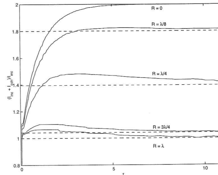
FIG. 6.4 – Comparaison entre les solutions numériques et analytiques à différentes distances R entre source et récepteur, exprimées en nombre de longueur d'onde. La solution numérique (en pointillé) évolue asymptotiquement vers la valeur prédite par la solution analytique (trait plein).
