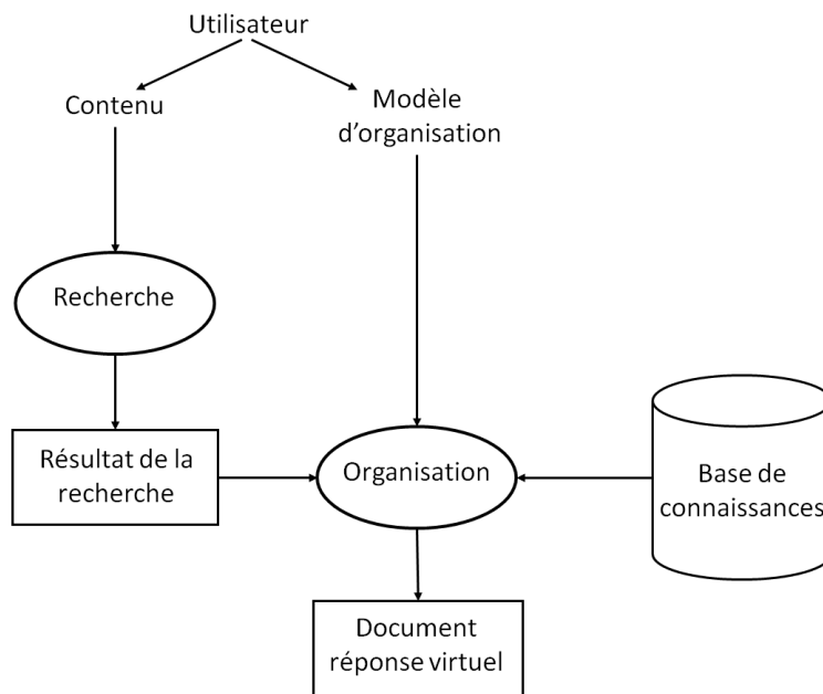
FIG. 2.1 – Génération d'un document réponse virtuel.
