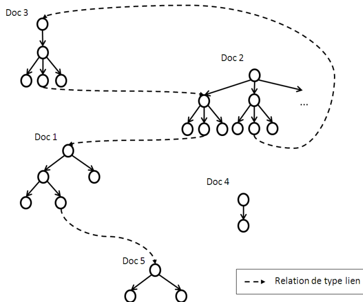
FIG. 3.3 – Relation non-compositionnelle entre doxels de \mathcal{C}^{exemple} .
