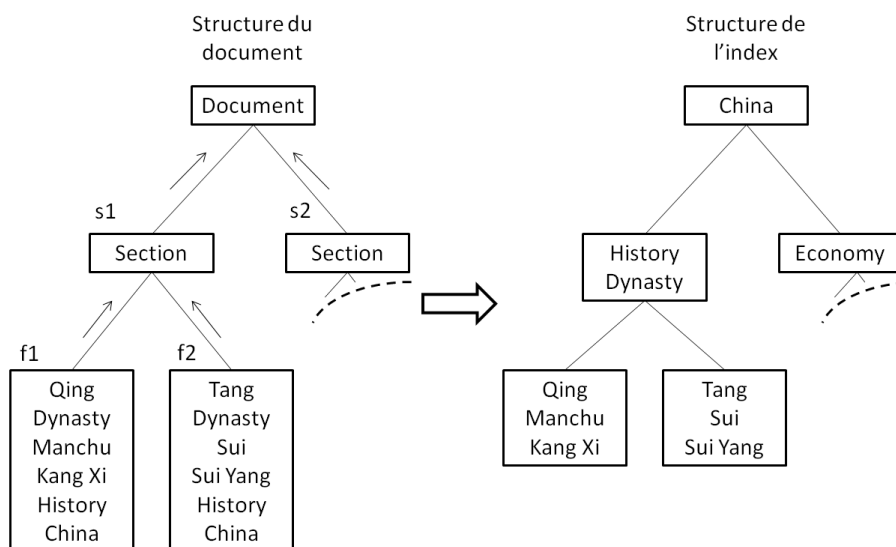
FIG. 1.2 – Propagation de l'index et mécanisme d'élagage [CWC03].
