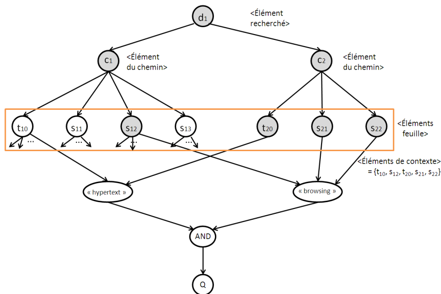
FIG. 1.4 – Un réseau d'inférence pour un document structuré et une requête [MJKZ98].
