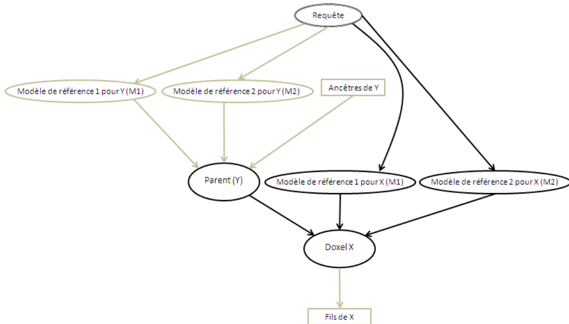
FIG. 1.5 – Vue locale d’un réseau Bayésien s’appuyant localement sur 2 modèles de recherche d’information M_1 et M_2 [PG04].
