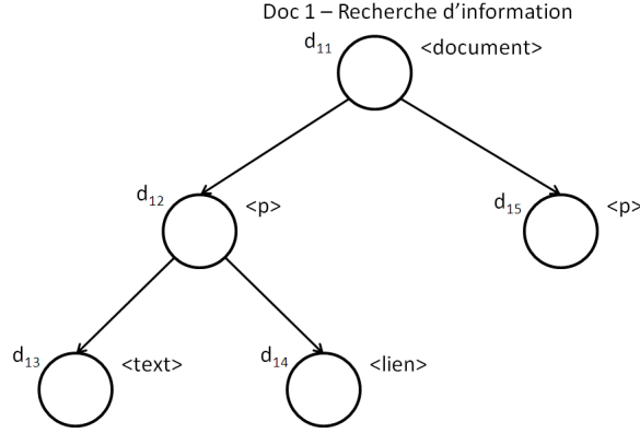
FIG. 3.2 – Représentation du document 1 de \mathcal{C}^{exemple} sous forme d'arbre.
