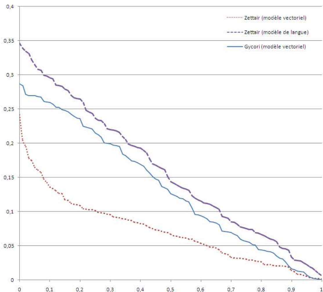
FIG. 8.4 – Comparaison de notre système avec Zettair (INEX 2007).
