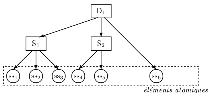
FIG. 1 – Exemple de représentation d'un document structuré (structuration explicite).
