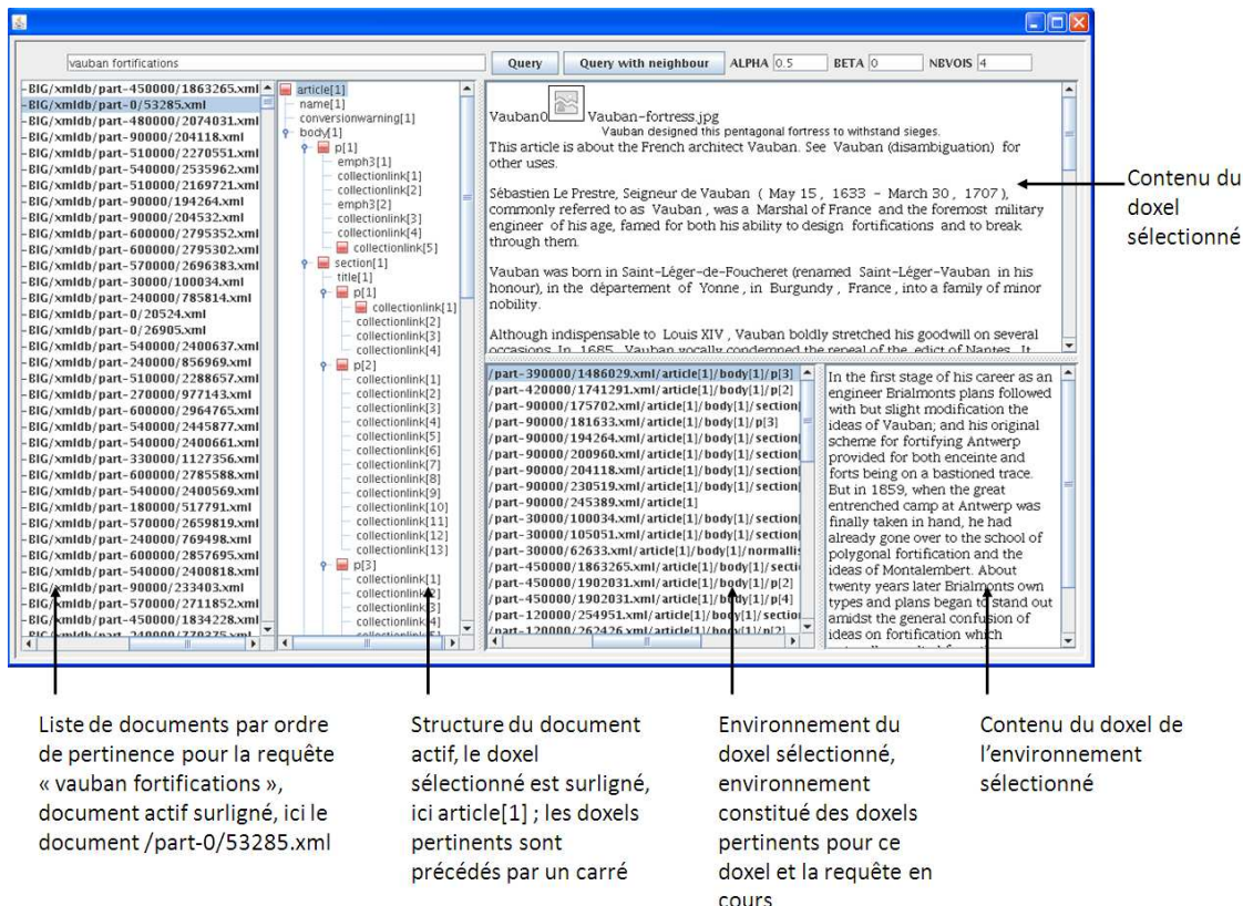
FIG. 5.1 – Exemple de présentation à l'écran.
