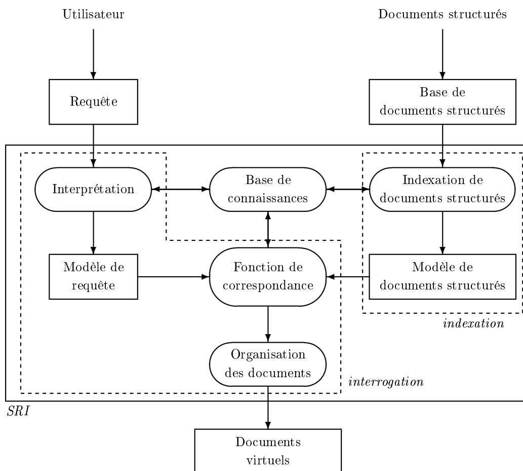
FIG. 4 – Système de recherche d'information pour des documents virtuels.
