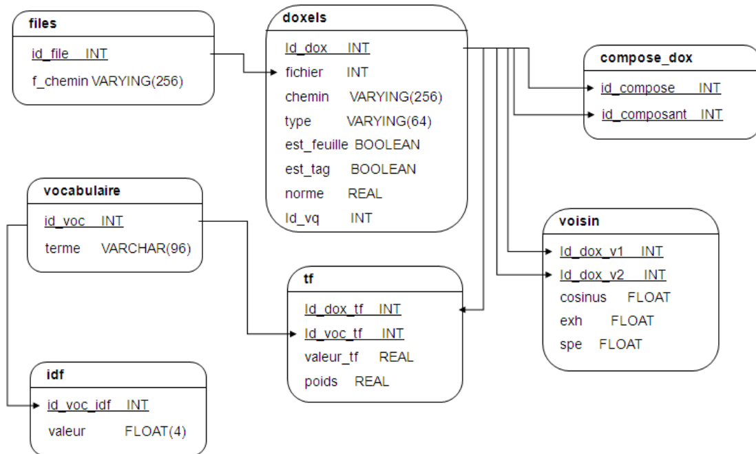
FIG. 8.3 – Schéma de la base de données
