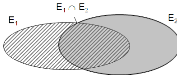
FIG. 6.2 – Deux ensembles E_1 et E_2 et leur intersection.
