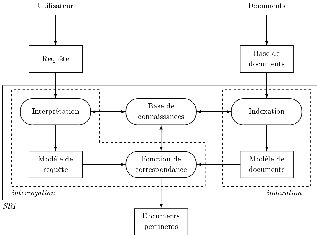
FIG. 3 – Architecture d'un système de recherche d'information.
