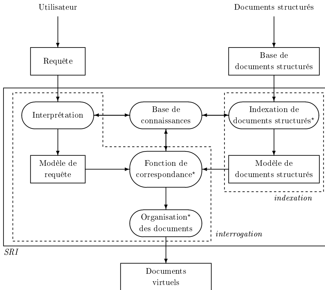
FIG. 3 – Système de recherche d'information pour des documents virtuels.
