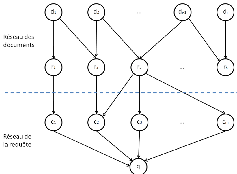
FIG. 1.3 – Un exemple de réseau d'inférence simple pour la recherche de documents [CCH92].
