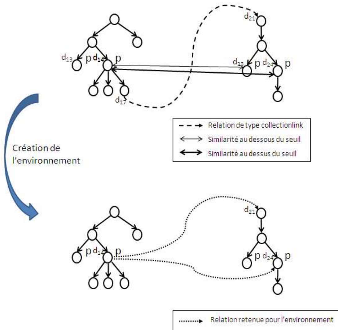
FIG. 8.1 – Création de l'environnement à partir d'un lien collectionlink .
