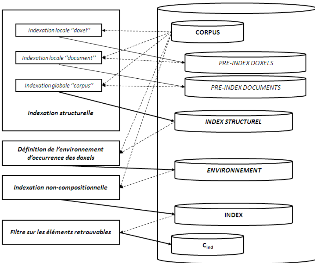
FIG. 4.1 – Modèle d'indexation de documents structurés.
