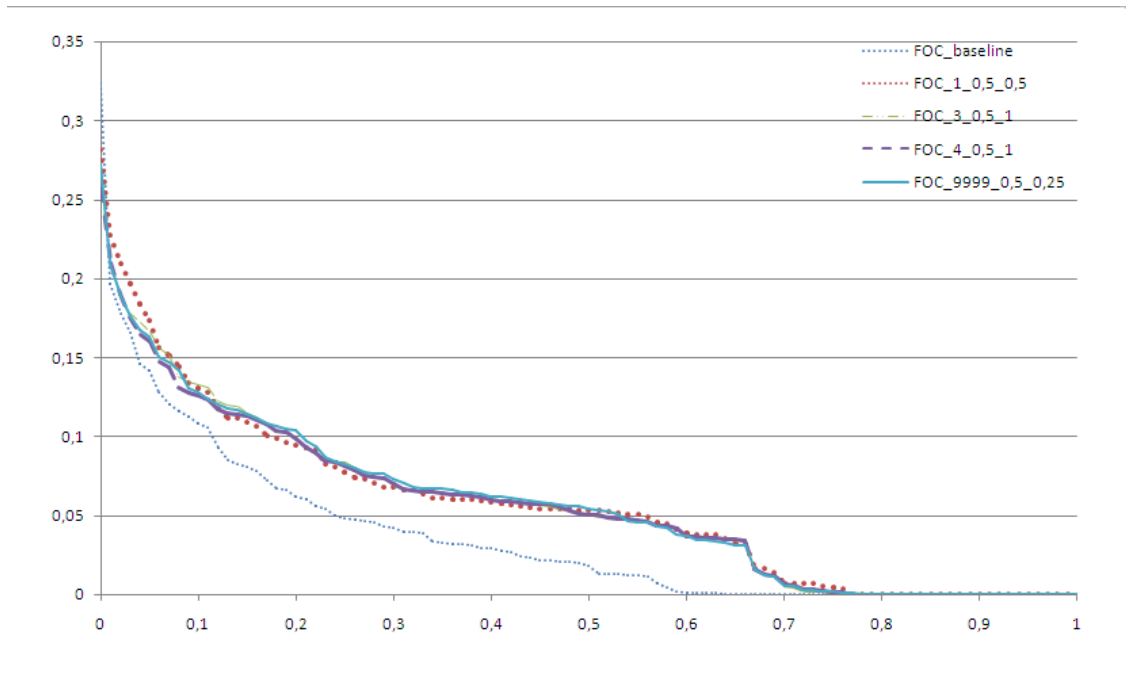
FIG. 8.5 – Courbe avec prise en compte du voisinage - liens sortants (type FOC_1 ).
