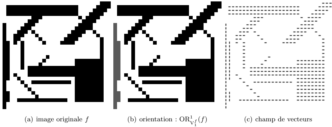
FIGURE 9.3 – Critère d'orientation à VAG \text{OR}_{V_1^f}^1(f) (b) de l'image originale f (a) et sa représentation par champ de vecteurs (c). Le ton de gris de chaque point x de la cartographie (b) représente son orientation locale. ■ \equiv 1 pixel.
