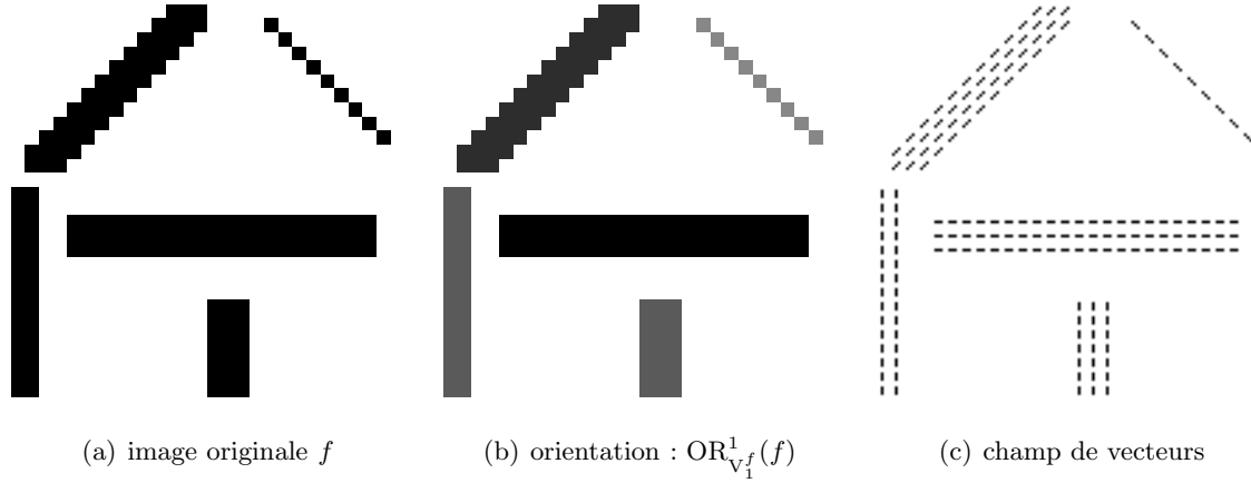
FIGURE 9.2 – Critère d'orientation à VAG \text{OR}_{V_1^f}^1(f) (b) de l'image originale f (a) et sa représentation par champ de vecteurs (c). Sur la cartographie d'orientation (b) \text{OR}_{V_1^f}^1(f) , le ton de gris de chaque point, représentant son orientation locale (en degrés), est associée à un vecteur (c). Les VAG sont calculés selon le modèle CLIP. L'icône ■ représente un pixel.
