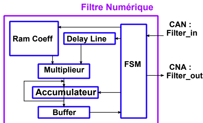
FIG. 5.2 – Schéma de principe du filtre FIR
