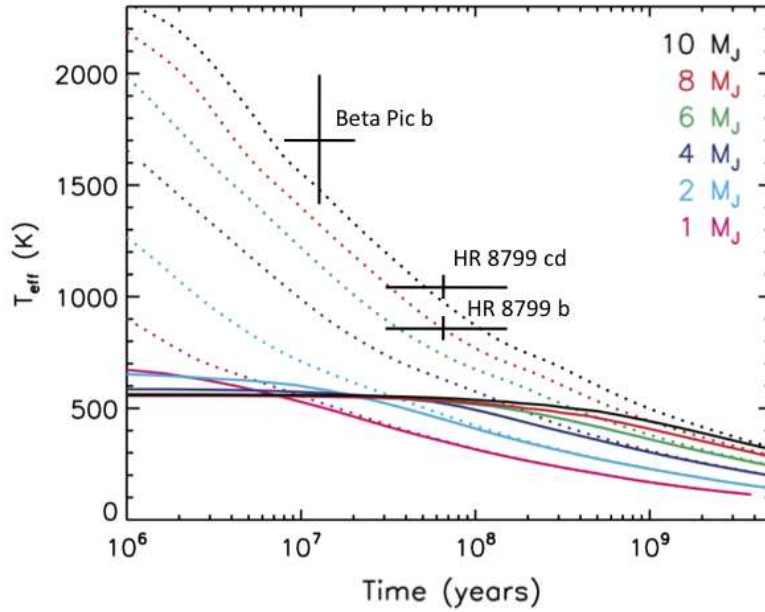
FIGURE I.2.9 – Diagramme d'évolution de la température effective de planètes géantes gazeuses. Les courbes en pointillés correspondent au modèle d'évolution sans prise en compte de la formation par accretion alors que les courbes en trait plein correspondent au modèle avec prise en compte de l'accretion. Le code couleur définit la masse de la planète et est indiqué dans la figure. J'ai placé sur ce graphique les planètes \beta Pictoris b ( T_{\text{eff}} = 1700 \pm 300 K, âge = 12_{-4}^{+8} Ma, Bonnefoy et al. 2011) et HR 8799 bcd ( T_{\text{eff}} = 800\text{--}900 , 1000\text{--}1100 et 1000\text{--}1100 K, âge = 60_{-30}^{+100} Ma, Marois et al. 2008b). Figure modifiée de Marley et al. (2007).
