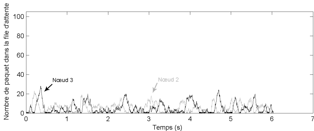
FIGURE 4.30 – Evolution des files d’attente des nœuds 2 et 3 avec un flux 1-6 avec régulateur de trafic optimisé
