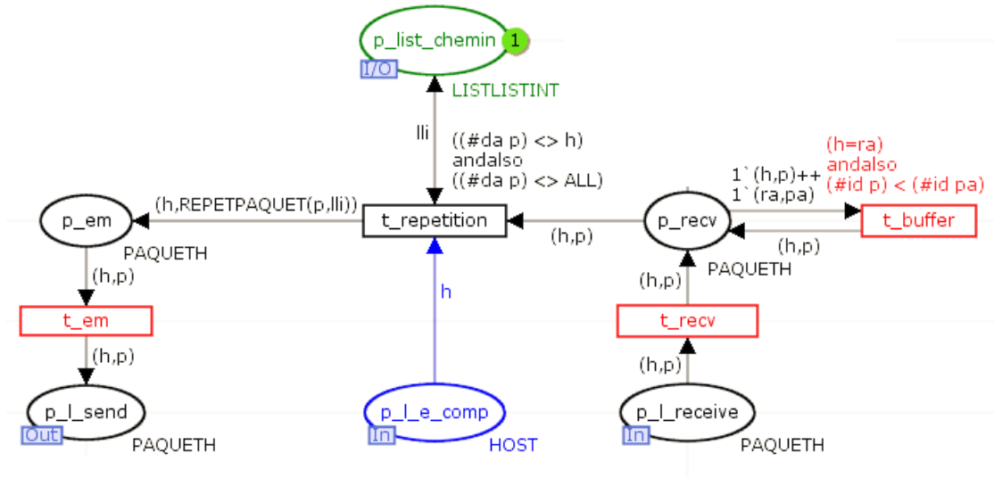
FIGURE 3.56 – Modèle LLC - 2 ème étape - Répétition de paquet
