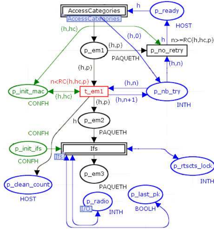
FIGURE 3.29 – Modèle MAC - 3 ème étape - décompte du temps interframe
