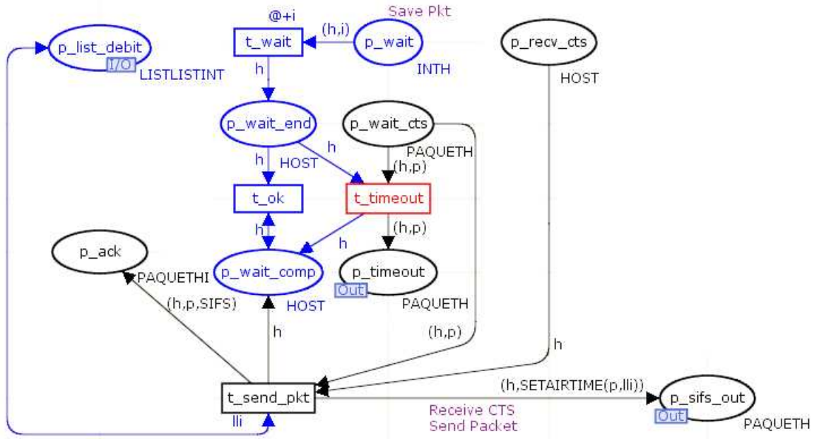
FIGURE 3.41 – Modèle ACKRTSCTS - 3 ème étape - Attente de CTS
