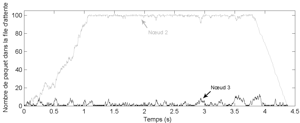
FIGURE 4.15 – Evolution des files d'attente des nœuds 2 et 3 avec un flux 1-4 et modification du paramètre CW_{min} sur le nœud source
