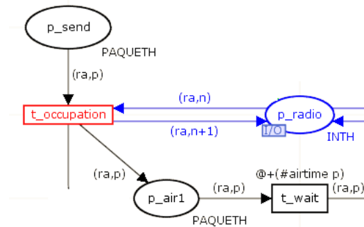
FIGURE 3.17 – Modèle Radio - 3 ème étape - temporisation et occupation du médium
