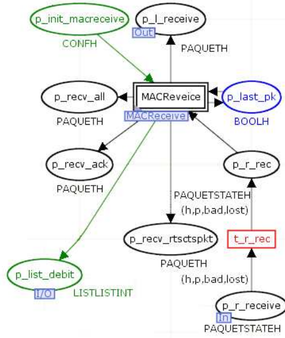
FIGURE 3.45 – Modèle MAC - 6 ème étape - Réception de paquet
