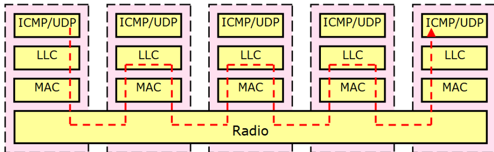
FIGURE 3.10 – Transmission sur chaque nœud
