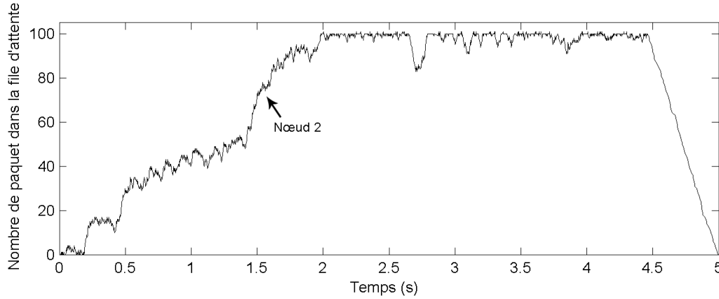
FIGURE 4.9 – Evolution de la file d'attente du nœud 2 avec un flux 1-4 et modification du paramètre AIFS sur le nœud source
