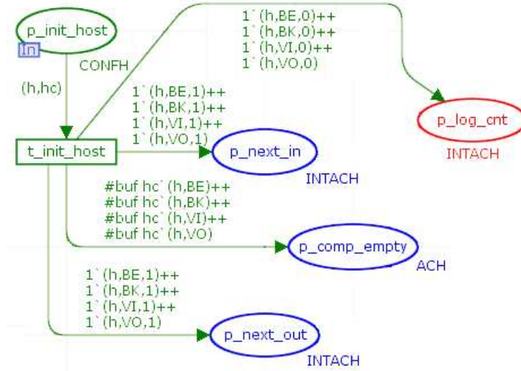
FIGURE 3.25 – Modèle AccessCategories - 1 ère étape - initialisation du modèle
