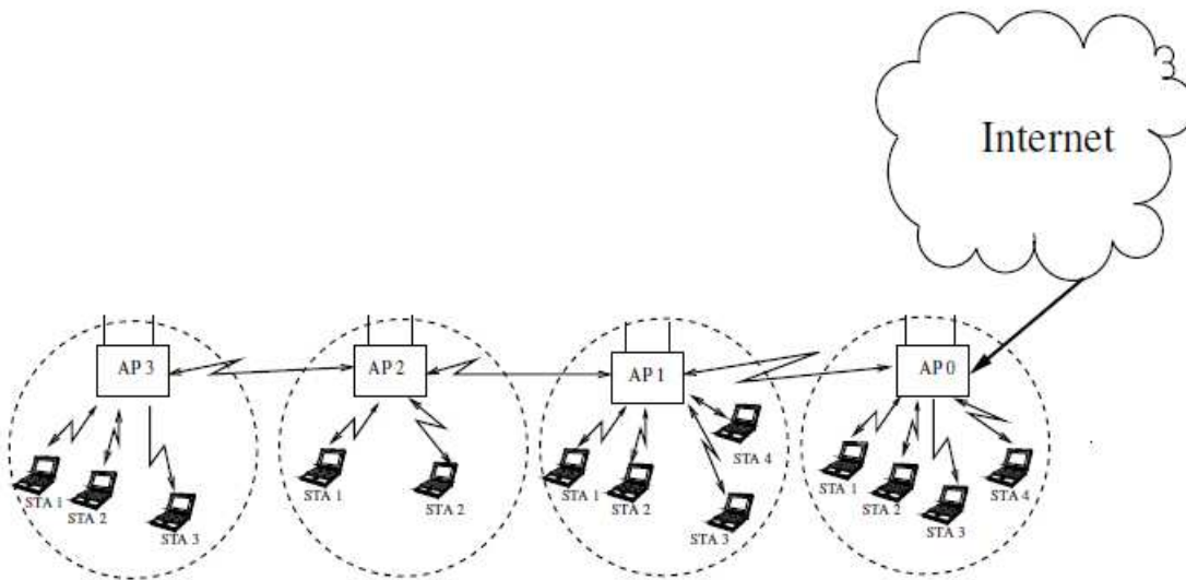
FIGURE 2.1 – Topologie présentant quatres nœuds alignés
