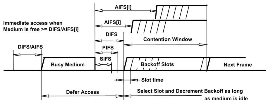
FIGURE 1.7 – Différents délais interframes présentés dans la norme [IEE99a]
