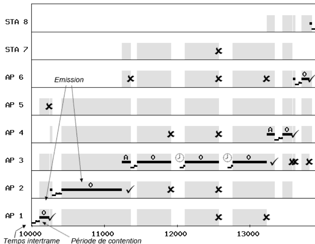
FIGURE 3.69 – Première partie du graphique généré lors d'un échange ICMP
