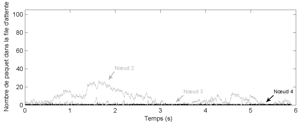
FIGURE 4.23 – Evolution des files d'attente des nœuds 2, 3 et 4 avec un flux 1-6 et modification du paramètre AIFS sur les nœud 1 et 2
