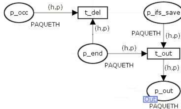
FIGURE 3.32 – Modèle Ifs - 3 ème étape - sortie du paquet
