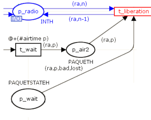
FIGURE 3.19 – Modèle Radio - 5 ème étape - libération du canal radio
