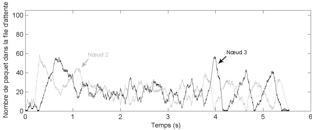
FIGURE 4.26 – Evolution des files d’attente des nœud 2 et 3 avec un flux 1-4 et régulateur de trafic
