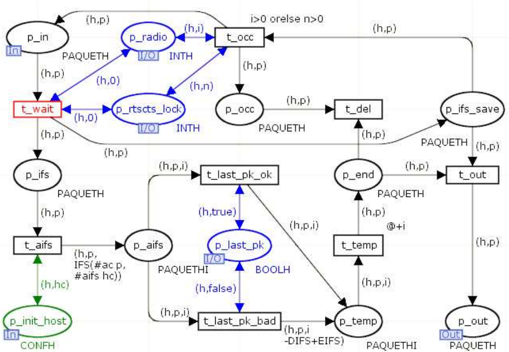
FIGURE 3.33 – Modèle Iifs complet
