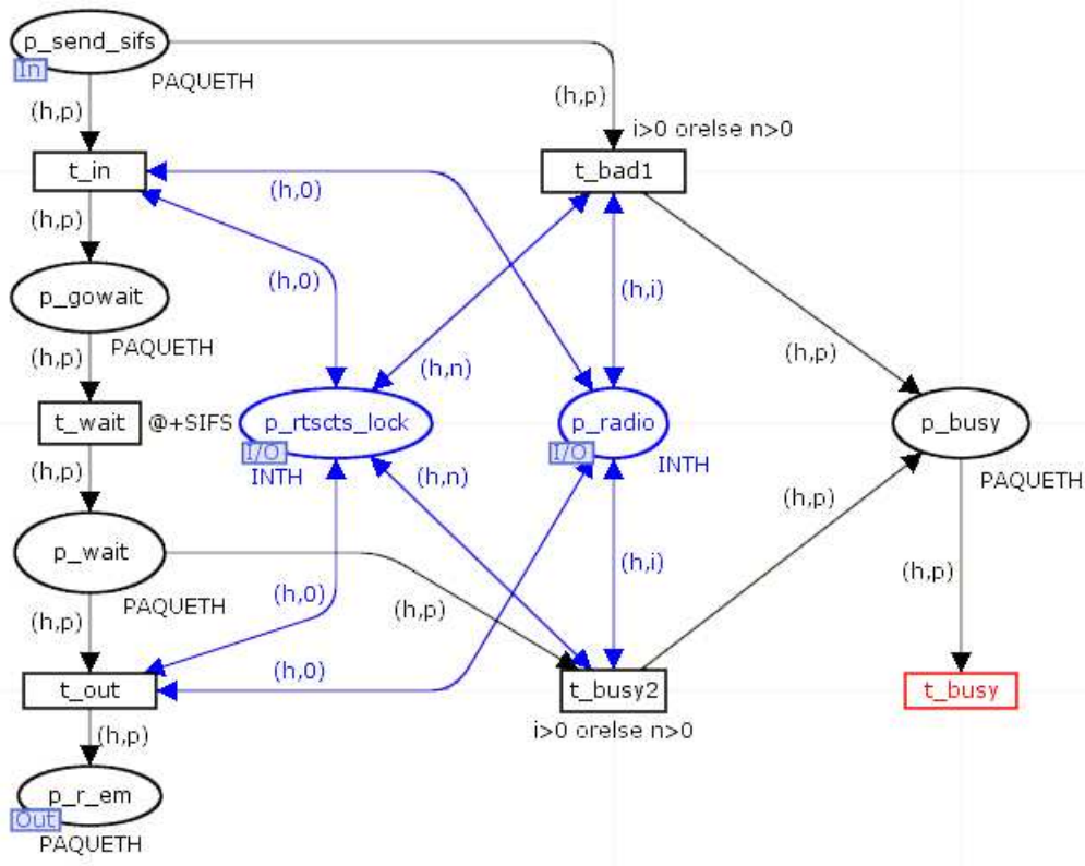
FIGURE 3.44 – Modèle SendWithSIFS
