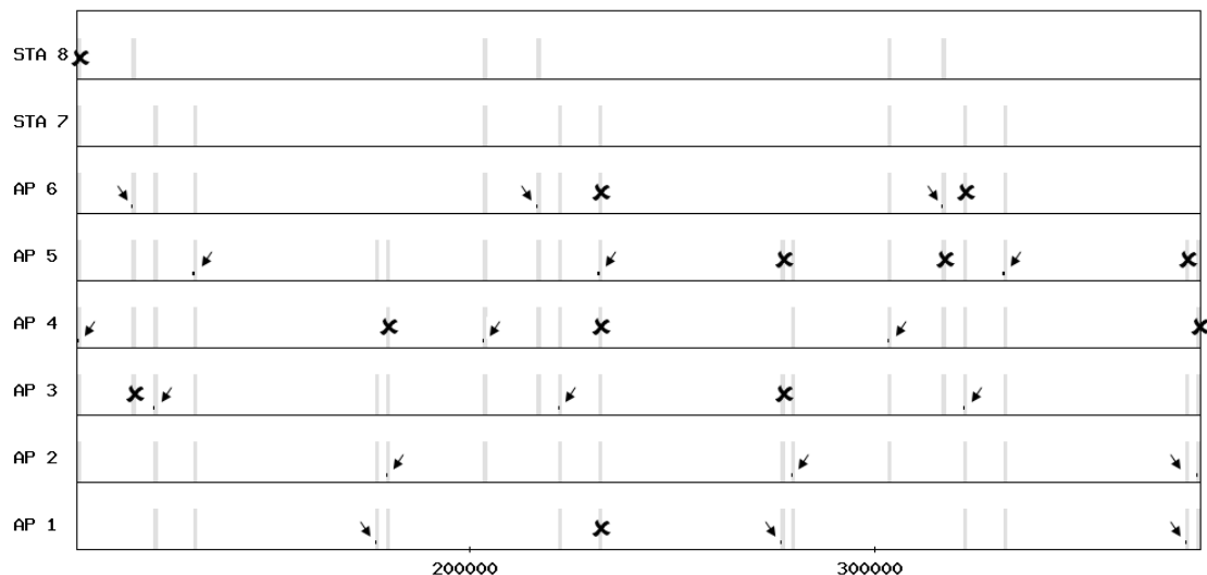
FIGURE 3.75 – Graphe généré lors d’une simulation de beacon
