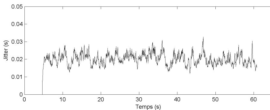
FIGURE 1.20 – Gigue sans WMM avec 1 RTP et 2 HTTP
