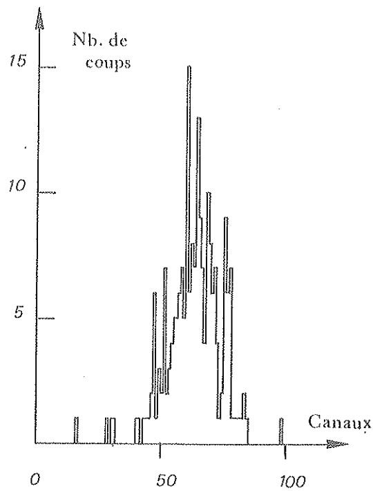
Figure 4 b - Spectre en localisation L/E sur 128 canaux . Ces spectres ont été tracés lors de l'étude de la réaction ^{16}\text{O}(d, ^6\text{Li})^{12}\text{C}^* 4.43 MeV sur une cible de \text{V}_2\text{O}_5 .
