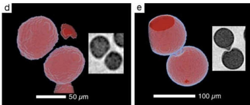
Figure 3.8: Coalescence des bulles dans un magma visqueux, par tomographie 3D. Gauche : planaire. Droite : champignon.
