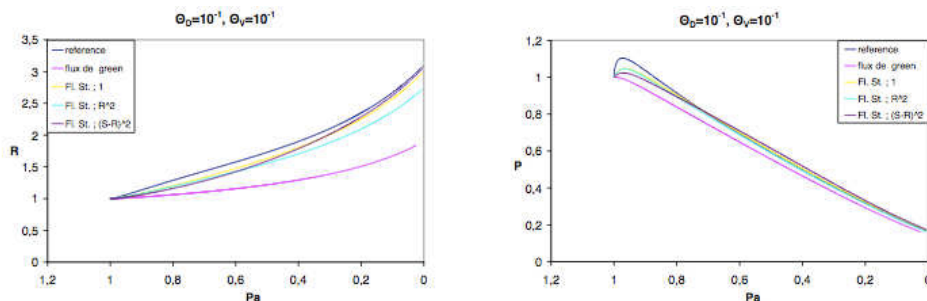
Figure 3.6: Comparaison flux système couplé et système simplifié pour \Theta_D = \Theta_V = 10^{-1} . Le rayon en fonction de P_a (gauche), la pression en fonction de P_a (droite).
