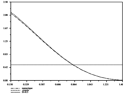
Figure 1.1: Coefficient de diffusion par rapport à \theta
