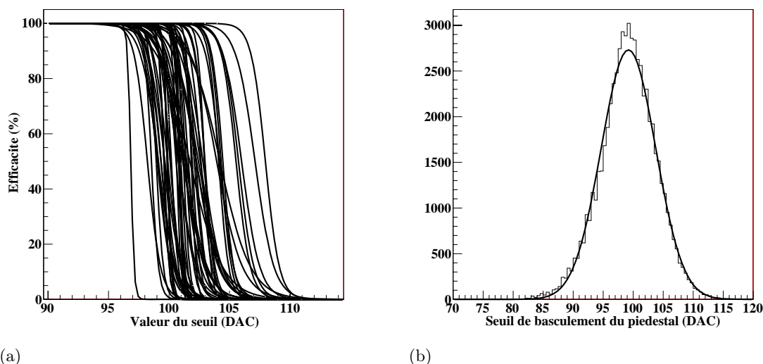
FIGURE 4.12 – (a) : Ajustement des courbes de piédestaux pour les 64 voies d'un HARDROC. (b) : Distribution du seuil de basculements des piédestaux, pour 64000 canaux.
