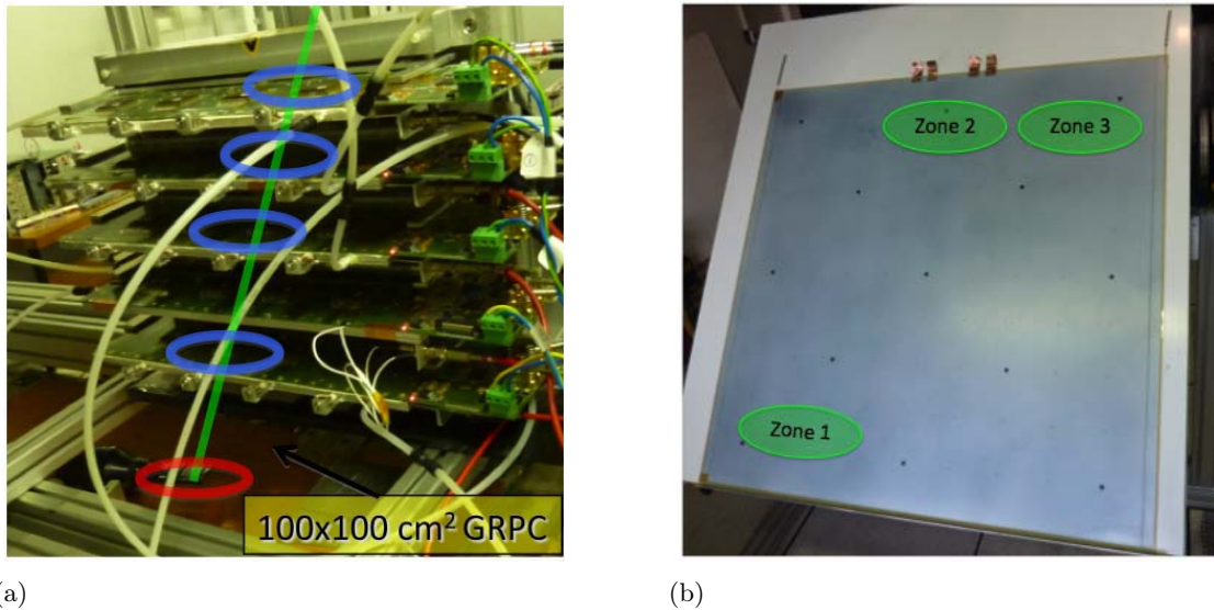
FIGURE 5.30 – (a) : Banc de test cosmique pour un détecteur de 1 \text{ m}^2 . (b) : Zones du détecteur testées.
