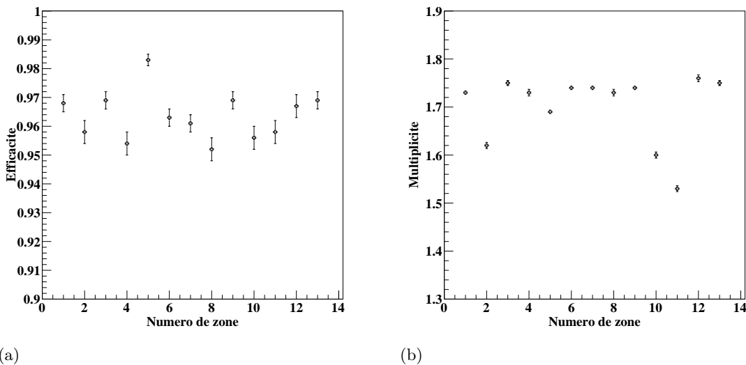
FIGURE 5.33 – Efficacité (a) et multiplicité (b) pour les 13 zones à l'étude.
