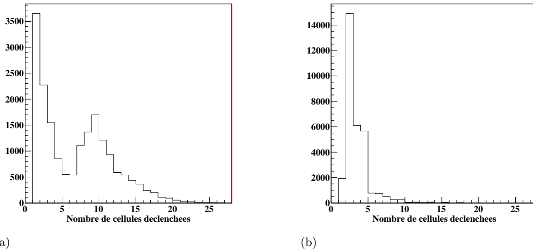
FIGURE 5.14 – Distribution du nombre de cellules déclenchées ( pad ) lors du passage d'un MIP pour deux compositions de gaz \text{TFE} , \text{CO}_2 , \text{SF}_6 : 95 %, 5 %, 0 % (a), et 94.5 %, 5 %, 0.5 % (b). La tension de polarisation appliquée est de 7.1 kV.
