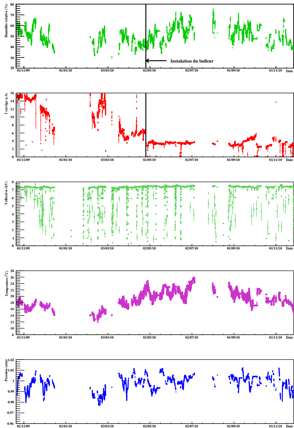
FIGURE 5.38 – Variations d’humidité relative, de courant corrigé, de tension effective, de température, et de pression, en fonction du temps d’exposition d’un détecteur GRPC de 1 \text{ m}^2 à la source radioactive du GIF.
