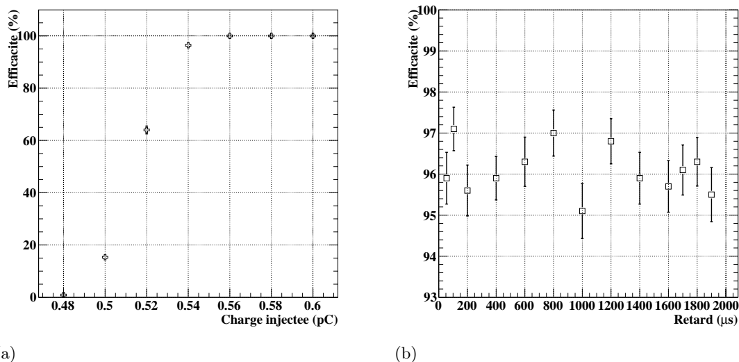
FIGURE 6.18 – (a) : Efficacité en fonction de la charge injectée (seuil : 140 DAC). (b) : Efficacité en fonction du retard entre alimentation et acquisition (Charge : 0.54 pC, seuil : 140 DAC).
