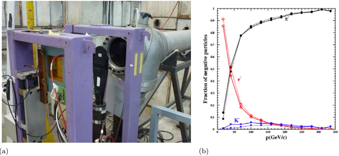
FIGURE 5.5 – (a) : Arrivée de la ligne secondaire dans la zone expérimentale. De gauche à droite : la chambre à fils (jaune), les scintillateurs (en partie occultés), le détecteur Cherenkov (tête de détection, et tube). (b) : Composition du faisceau secondaire sur la ligne H4 du SPS (North Area CERN).
