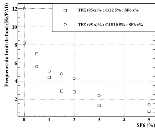
FIGURE 5.15 – Fréquence du bruit de fond en fonction de la proportion de \text{SF}_6 présente dans le mélange, (Seuil : \text{DAC} = 200 ).
