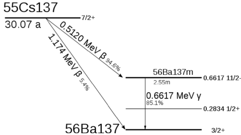
FIGURE 5.7 – Diagramme de désintégration du césium 137.
