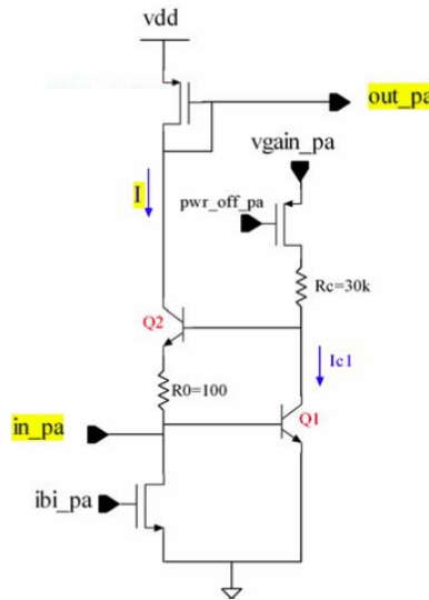
FIGURE 4.2 – Schéma de l'étage de préamplification du HARDROC.
