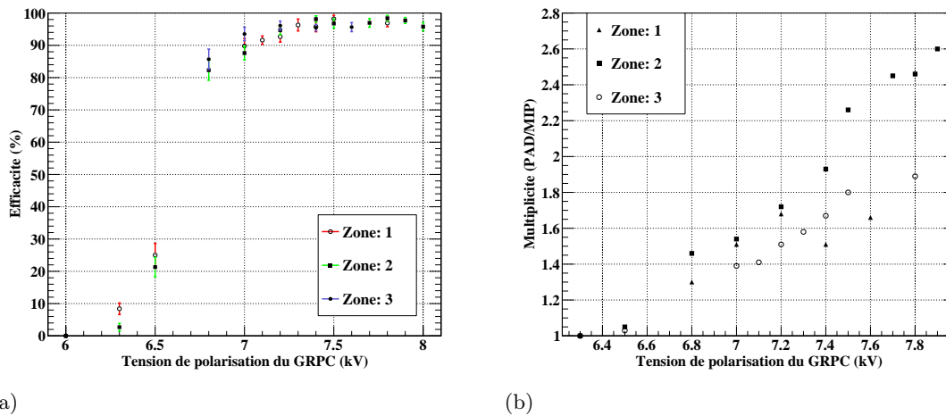
FIGURE 5.31 – (a) : Efficacité en fonction de la haute tension appliquée sur les trois zones étudiées. (b) : Multiplicité en fonction de la haute tension appliquée sur les trois zones étudiées.
