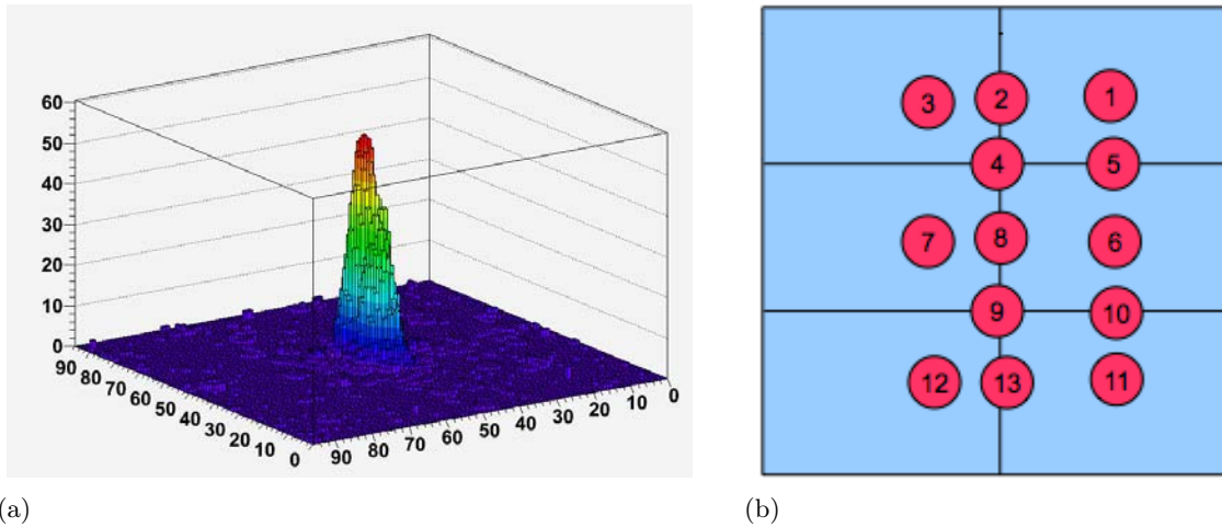
FIGURE 5.32 – (a) : Profil du faisceau obtenu dans notre GRPC de 1 \text{ m}^2 sur la ligne H4 du CERN ( 50 \text{ Hz/cm}^2 ). (b) : Zones étudiées sur les deux grands détecteurs.
