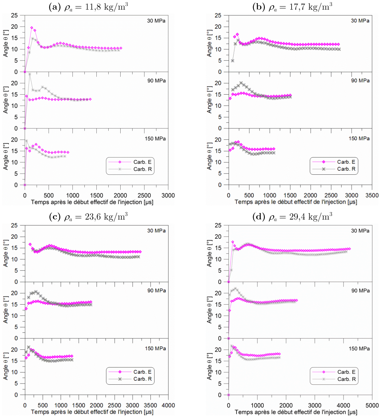
FIG. 4.14 : Évolution temporelle de l'angle du spray – Influence de la viscosité - P_i = 30 à 150 MPa, \rho_a = 11,8 à 29,4 kg/m 3 , T_a = 297 K, t_i = 4000 \mu s
