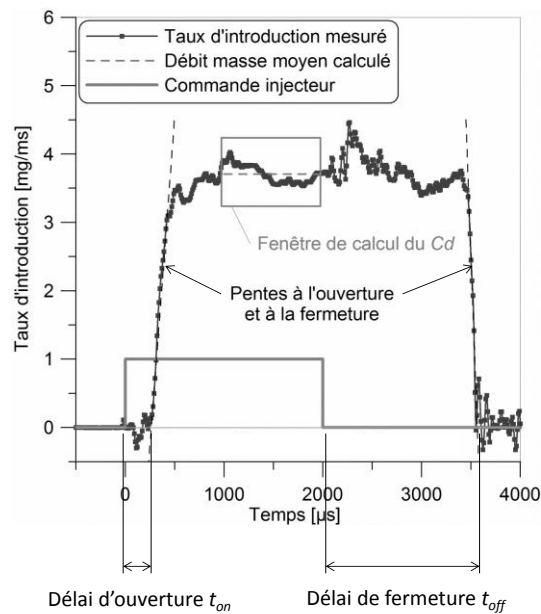
FIG. 2.3 : Principe de détection de l'instant d'ouverture et de fermeture de l'injecteur et fenètre de calcul du coefficient de décharge
