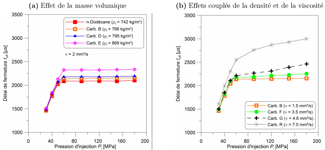
FIG. 3.5 : Influence de la densité (a) et du couplage densité/viscosité (b) sur le délai de fermeture – t_i = 2000 \mu s
