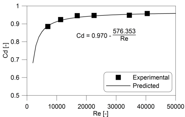
FIG. 1.9 : Évolution du coefficient de décharge en fonction du nombre de Reynolds [Payri et al. , 2008]
