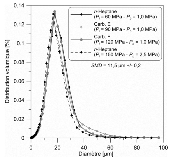
FIG. 5.14 : Distribution granulométrique à iso- SMD pour différents carburants et conditions
