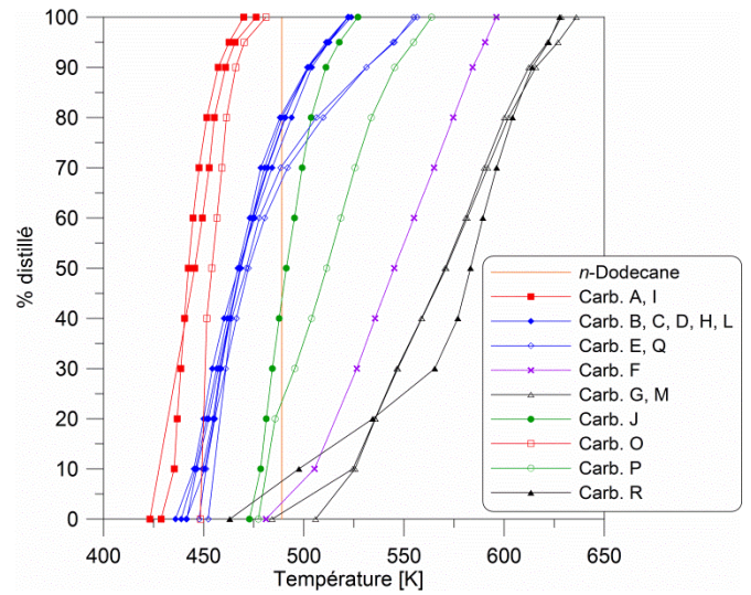
FIG. 2.46 : Courbes de distillation à P_{atm} des carburants de la matrice mesurés
