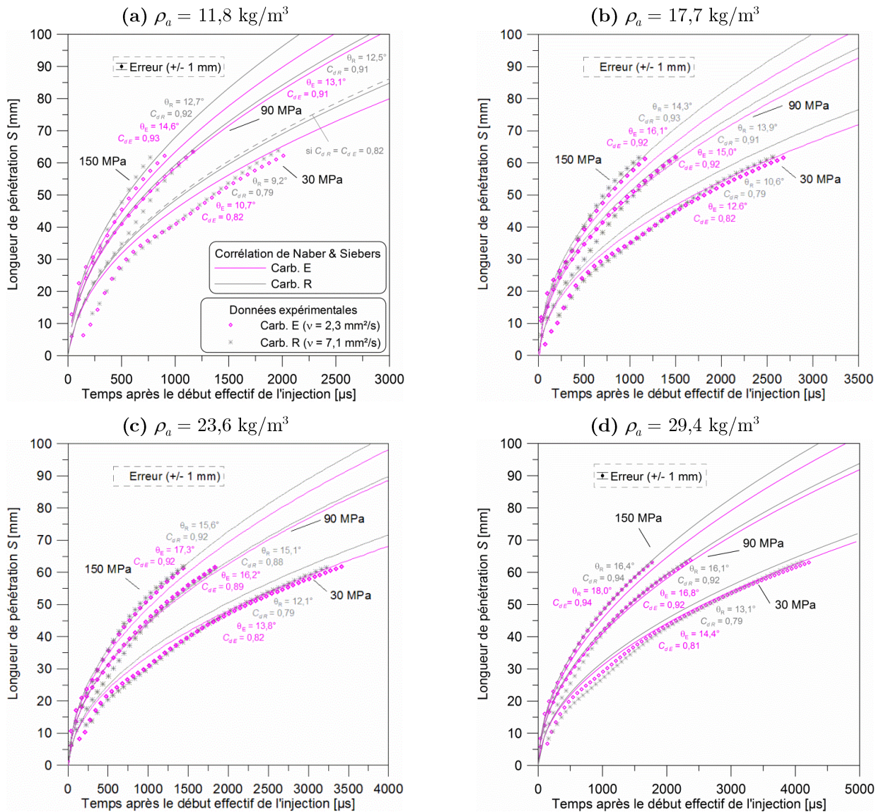
FIG. 4.13 : Valeurs expérimentales et estimées de l'évolution temporelle de la longueur de pénétration – Influence de la viscosité - P_i = 30 à 150 \text{ MPa} , \rho_a = 11,8 à 29,4 \text{ kg/m}^3 , T_a = 297 \text{ K} , t_i = 4000 \mu\text{s}
