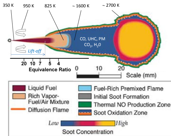
FIG. 1.33 : Schéma du modèle conceptuel de la combustion Diesel contrôlée par le mélange avant la fin de l'injection [Dec, 1997] étendu par Flynn et al. (1999)
