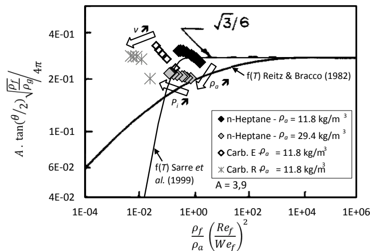
FIG. 4.5 : Dépendance théorique de l'angle du spray en fonction des conditions de fonctionnement [Reitz & Bracco, 1982]
