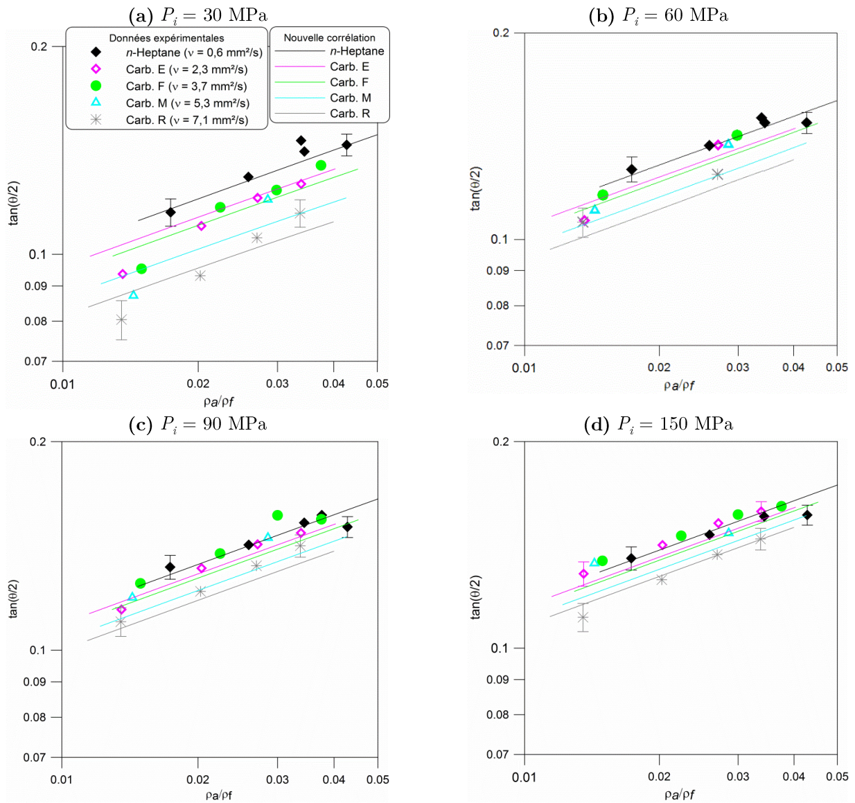
FIG. 4.3 : Valeurs expérimentales et estimées de la tangente de l'angle du demi-spray en fonction du rapport des densités air/carburant - Influence de la viscosité - P_i = 30, 60, 90 et 150 MPa
