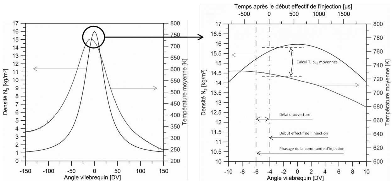
FIG. 6.1 : Évolution de la densité et de la température dans le cylindre à partir du relevé de pression cylindre – P col = 1,1 bar
