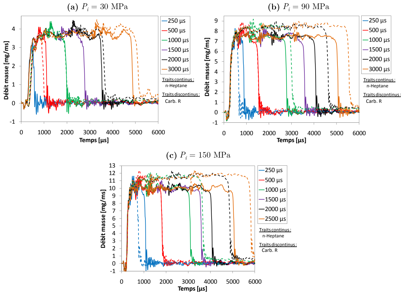
FIG.-A IV-I : Taux d'introduction pour différentes pressions d'injection et différents temps de commande - Carburants : n -Heptane et carb. « R »
