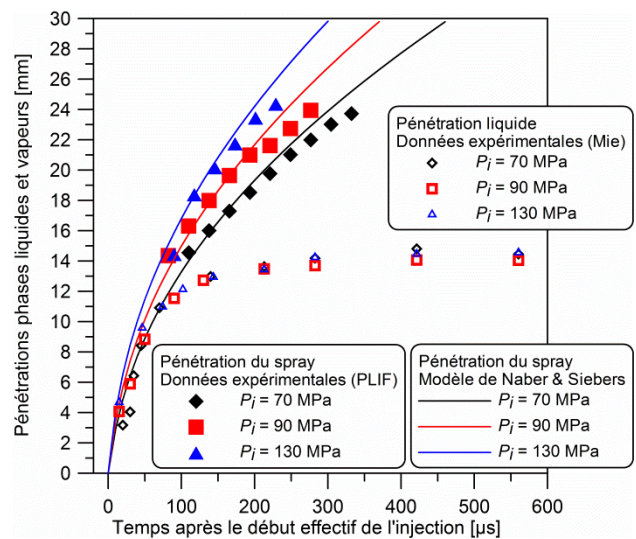
FIG. 6.14 : Pénétrations des phases liquide et vapeur pour trois pressions d'injection – Carb. « A » – \rho_{N_2} = 15,8 kg/m 3 – T_{N_2} = 721 K
