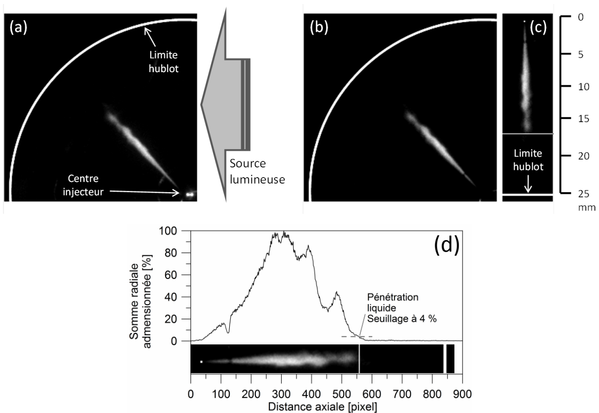
FIG. 2.26 : Etapes du traitement des images de diffusion de Mie. (a) Image brute ; (b) Bruit de fond soustrait ; (c) Image pivotée ; (d) Détermination de la longueur liquide à partir du profil longitudinal.
