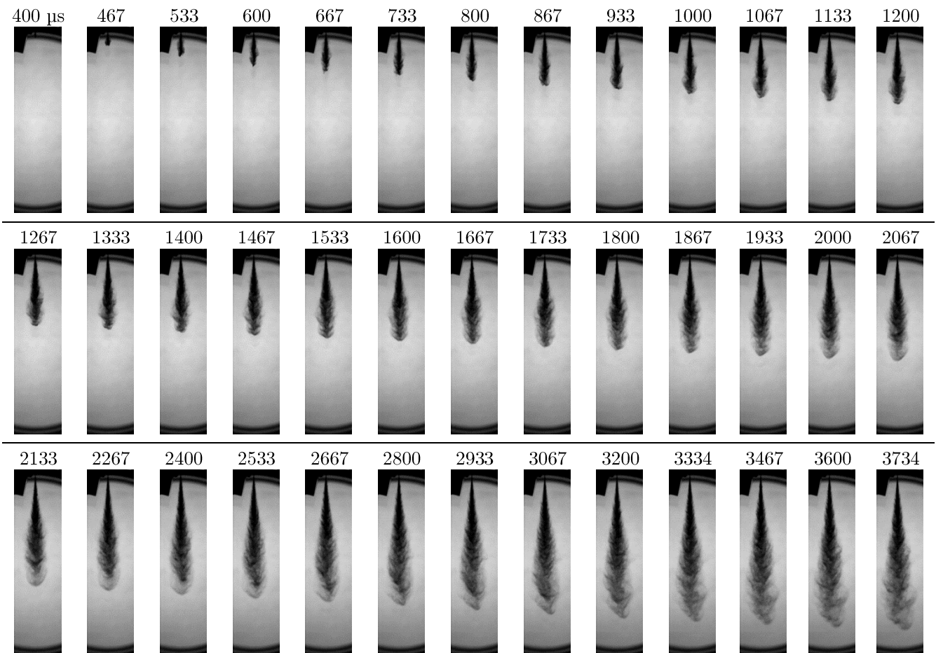
FIG. 2.6 : Exemple d'évolution du spray – n -Heptane – P_i = 30,0 \text{ MPa} – \rho_a = 11,8 \text{ kg/m}^3
