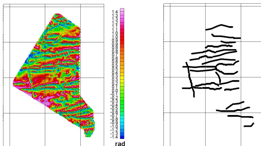
Figure 6.36 : Carte du tilt angle (à gauche) et son analyse structurale (à droite), AREVA09 Mikouloungou Kiéné Nord.
