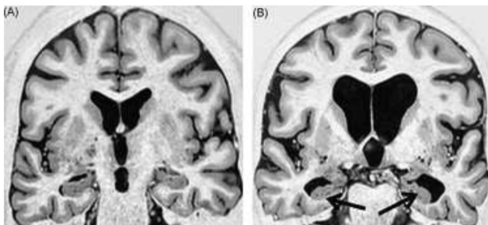
Figure 1 - Pariante et al. (2009), IRM cérébrales obtenues à l'aide de séquences TIR en coupes coronales.
