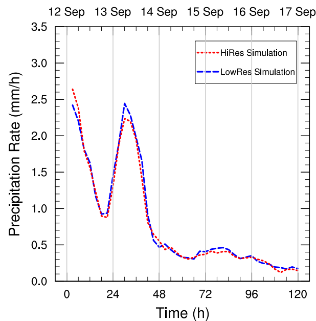
FIG. 4.5: Evolution temporelle du taux de précipitations à partir du 12 septembre 2006 à 0 h UTC, moyenné dans un rayon de 400 km autour de la position de Florence, dans les simulations Méso-NH HiRes et LowRes.
