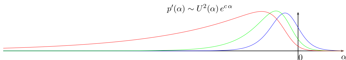
FIGURE 10 – Comportement de p'(\alpha) pour différentes valeurs du seuil de l'effet Allee \rho : en bleu \rho = 0.1 , en vert \rho = 0.3 et en rouge \rho = 0.45 .
