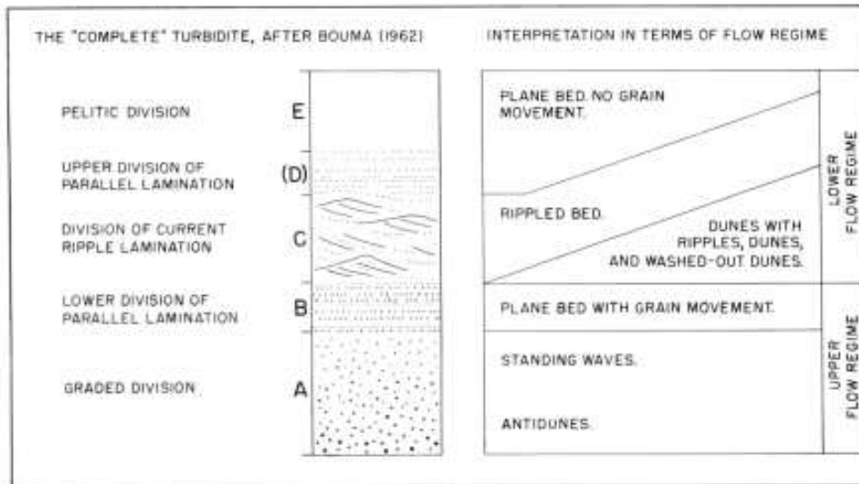
Figure 1.7 : interprétation de la séquence de Bouma en terme de régime hydraulique par Walker (1967).
