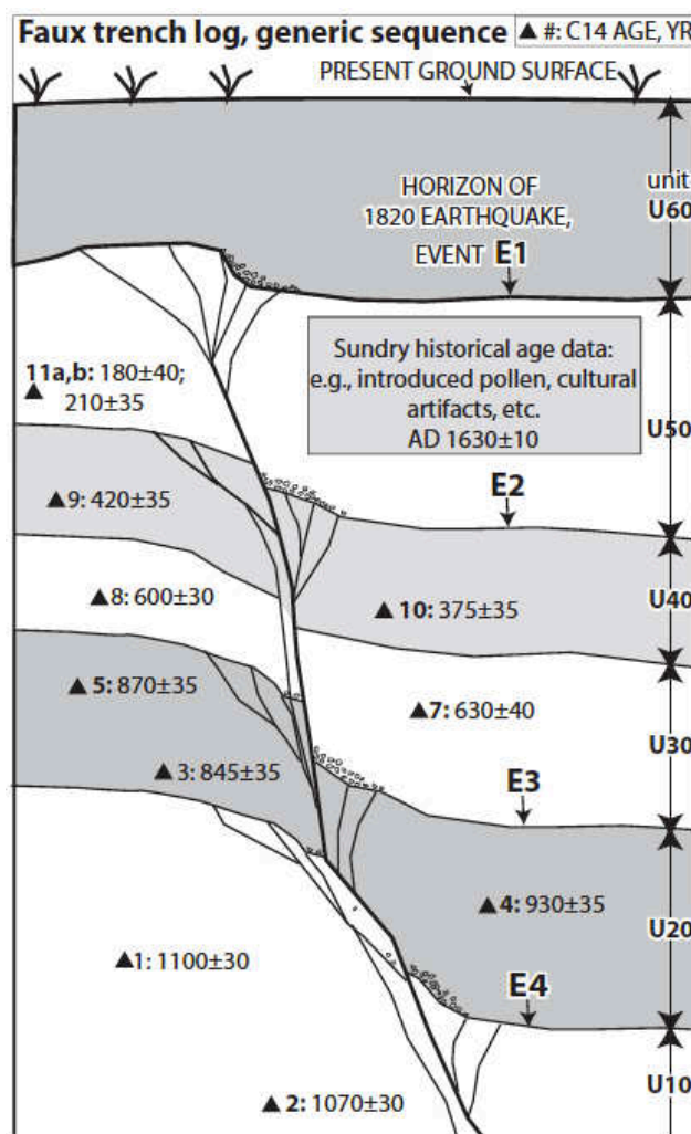
Figure 1.32 : modèle d'une tranchée de faille (Lienkaemper and Bronk Ramsey, 2009). Les niveaux en gris sont des paléosols traversés lors des paléo-séismes. La datation du séisme se fait par datation des différents horizons E.
