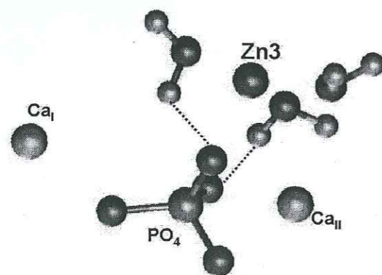
Figure 6.2 : Représentation d'un ion zinc, proche du groupe phosphate, entouré de sa première sphère d'hydratation. Les lignes en pointillé représentent des liaisons d'hydrogène.
