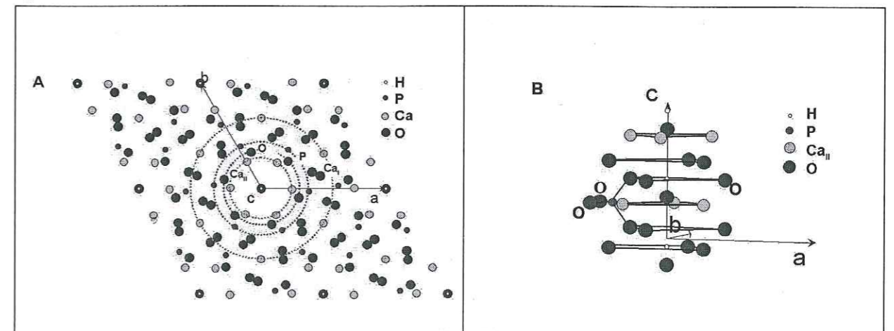
Figure 4.2 : (a) Vue de la structure de l'hydroxylapatite dans le plan (001). (b) Vue de la structure de l'environnement de l'axe z.
