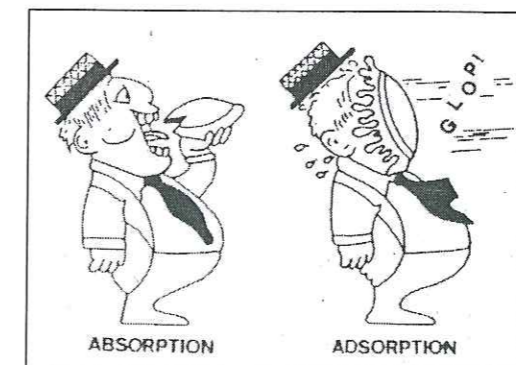
Figure 4.9 : Différence entre adsorption et absorption (LAGUÈS, 1990)
