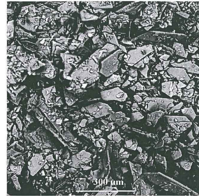
Figure 5.11 : Image MEB de la poudre hydroxylapatite BioRad.
