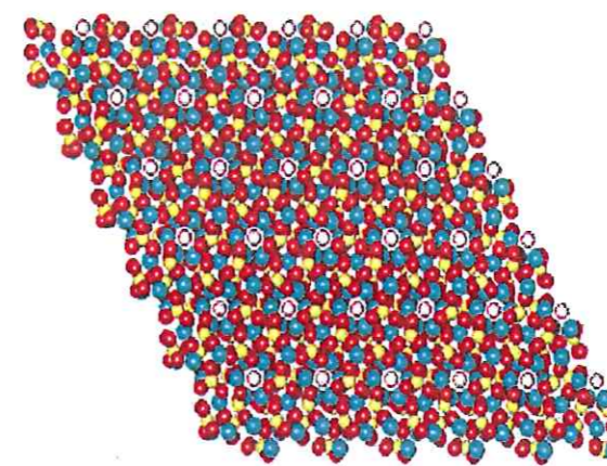
Figure 5.1 : L'hydroxylapatite est construite avec 36 cellules unitaires. En rouge les atomes d'oxygène, en bleu les atomes de calcium, en jaune les atomes de phosphore et blanc les hydroxydes.
