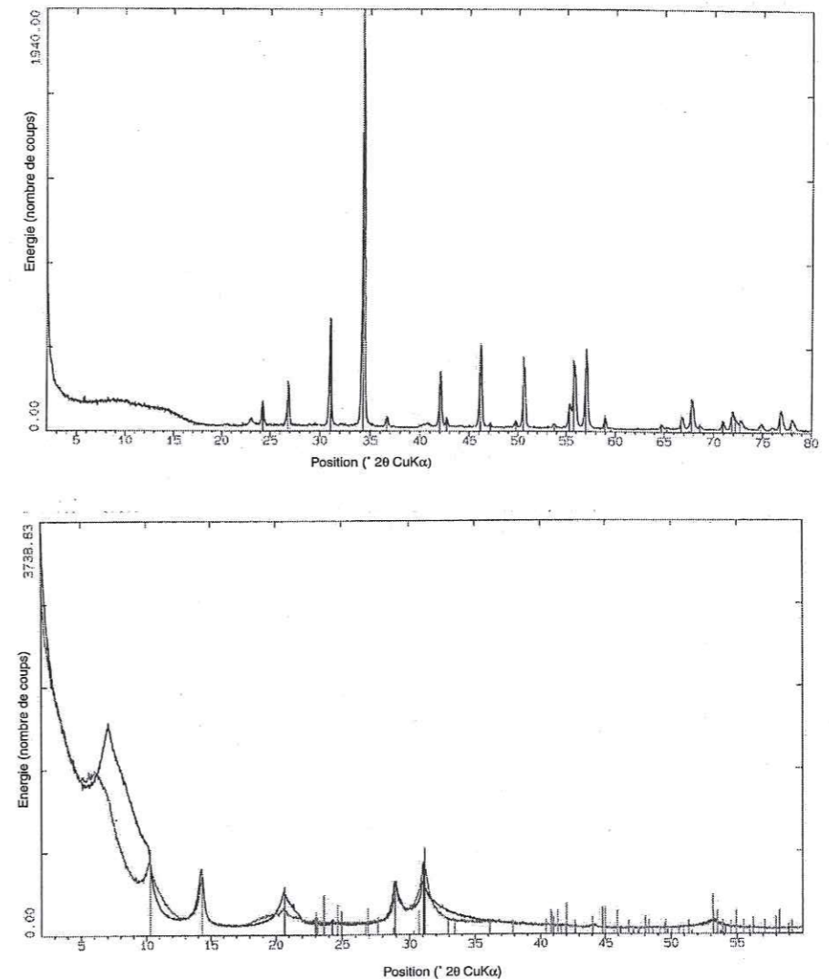
Figure 5.18 : Spectres de diffraction de rayons X des sédiments du fond du lac. (a) la fraction totale : spectres dominés par ceux de la calcite et du quartz. (b) la fraction fine < 2 μm : pics supplémentaires correspondant à la muscovite, la kaolinite et à des interstratifiés smectite/illite.
