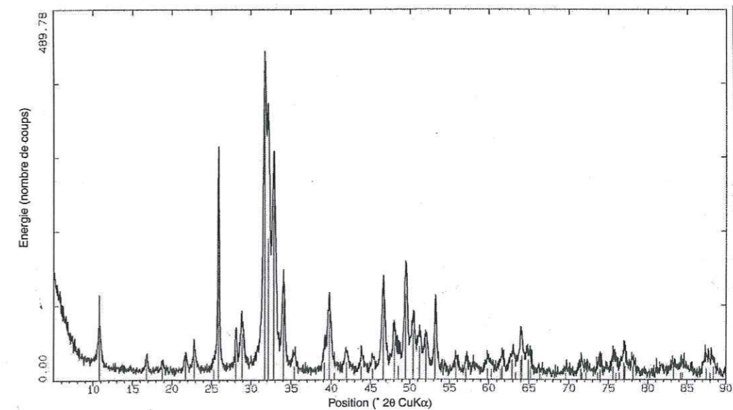
Figure 5.12 : Spectre de l'HAP Bio-Rad par DRX.
