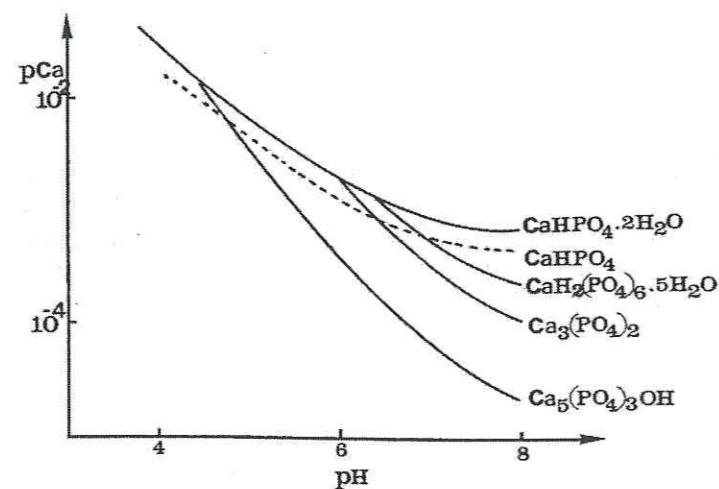
Figure 4.14 : Isothermes de solubilité à 25°C de phosphates calciques dans le système Ca(OH)_2-H_3PO_4-H_2O , avec une constante de solubilité pour l'hydroxylapatite de 4.7 \cdot 10^{-59} d'après (THIRIOUX, 1990)
