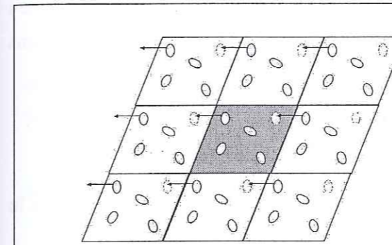
Figure 5.6 : Déplacement des molécules dans un système périodique à deux dimensions (ALLEN and TILDESLEY, 1987)
