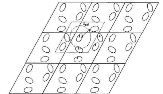
Figure 5.7 : Un potentiel tronqué agissant sur une molécule dans un système périodique à deux dimensions d'après (ALLEN and TILDESLEY, 1987)
