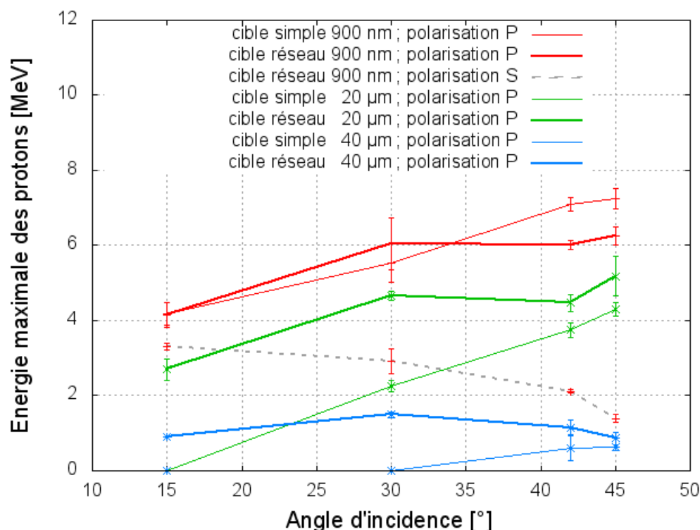
FIGURE 5.17 – Energie maximale des protons accélérés lors de l’interaction avec des cibles réseaux en fonction de l’angle d’incidence, en polarisation S et P et pour des cibles de 900 nm, 20μm et 40μm d’épaisseur. Pour ces deux dernières épaisseurs, les énergies des protons en polarisation S n’ont jamais dépassé le seuil de détection.
