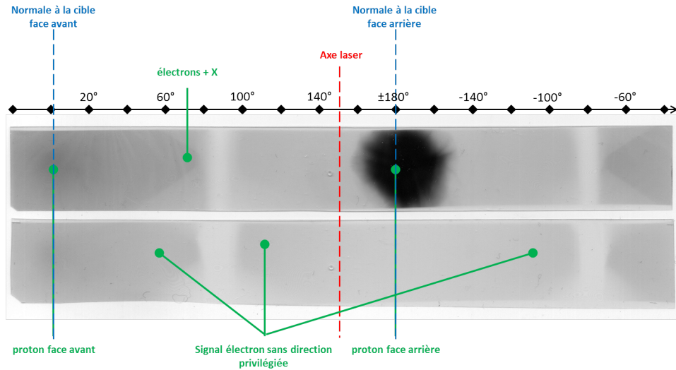
FIGURE 5.18 – Signal obtenu en régime Bas Contraste sur une pile de deux films radiochromiques protégés par un filtre de 2\ \mu\text{m} de Mylar aluminisé, disposées en couronne à 3 cm de l’interaction du laser incident à 30^\circ sur une cible réseau de 20\ \mu\text{m} d’épaisseur (réseau de 500\ \text{nm} de profondeur et de pas 2\lambda )
