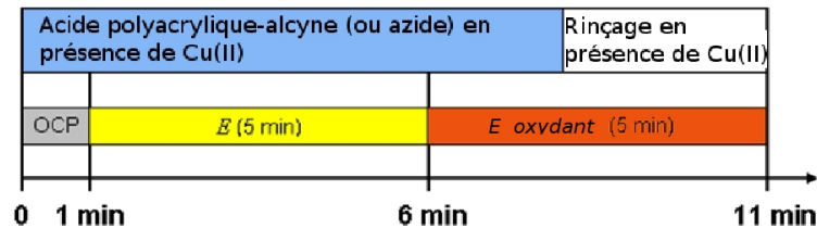
FIGURE 3.2 – Protocole de construction d'une multicouche de polymères réticulée par chimie click électrocontrôlée.
