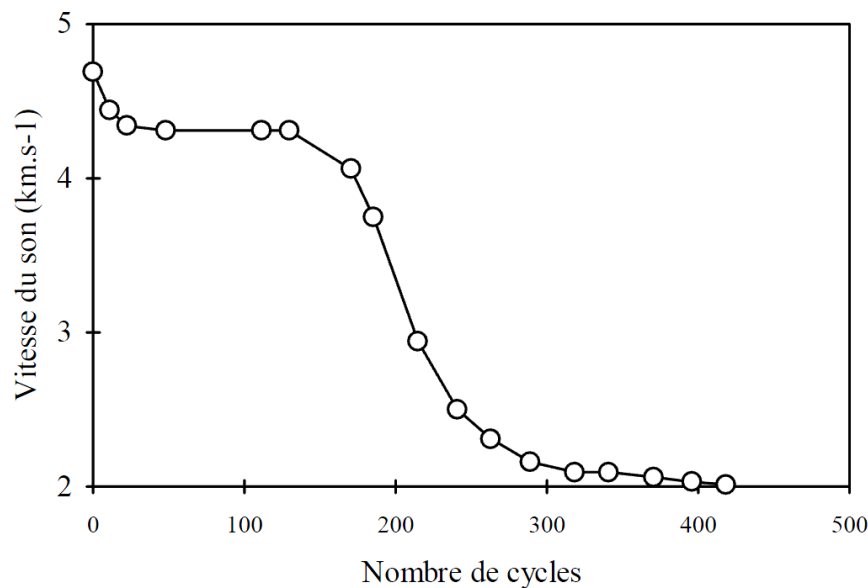
Figure IV. 34 : Dégradation progressive d'un béton par des cycles de gel/dégel (norme ASTM-C-666, procédure B) [CAR92]
