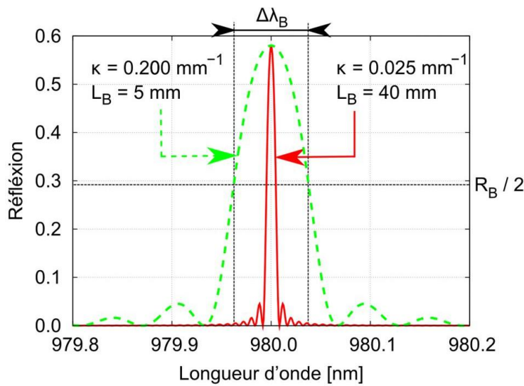
figure 4-19 : Spectre de réflexion de deux réseaux de Bragg possédant un produit \kappa \times L_B = 1 .
