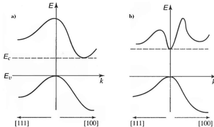
figure 2-2 : Diagramme de bande pour les axes cristallographiques [111] et [100] pour a) le silicium et b) l'arséniure de gallium, d'après [70].
