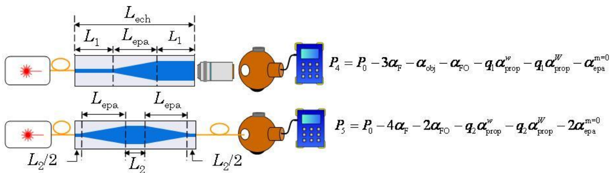
figure 3-31 : Bancs de caractérisation pour mesurer les pertes occasionnées par l'épanouisseur.
