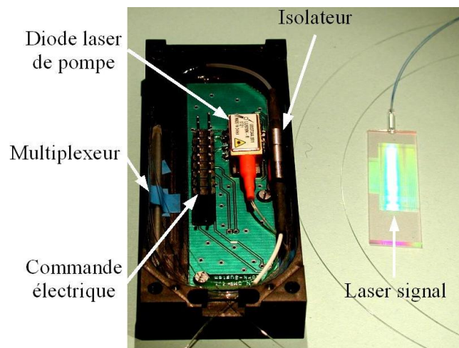
figure 1-11 : Injecteur optique et son environnement développé dans le cadre du projet européen NESLIE.
