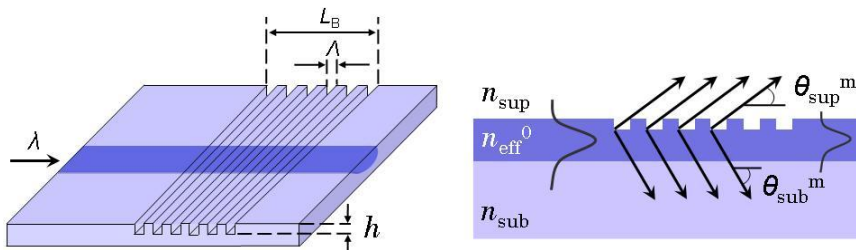
figure 4-12 : Schéma d'un guide d'onde de Bragg et principe du découplage d'un mode guidé.
