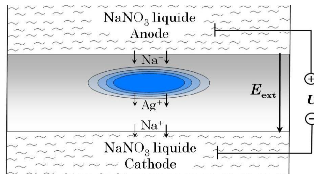
figure 3-7 : Principe de l'enterrage d'un guide d'onde.
