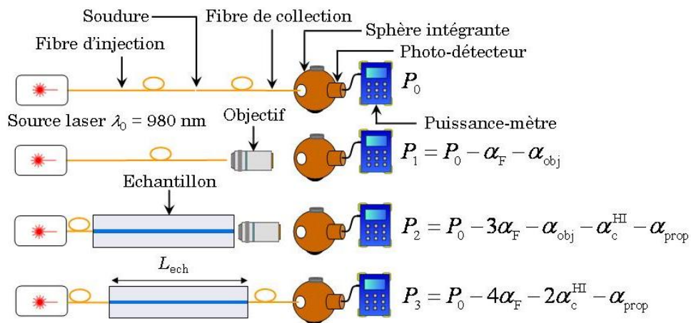
figure 3-22 : Méthode des quatre mesures permettant de caractériser les pertes d'un guide d'onde.
