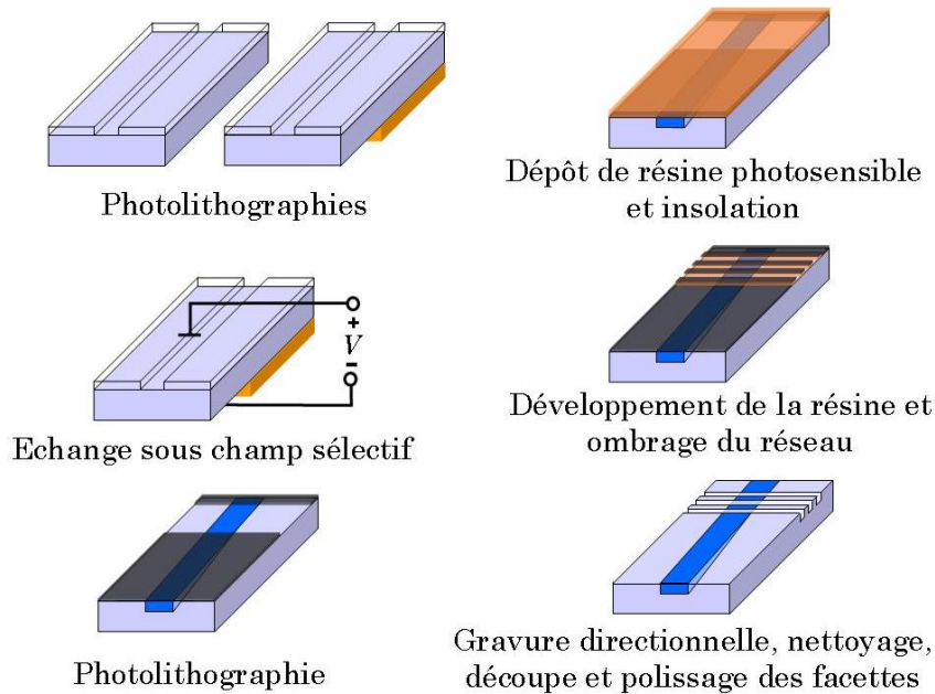
figure 4-22 : Etapes de fabrication du guide d'onde de Bragg.
