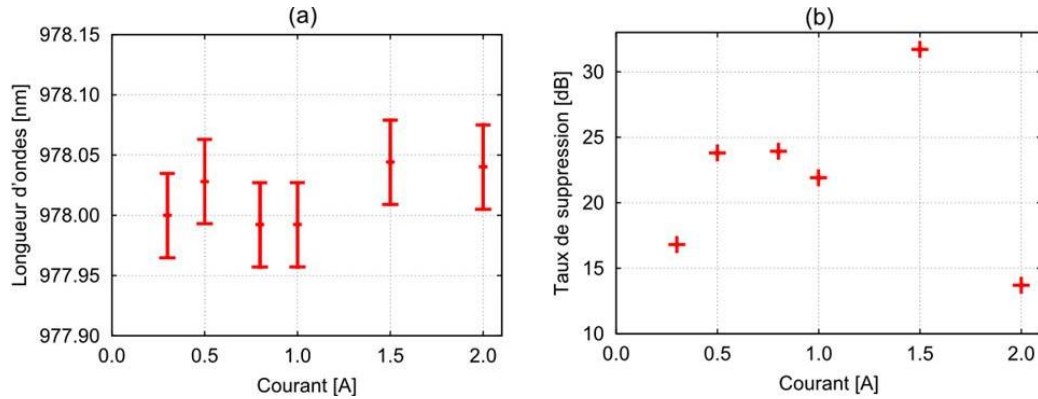
figure 4-29 : Evolutions de la longueur d'onde du pic d'émission (a) et du taux de suppression du mode secondaire (b) en fonction du courant.
