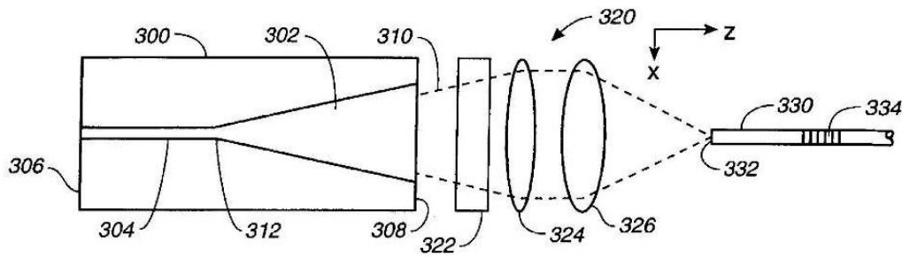
figure 1-21 : Diode laser à épanouisseur stabilisée par une fibre de Bragg placée du côté large. Le champ de la diode laser est adapté est celui supporté par la fibre grâce à des optiques de volume, d'après [48].
