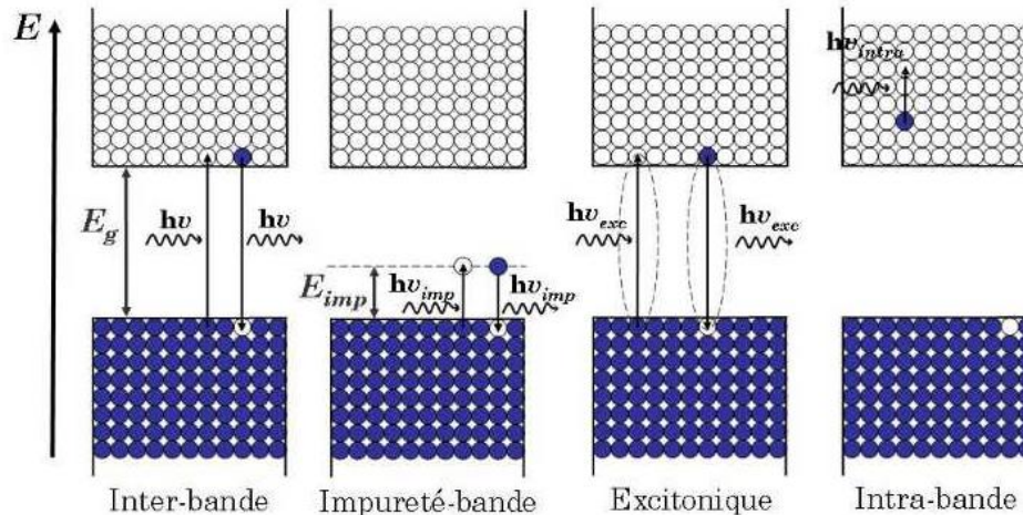
figure 2-4 : Illustration des mécanismes d'absorption et d'émission dans les semi-conducteurs.
