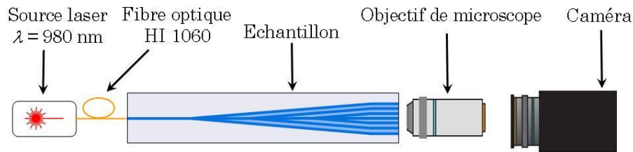
figure 4-5 : Banc de mesure du champ proche du guide d'onde d'entrée du convertisseur.
