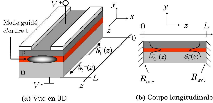
figure 2-11 : Schéma d'une diode laser Fabry-Perot.
