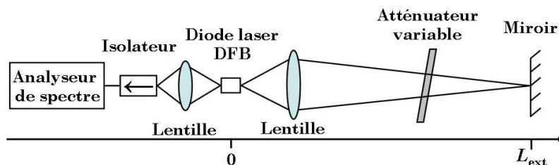
figure 2-16 : Schéma du montage expérimental permettant d'étudier l'effet de la rétroaction sur une diode laser.
