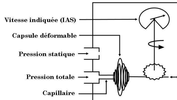
figure 1-2 : Structure minimale d'un indicateur de vitesse, souvent appelé « Badin » en référence au nom de son inventeur.
