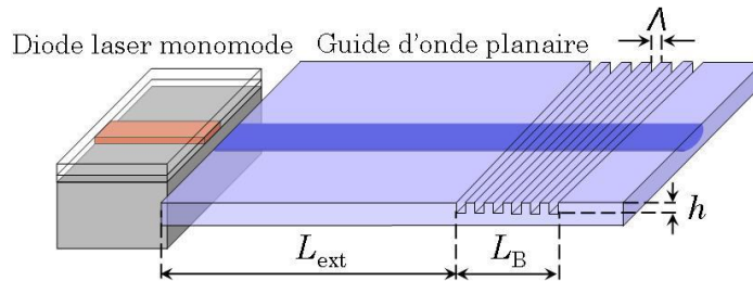
figure 2-22 : Schéma d'une diode laser monomode dont le champ en sortie est couplé dans un guide d'onde planaire monomode sur lequel est inscrit un réseau de Bragg en surface supérieure.
