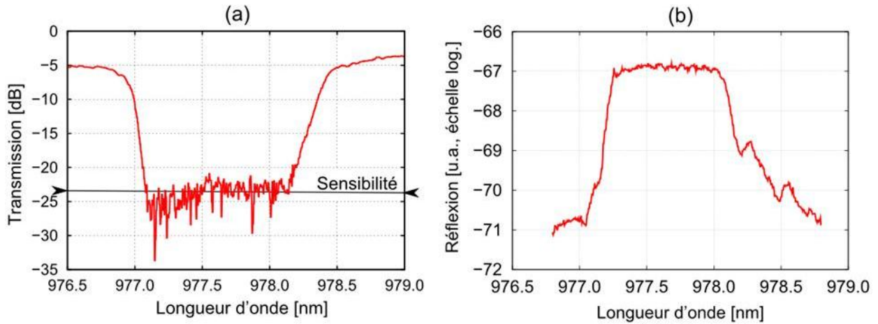
figure 4-24 : Courbes de transmission et de réflexion du guide d'onde de Bragg de largeur w = 2 \mu\text{m} .
