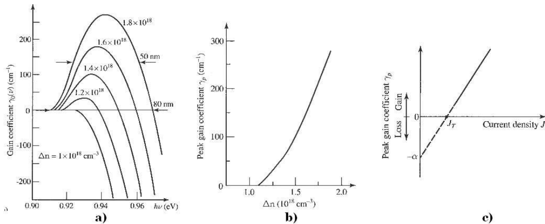
figure 2-8 : Evolutions à T = 300 \text{ K} pour l'alliage InGaAsP du coefficient de gain \gamma en fonction de l'énergie h\nu pour plusieurs concentrations de porteurs injectés (a), du pic de gain \gamma_p en fonction de l'injection (b) et linéarisation de la relation entre le pic de gain et la densité de courant (c). D'après [76].
