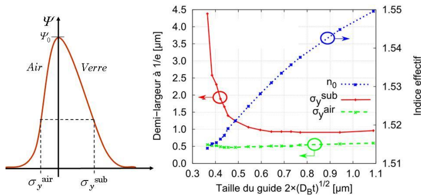
figure 3-13 : Profil typique d'un mode guidé et évolutions de l'indice effectif ainsi que de la taille verticale du mode fondamental en fonction de la taille caractéristique du guide.
