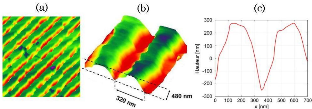
figure 4-18 : Image AFM de la surface du verre (a), zoom sur une période (b) et profil du réseau (c).
