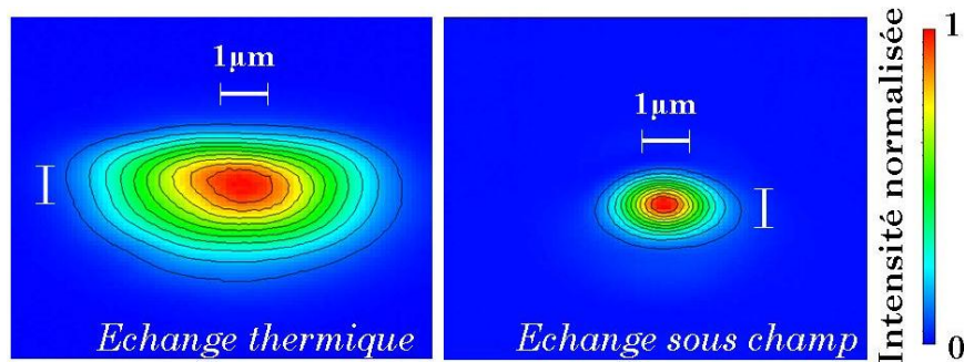
figure 3-25 : Champs proches d'un guide d'onde de largeur 2 \mu\text{m} . A gauche côté masqué, à droite côté échange sous champ.
