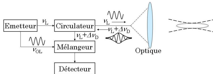
figure 1-7 : Principe optique de l'anémomètre laser à référence, tiré de [9]. Ce schéma décrit la version mono-statique, où les directions optiques aller et retour sont confondues.
