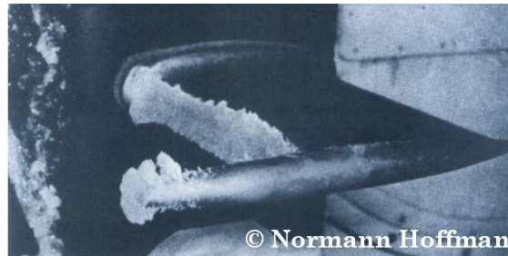
figure 1-4 : Photographie de l'entrée d'un tube de Pitot bouchée par de la glace lors d'un arrêt au sol. Photographie extraite de [5].
