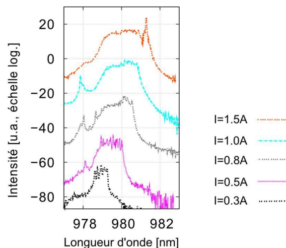
figure 4-1 : Spectre de la diode laser à ruban large pour cinq courants. Les courbes ont été décalées verticalement pour faciliter leur lecture.
