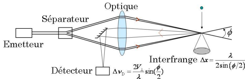
figure 1-6 : Principe de l'anémomètre à franges, d'après [8].
