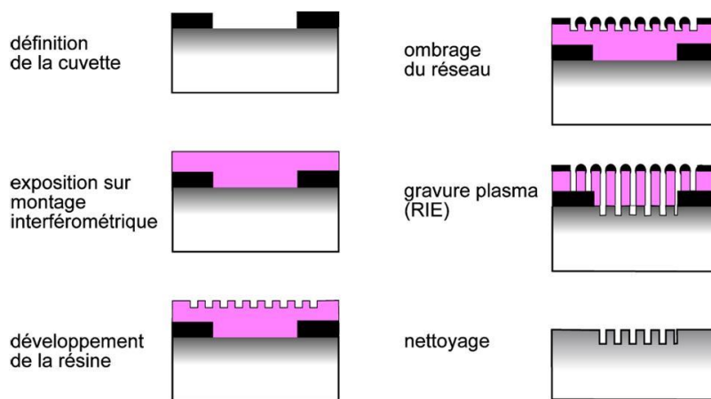
figure 4-13 : Etapes de fabrication d'un réseau de Bragg sur un substrat de verre, d'après [121].
