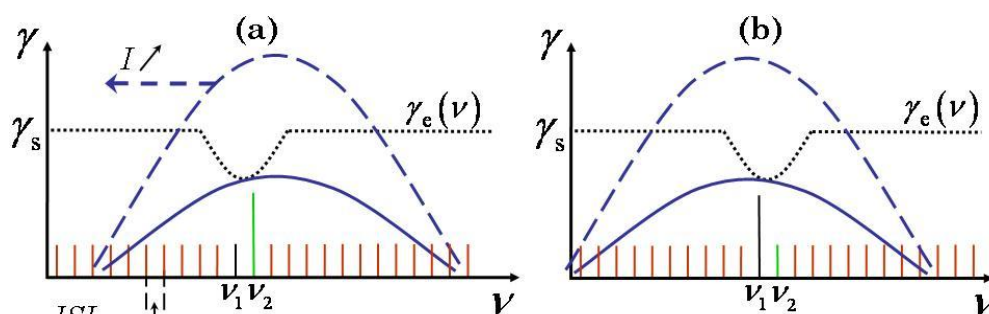
figure 4-9 : Fréquence d'émission de la cavité à faible courant (a) et à fort courant (b).
