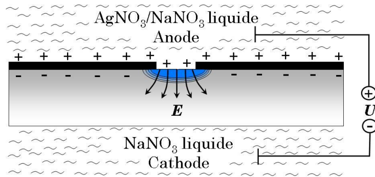
figure 3-9 : Principe de l'échange d'ions assisté par champ électrique ou échange sous champ.
