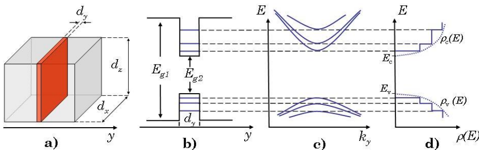
figure 2-9 : Structure à puits quantique a), sa distribution en énergie b), son diagramme de bandes c) et sa densité d'états d).
