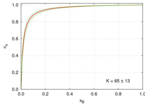
figure 3-4 : Concentration normalisée c_s à la surface du verre en fonction de la fraction molaire x_B des ions Argent présent dans un bain de nitrate de sodium et d'argent.
