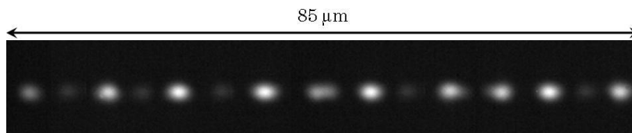
figure 4-6 : Intensité en sortie du guide d'onde d'entrée du convertisseur.
