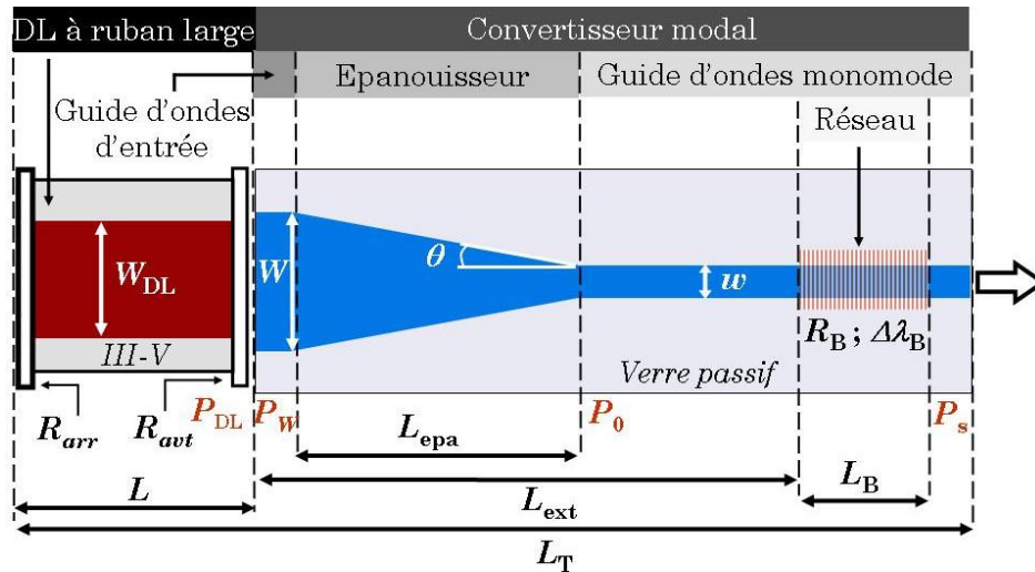
figure 2-25 : Vue du dessus du dispositif à réaliser.
