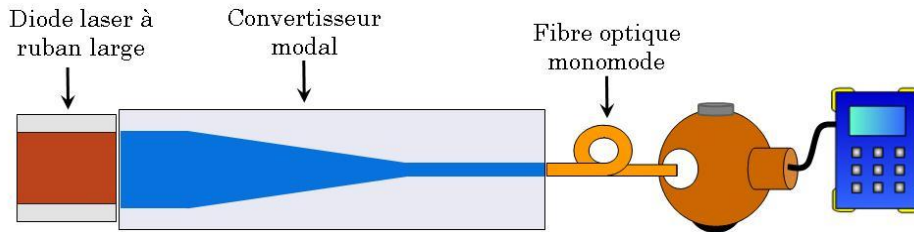
figure 3-32 : Banc de mesure des pertes d'insertion de l'épanouisseur
