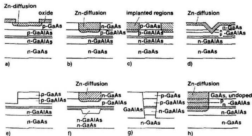
figure 1-16 : Quelques structures lasers faites en GaAs/ \text{Ga}_{1-x}\text{Al}_x\text{As} , d'après [21].
