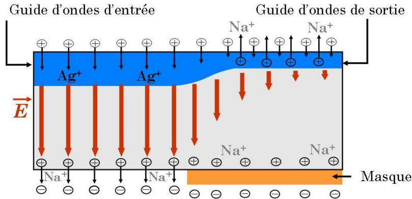
figure 3-14 : Principe de l'échange sous champ masqué.
