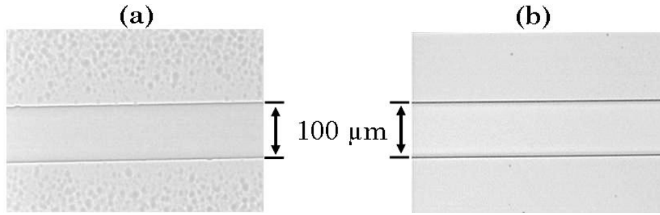
figure 3-24 : Etat du masque diélectrique après échange sous champ pour une épaisseur de 40 nm (a) et pour une épaisseur de 80 nm (b).
