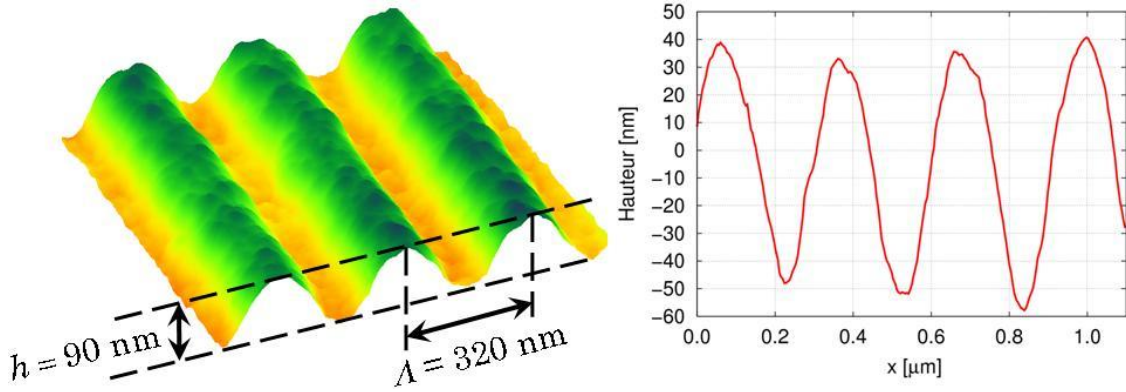
figure 4-15 : Image AFM du réseau inscrit dans la résine.
