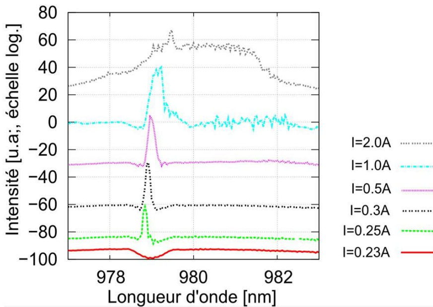
figure 4-8 : Spectres d'émission obtenus avec un convertisseur classique et une fibre à réseau de Bragg. Les courbes ont été décalées dans la direction verticale.
