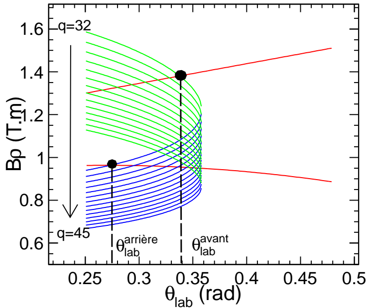
FIGURE 3.49 – Cinématique des différents états de charge du ^{122}\text{Sn} . L'état de charge le plus petit ( q=32 ) correspond aux valeurs de B\rho les plus grandes et l'état de charge le plus grand ( q=45 ) aux valeurs les plus petites. La partie verte représente les angles avant de la distribution et la bleue les angles arrière. Les traits rouges représentent les limites de l'acceptance que nous avons observées expérimentalement. Les points noirs représentent les angles avant et arrière déterminant les limites de l'acceptance pour l'ion ^{122}\text{Sn}^{32+} .
