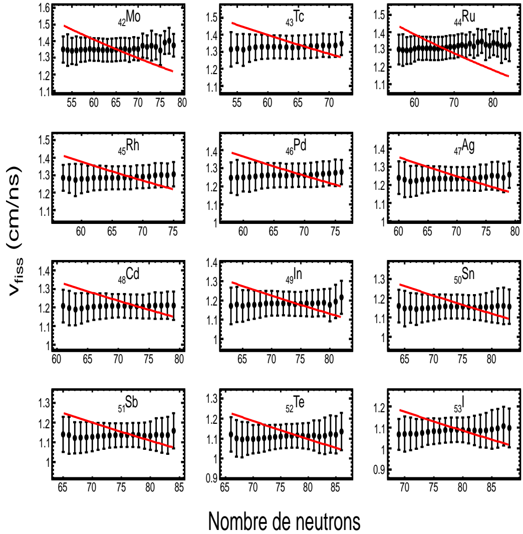
FIGURE 5.7 – Évolution de la vitesse d'un fragment de fission dans le référentiel du noyau fissionnant v_{\text{fiss}} en fonction du nombre de neutrons pour la fission du ^{250}\text{Cf} pour les éléments du _{42}\text{Mo} au _{53}\text{I} . Les barres d'erreurs correspondent à la largeur de la distribution en vitesse. La courbe rouge correspond à la relation 5.5 avec les paramètres r_0=1,16 fm, \beta_1=\beta_2=0,625 et d=2 fm.
