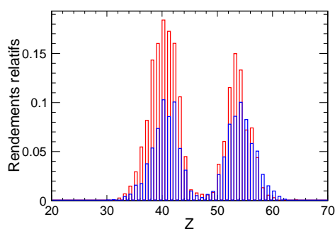
FIGURE 5.19 – Nombre de coups normalisés enregistrés pour les différents numéros atomiques Z des fragments de fission issus du ^{240, 241}\text{Pu} dans la partie gauche (en rouge) et droite (bleu) du télescope SPIDER.
