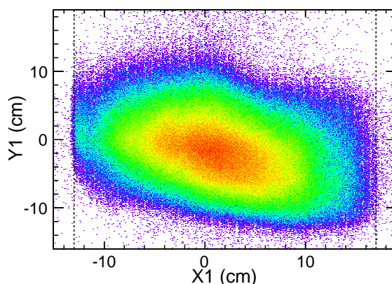
FIGURE 4.4 – Répartition des impacts des fragments de fission sur la Galette31. Les deux traits en pointillé représentent les limites physiques du détecteur.
