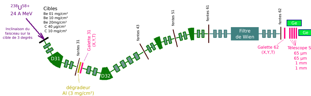
FIGURE 4.1 – Dispositif expérimental de l'expérience e547.
