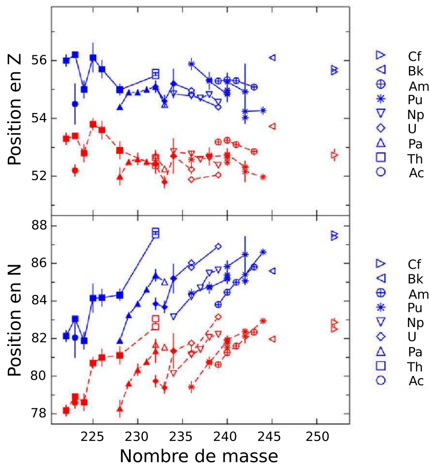
FIGURE 5.30 – Positions moyennes des différents modes de fission standard en fonction du nombre de proton (en haut) et de neutron (en bas) pour différents systèmes fissionnants. Le mode standard I est présenté en traits pleins bleus et le mode standard II en traits pointillés rouges. Issu de [Böckstiegel et al., 2008].
