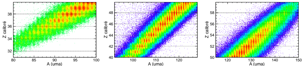
FIGURE 3.19 – Évolution de la charge Z en fonction de la masse expérimentale A pour l'ensemble de l'expérience (runs 295 à 412) soit environ 16 millions d'événements pour différentes régions.
