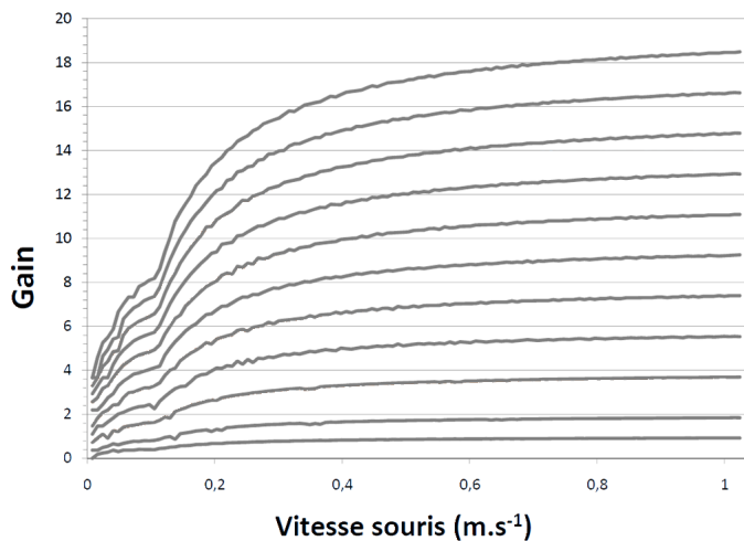
FIGURE 2.10 – Courbes d'accélération Windows XP dans l'espace vitesse/gain.
