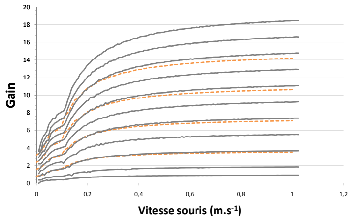
FIGURE 2.12 – Courbes d'accélération Windows XP (en gris) comparées aux courbes trouvées par Casiez ([CVBC08] - en orange pointillé)
