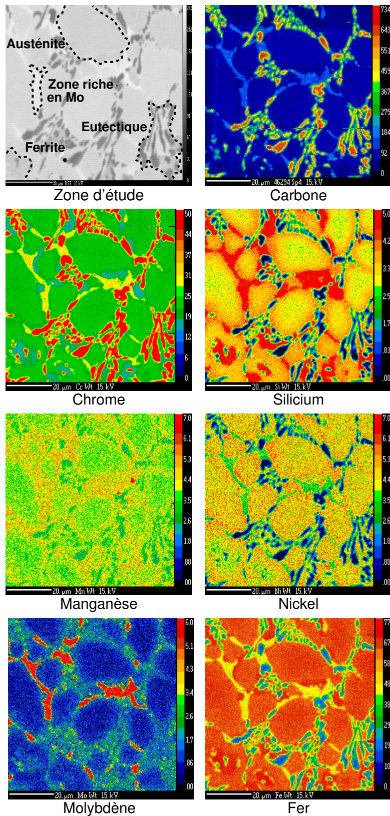
FIGURE 2.7: Norem02 brut de dépôt : cartographie de répartition des éléments chimiques.
