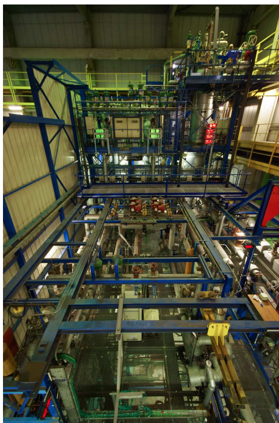
FIGURE 1: Boucle d'essai Cypres-Cythere
