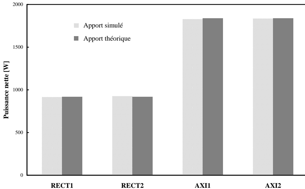
FIGURE 4.8: Comparaison pour chaque configuration de la puissance nette apportée en théorie et dans les cas modélisés.
