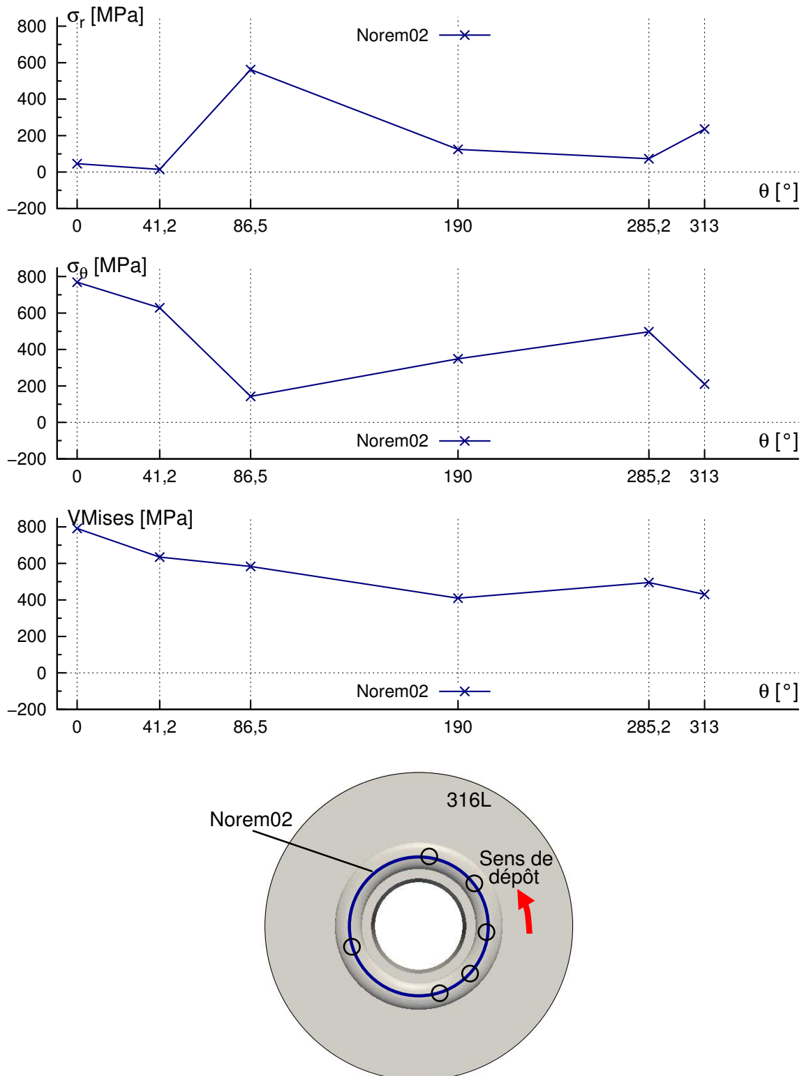
FIGURE 3.23: Cas AXI2 - Évolution de la contrainte radiale \sigma_r , circonférentielle \sigma_\theta et de la contrainte équivalente de von Mises dans le cordon de Norem02 déposé.
