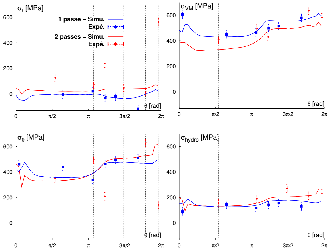
FIGURE 5.19: Comparaison des contraintes équivalentes de von Mises \sigma_{VM} , des contraintes circonférentielles \sigma_{\theta} et des pressions hydrostatiques \sigma_{hydro} en fonction de l'azimut mesurées expérimentalement et calculées dans le cordon de Norem02 entre les cas AXI1 et AXI2.
