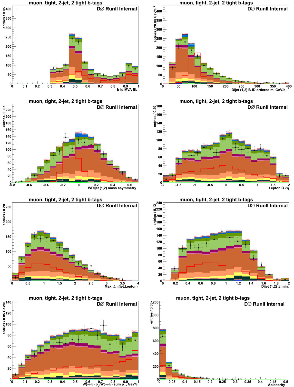
FIGURE V.13 – Histogrammes comparant les données (points) et la prédiction de la simulation (couleurs) pour les variables d’entrée du discriminant final de l’analyse, dans le canal 2 jets muon 2 tag tight. Le code de couleurs est visible sur la figure V.10.
